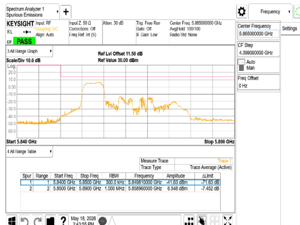
802.11ax_20MHz_Chain0_5865MHz_RU106_53
