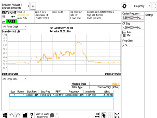
802.11ax_20MHz_Chain0_5885MHz_RU52_40
