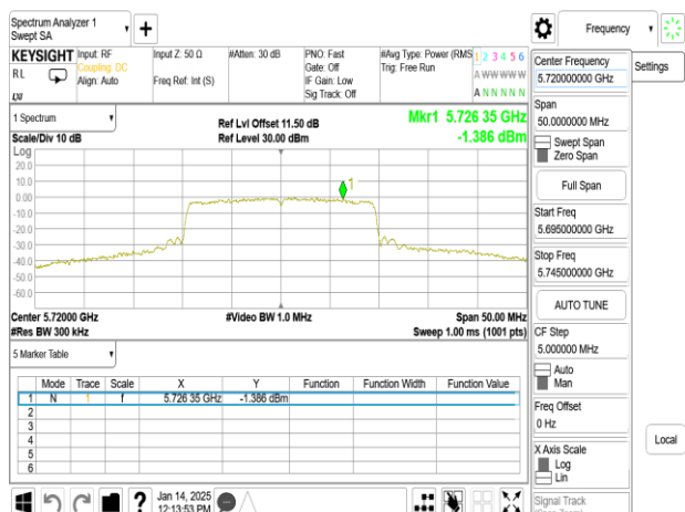
802.11ax_20MHz_Chain0_5720MHz_UNII 3
