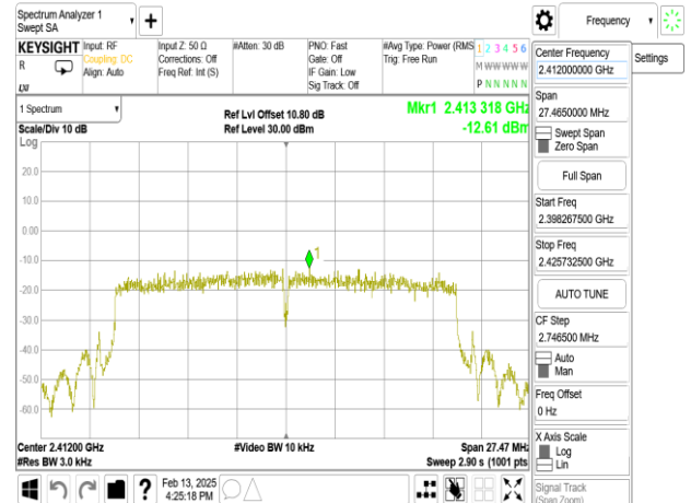
802.11ax_20MHz_Chain0_2412MHz_RU26_0
