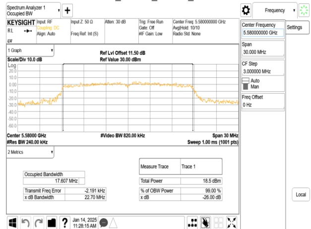
802.11n_20MHz_Chain0_5580MHz
