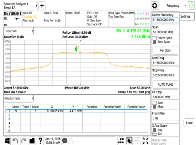
802.11ax_20MHz_Chain0_5180MHz_RU26_0
