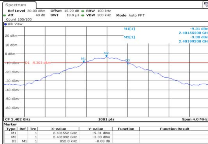
BLE BT5.0 Ant1 2402
