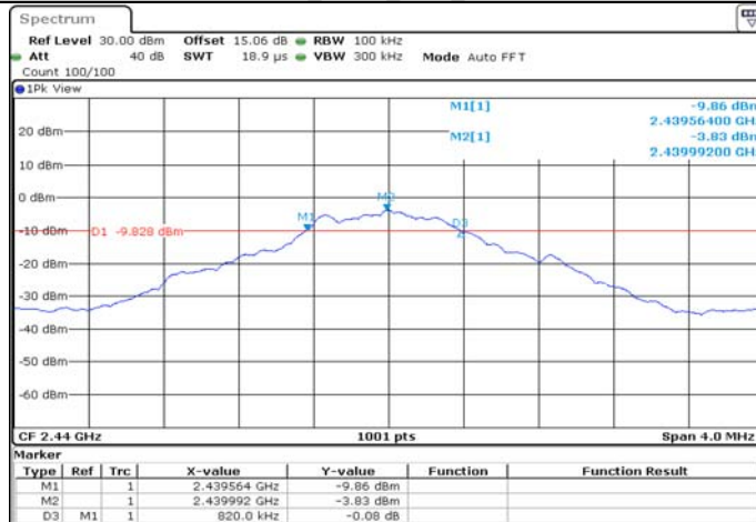
BLE BT5.0 Ant1 2440
