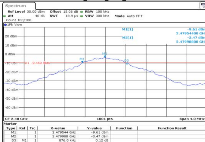
BLE BT5.0 Ant1 2480
