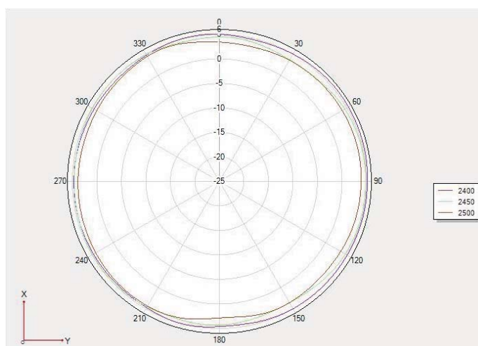
Theta 90 2D 图
