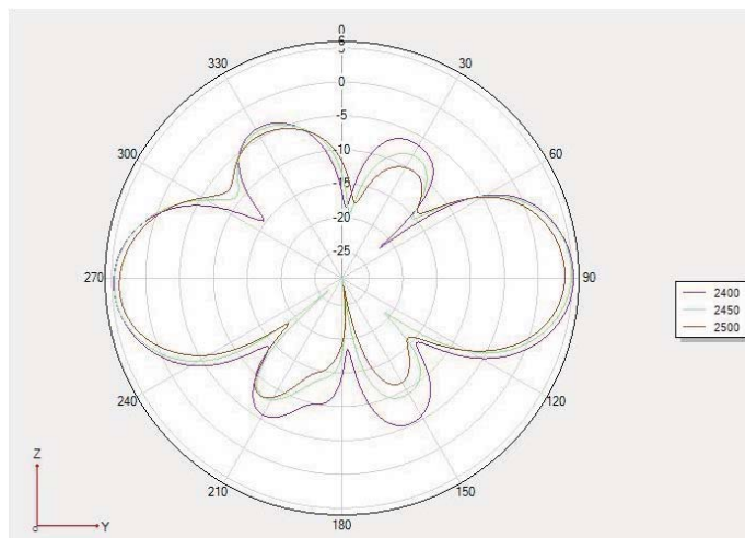
Phi 90 2D 图
