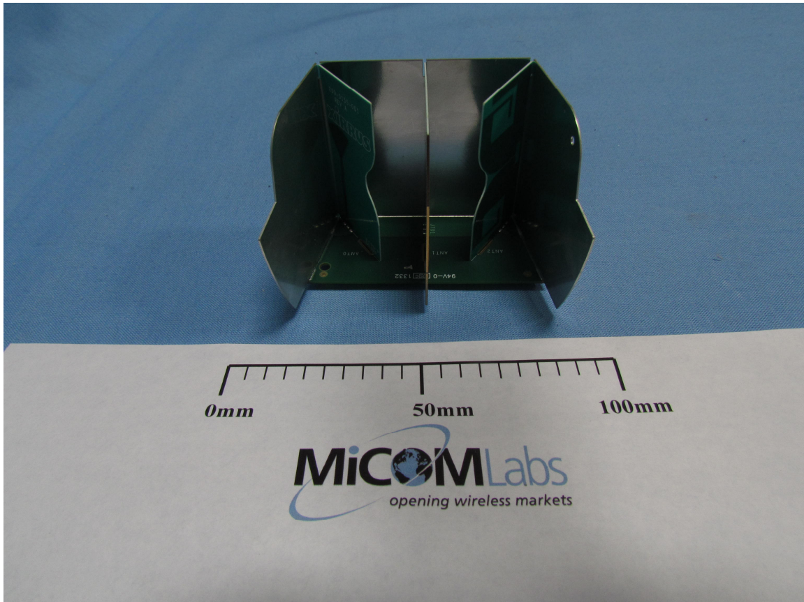
EUT bottom
