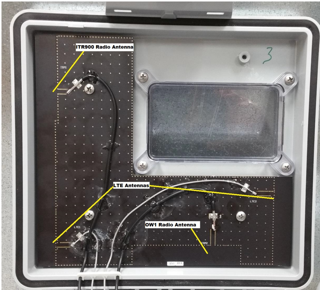
SBR ANTENNA ARRAY
