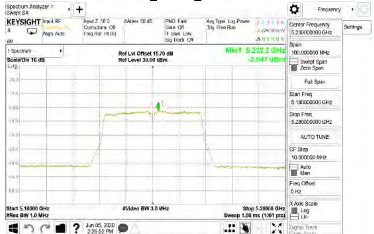
802.11n_40MHz_5230MHz
