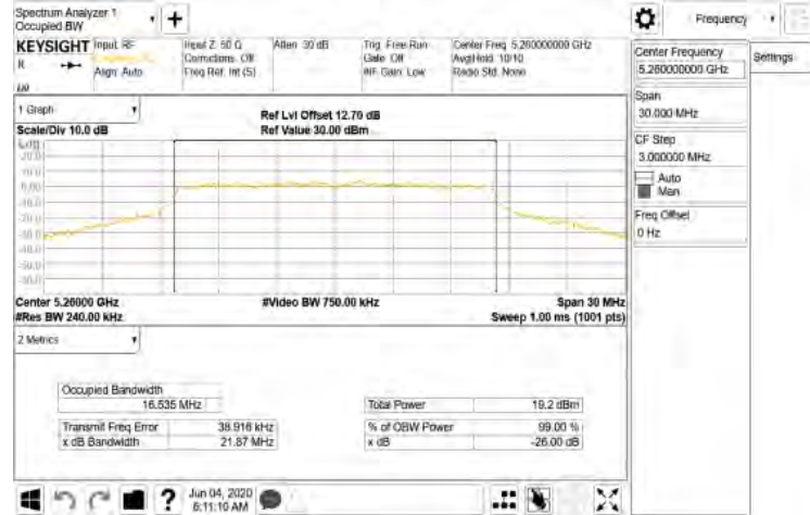
FCC_802.11a_20MHz_Chain0_5260MHz
