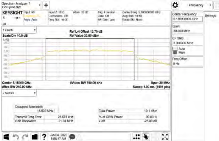
FCC_802.11a_20MHz_Chain0_5180MHz
