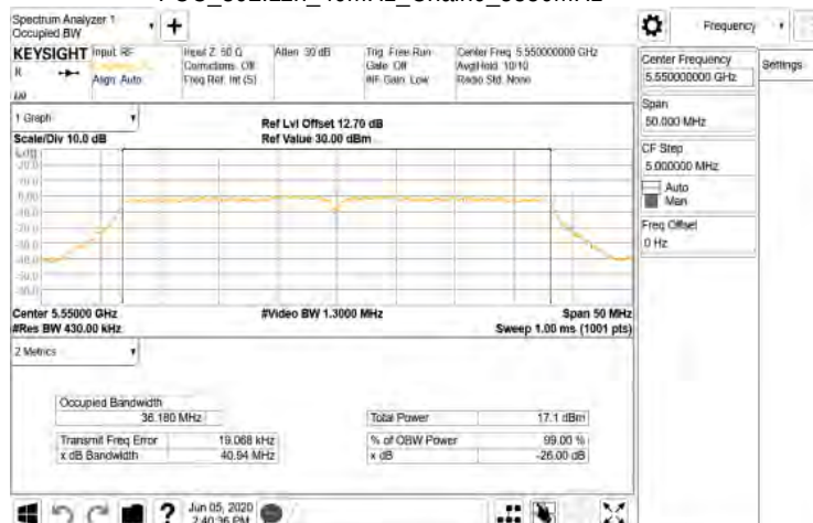
FCC_802.11n_40MHz_Chain0_5550MHz
