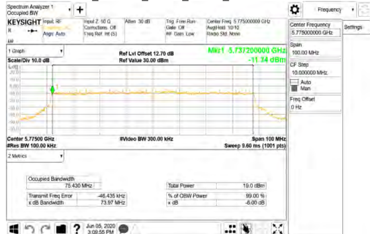
FCC_802.11ac_80MHz_Chain0_5775MHz
