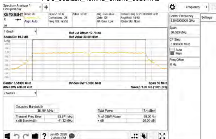
FCC_802.11n_40MHz_Chain0_5510MHz
