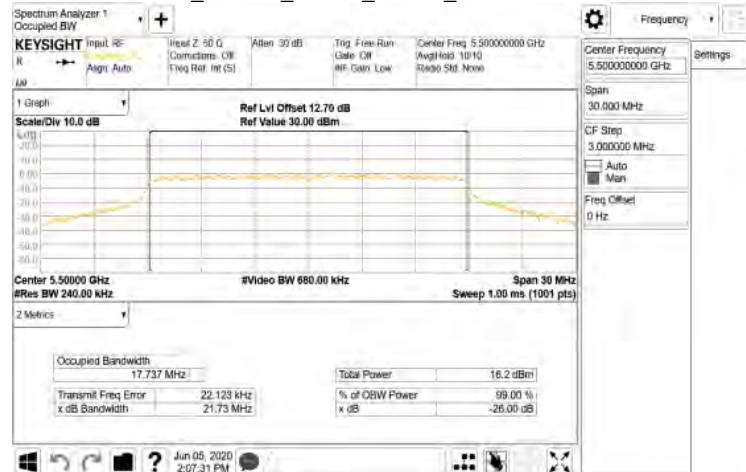
FCC_802.11n_20MHz_Chain1_5500MHz
