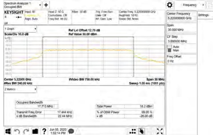
FCC_802.11n_20MHz_Chain1_5220MHz
