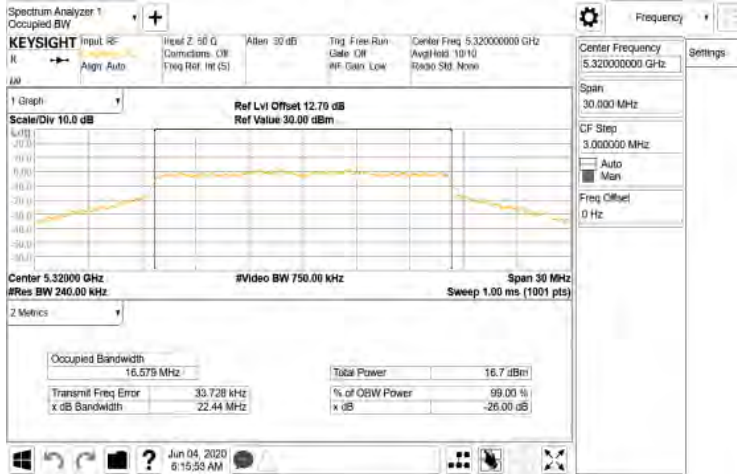
FCC_802.11a_20MHz_Chain1_5320MHz
