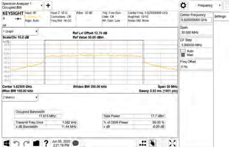
FCC_802.11n_20MHz_Chain0_5825MHz
