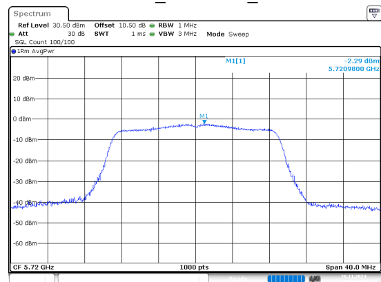
802.11n20_5720MHz_Chain 1
