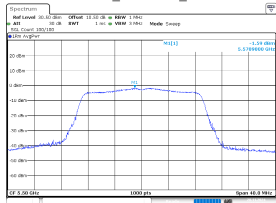
802.11n20_5580MHz_Chain 1
