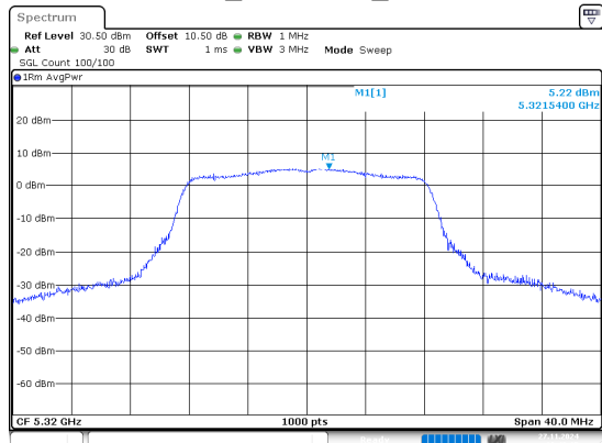
802.11a_5320MHz_Chain 0
