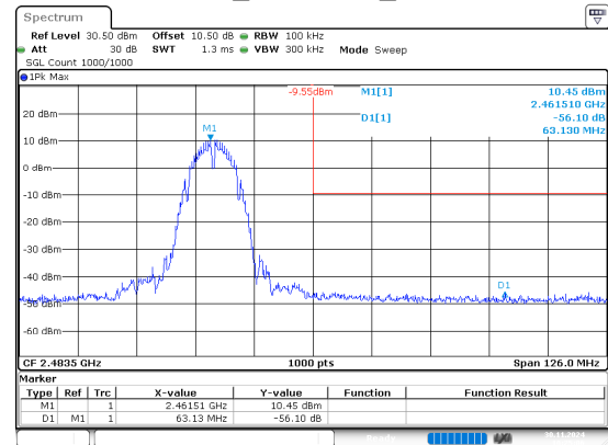
802.11b_2462MHz_Chain 0
