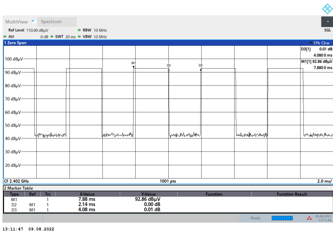
BLE (1Mbps)
