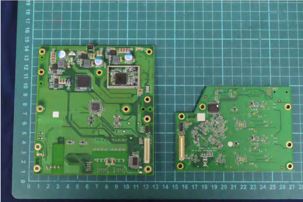
(16) EUT Photo
