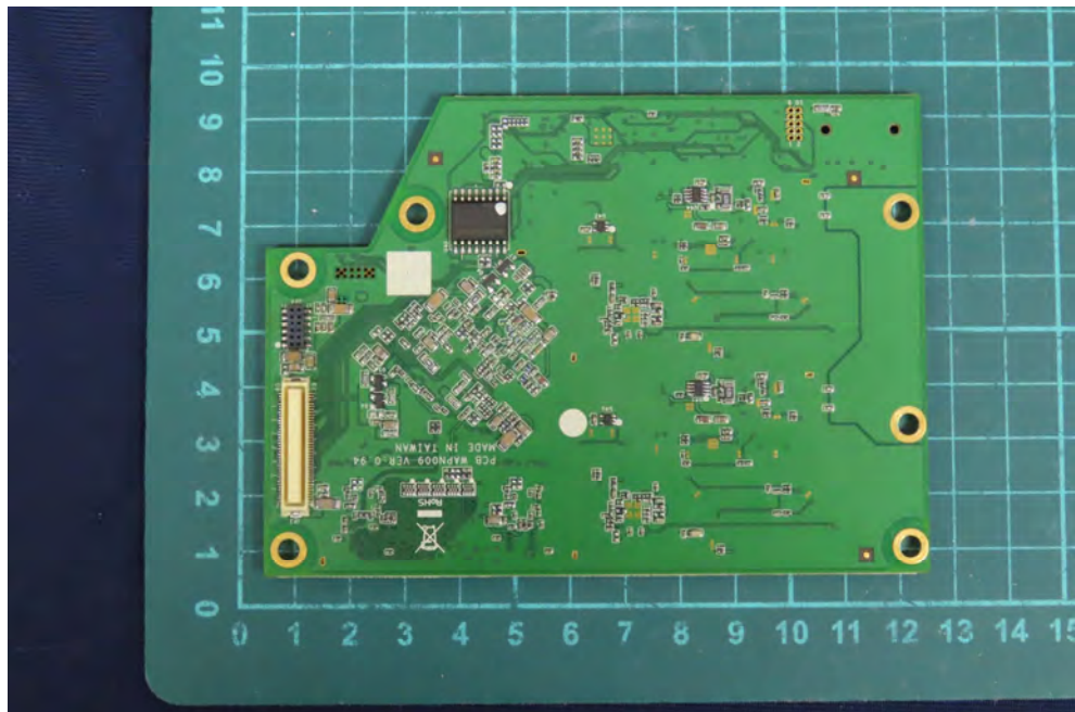
(18) EUT Photo
