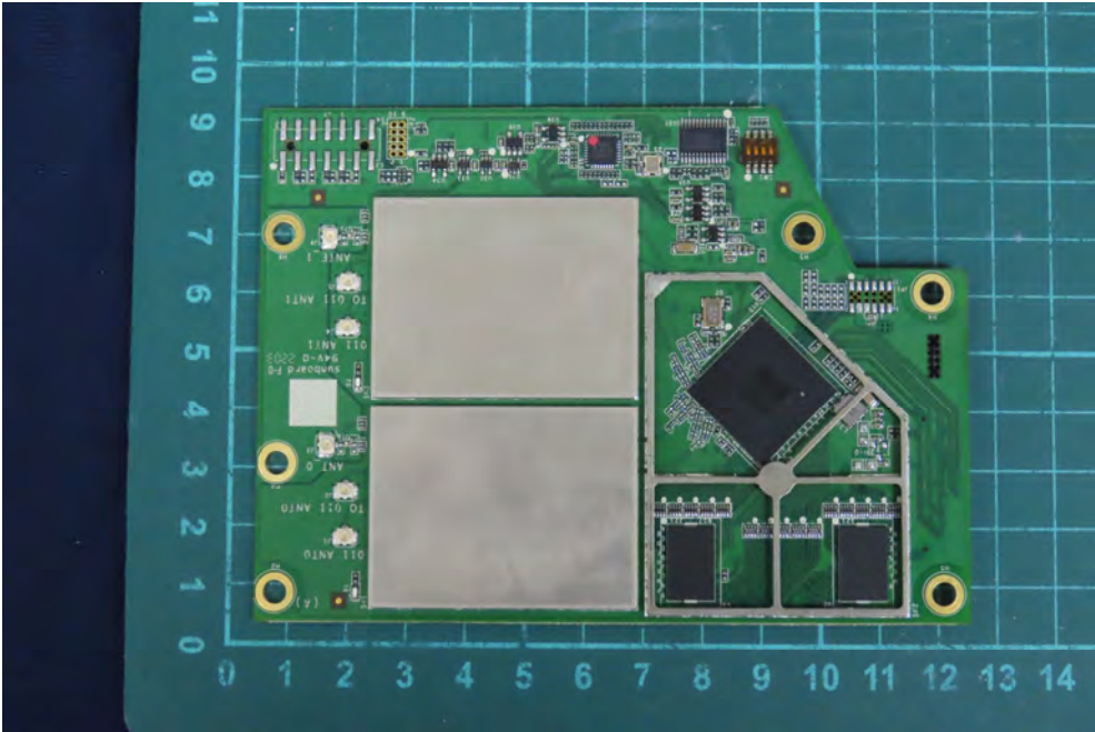
(19) EUT Photo
