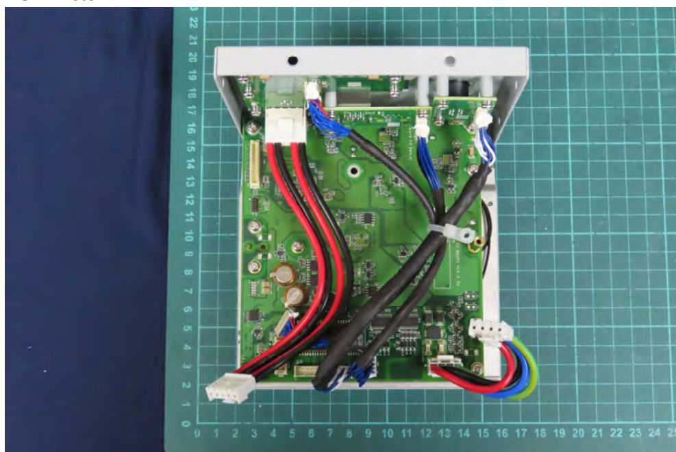
(12) EUT Photo
