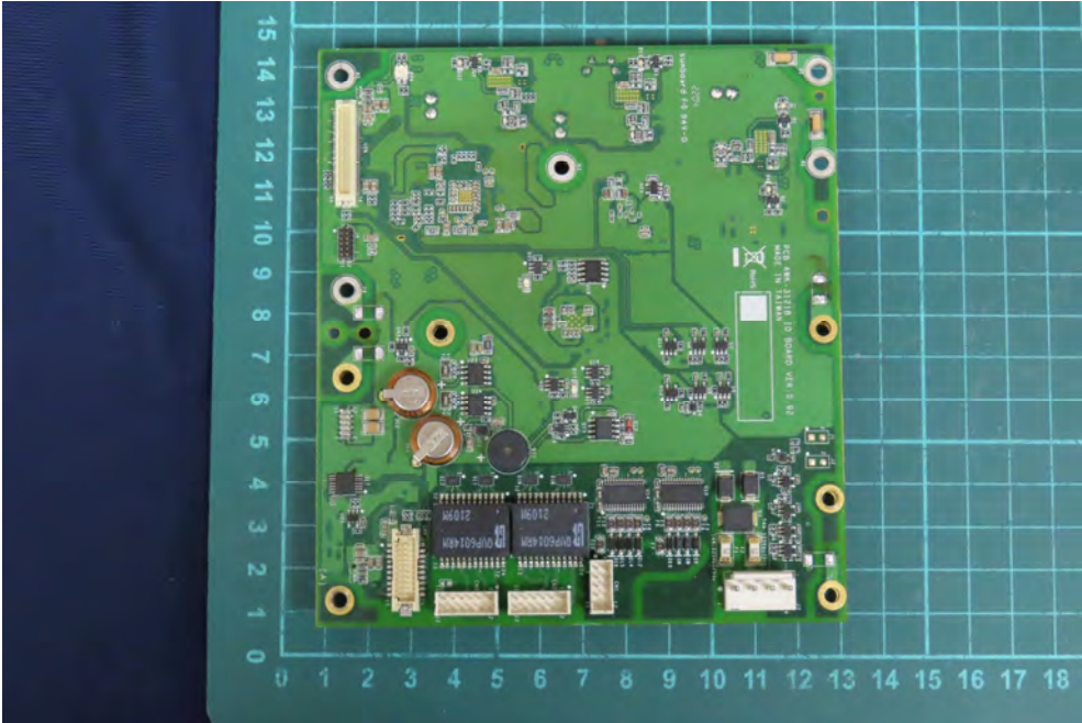
(14) EUT Photo
