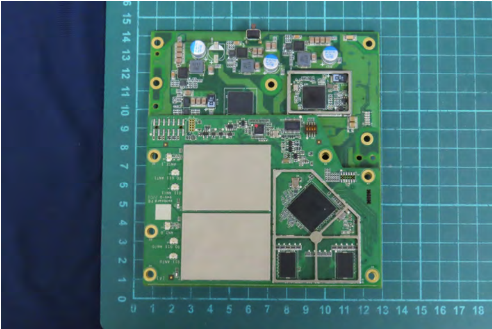
(15) EUT Photo
