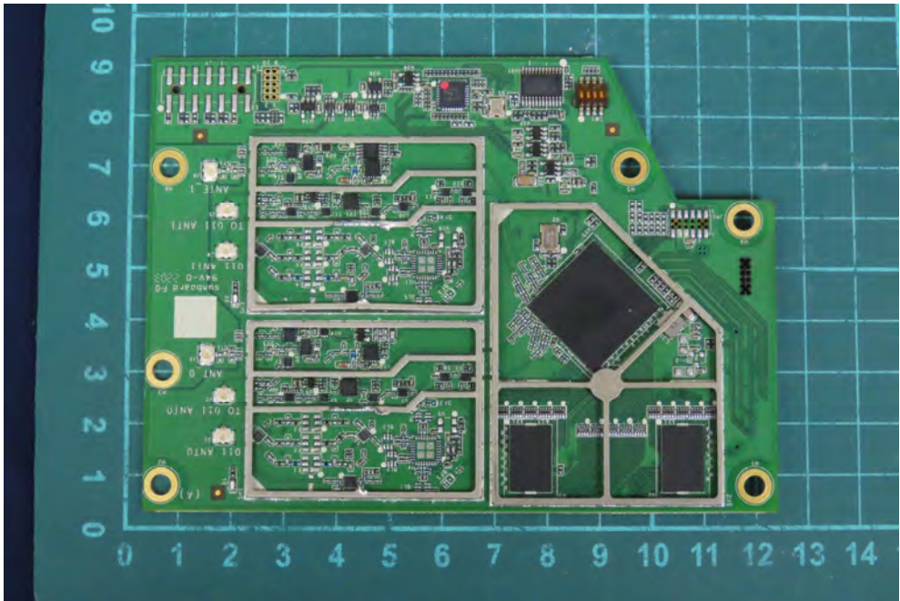
(21) EUT Photo
