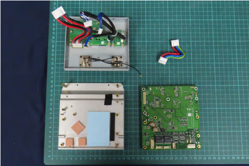
(13) EUT Photo
