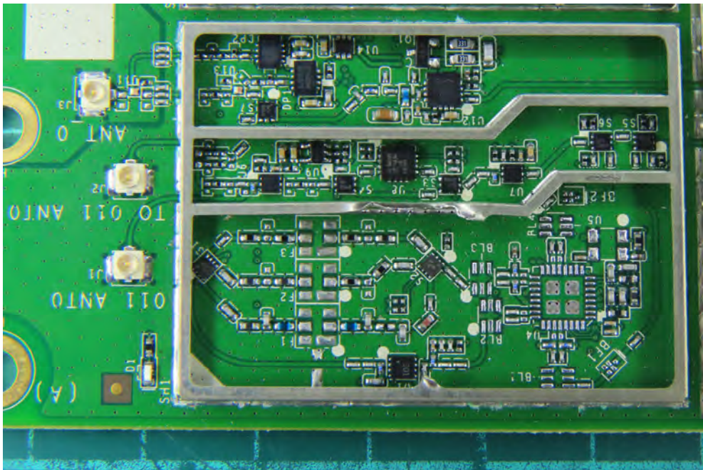
(24) EUT Photo
