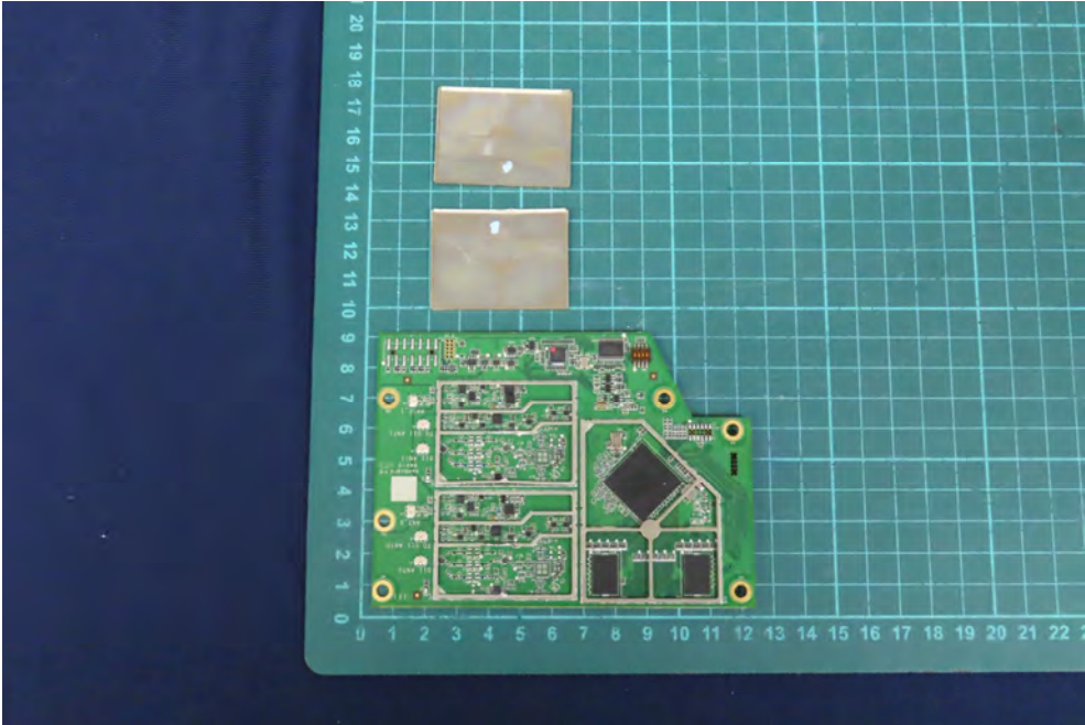
(20) EUT Photo
