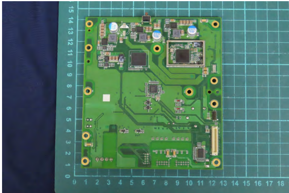
(17) EUT Photo
