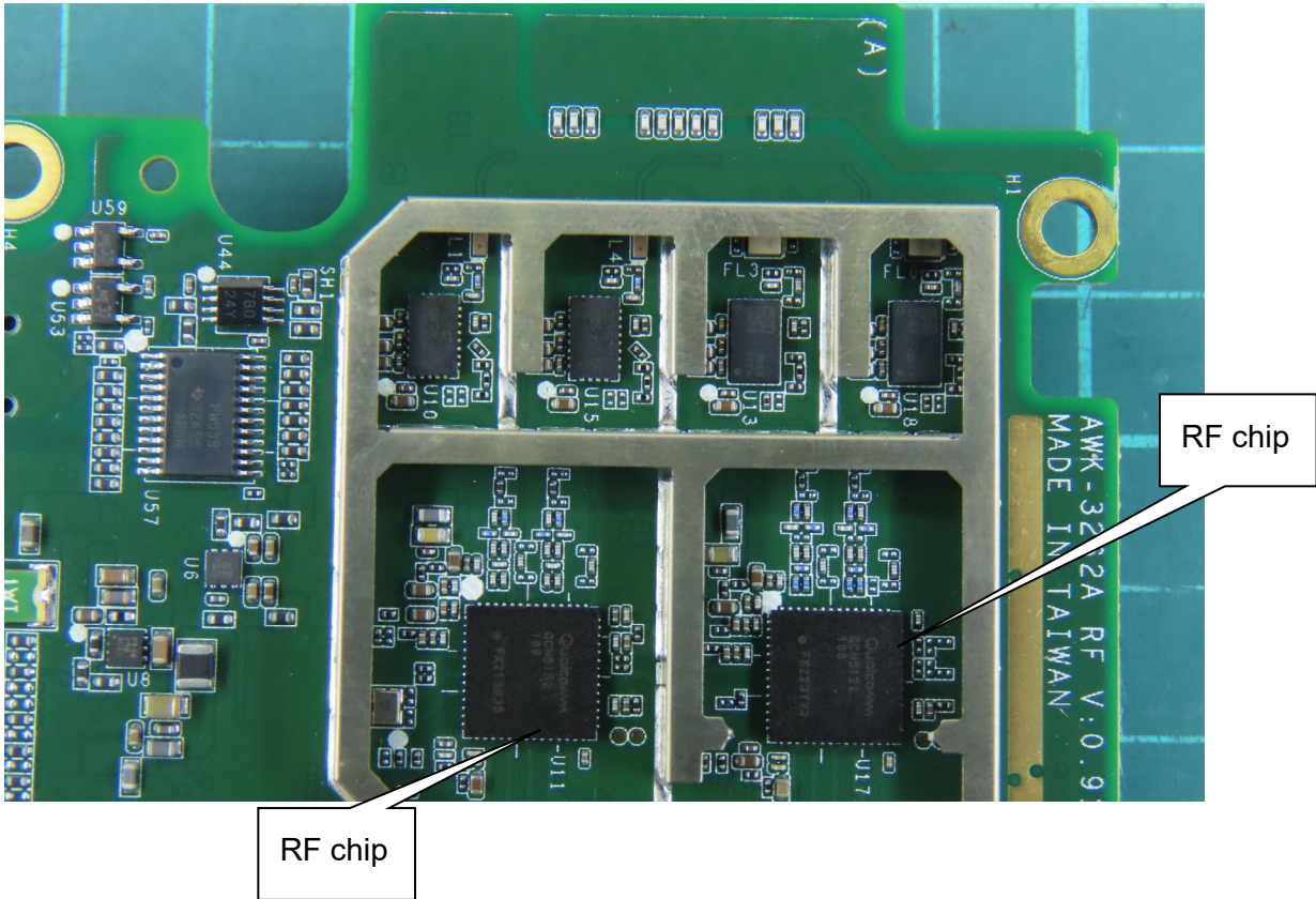
(30) EUT Photo
