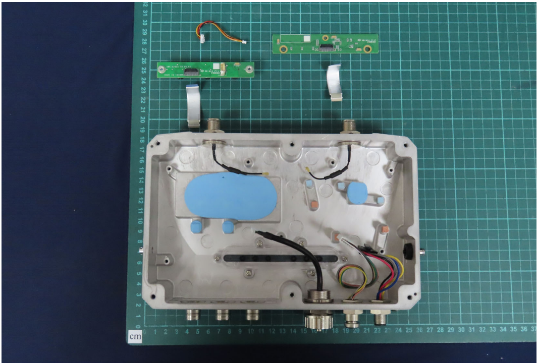
(58) EUT Photo
