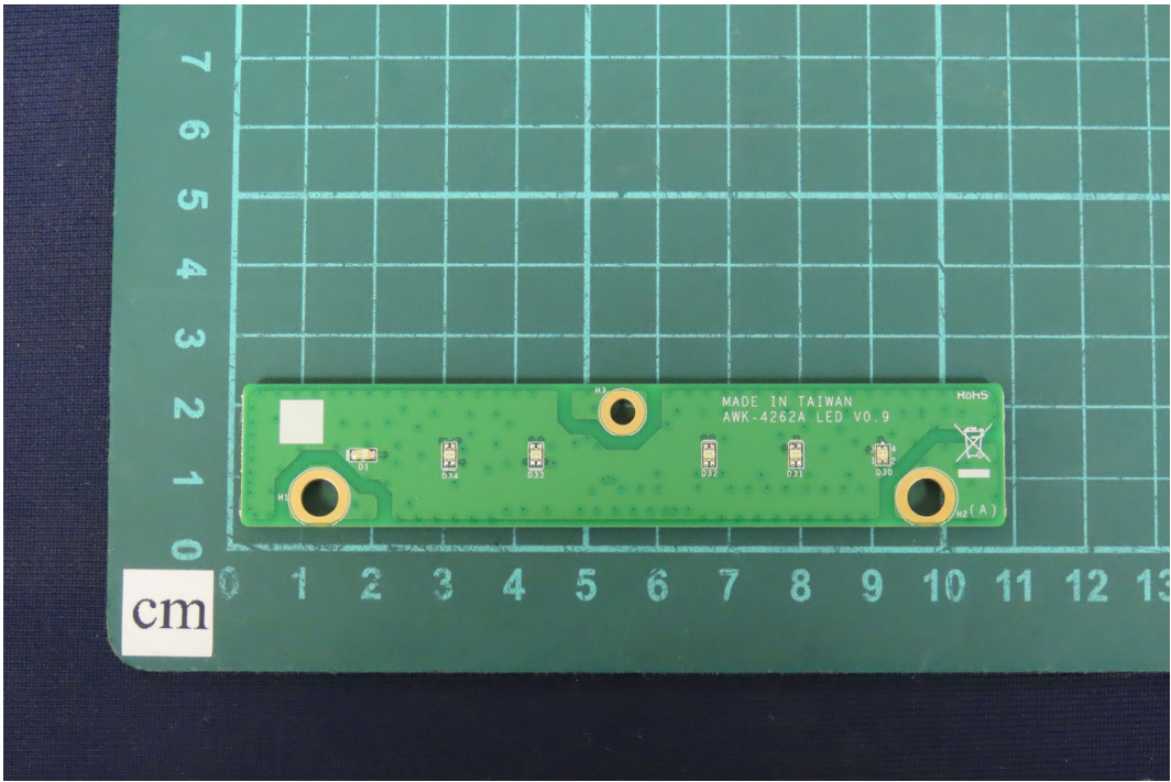
(62) EUT Photo
