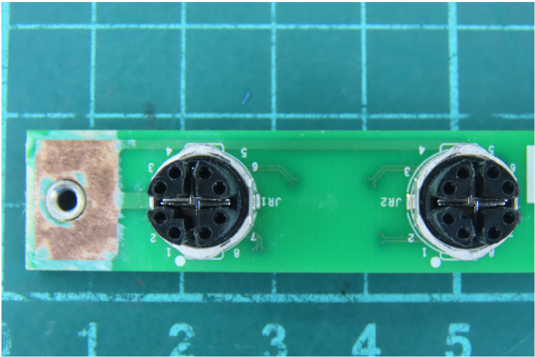
(70) EUT Photo
