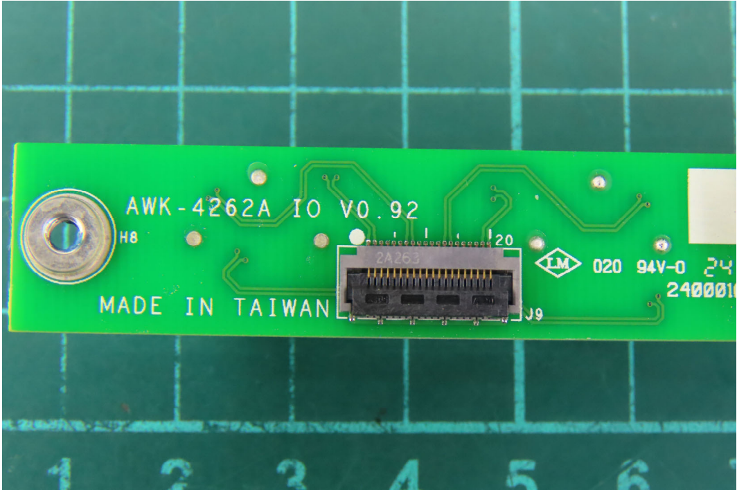
(67) EUT Photo
