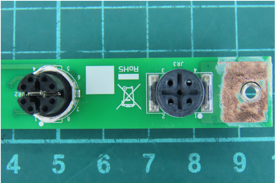
(69) EUT Photo
