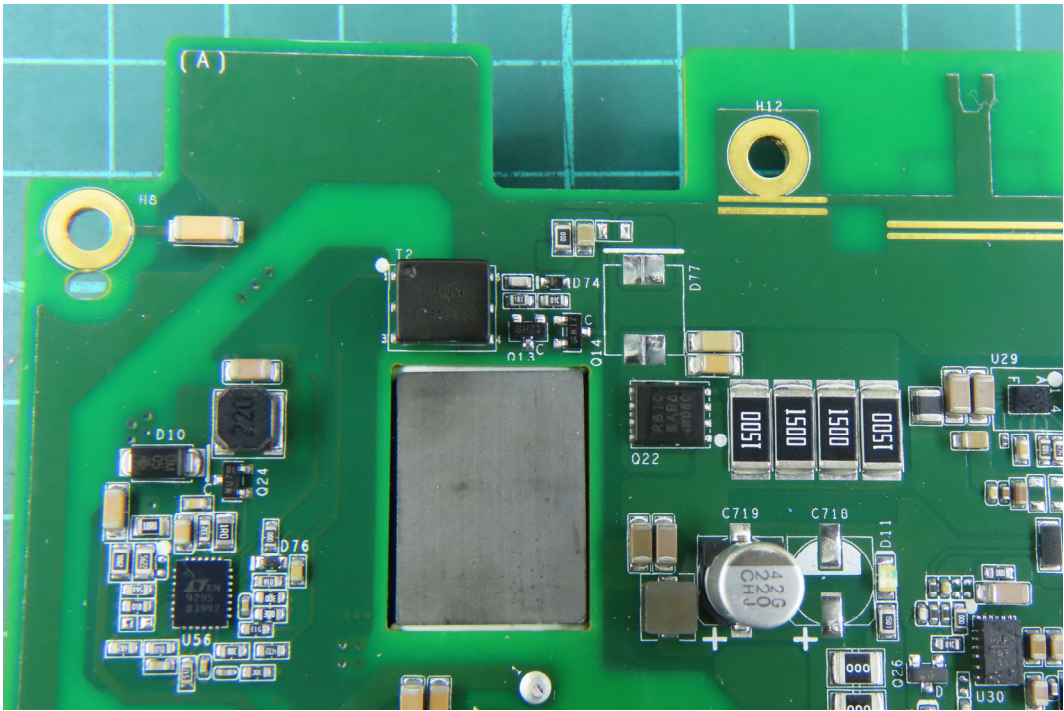
(56) EUT Photo
