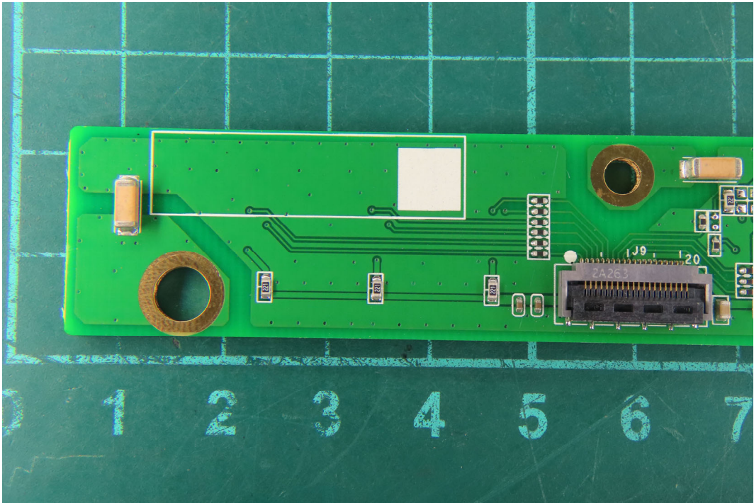
(61) EUT Photo
