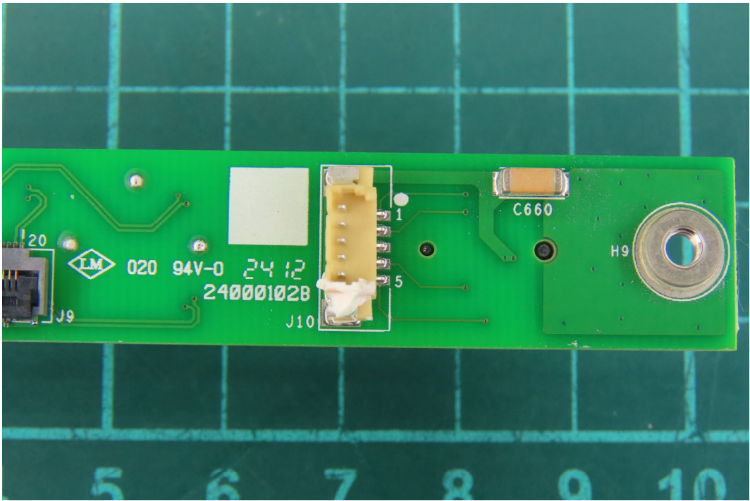
(66) EUT Photo
