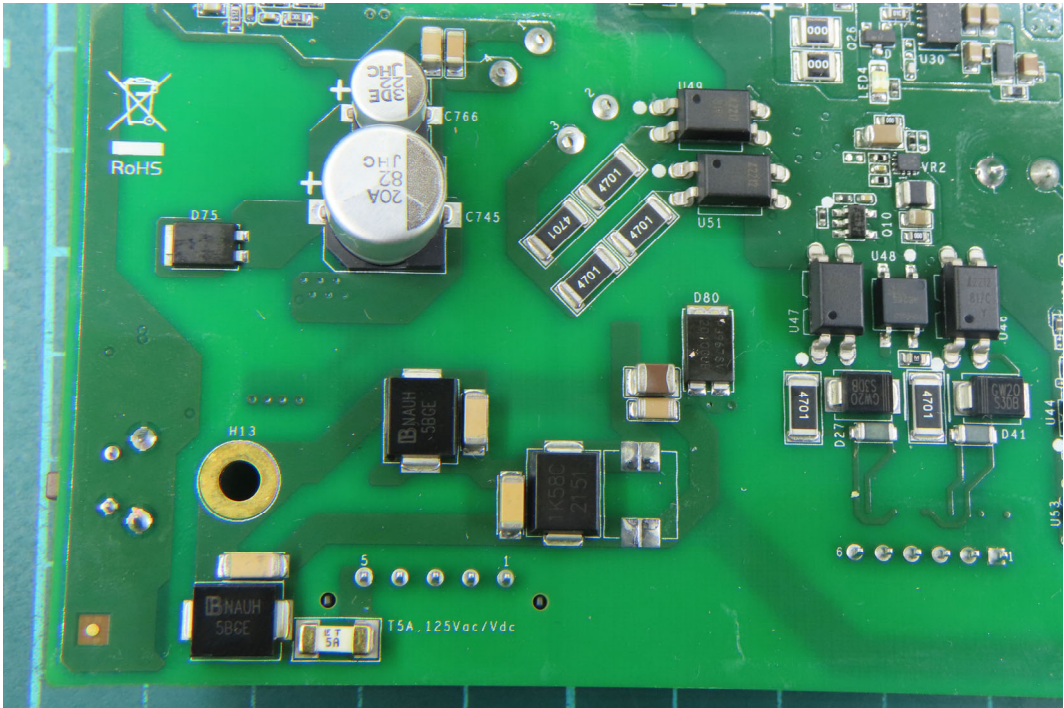
(57) EUT Photo
