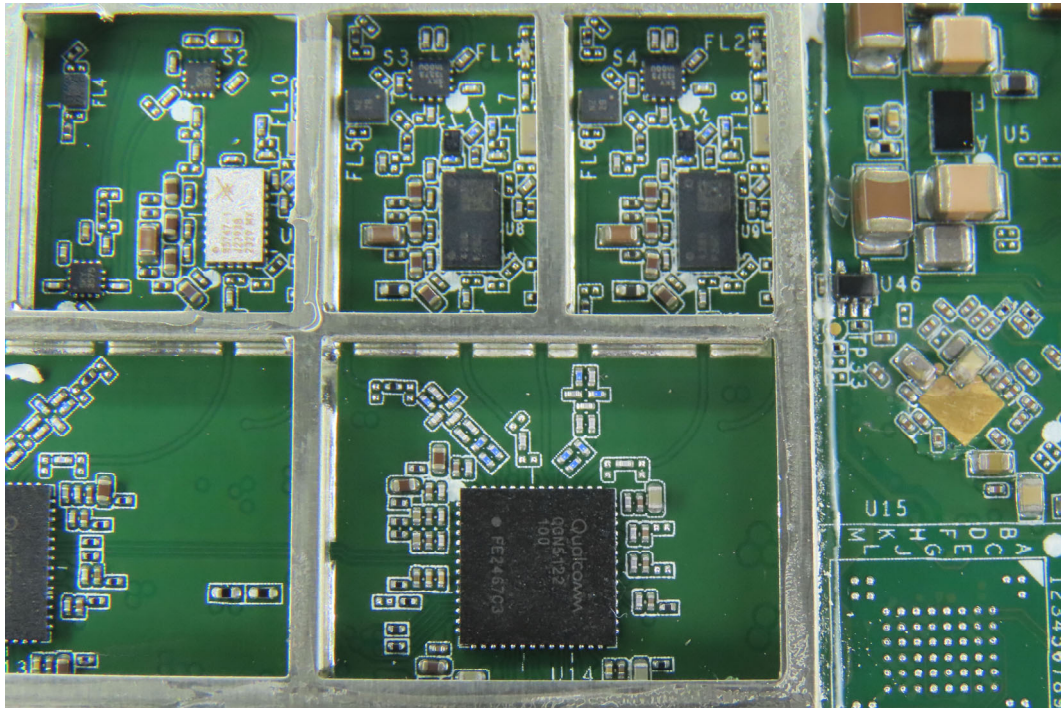
(61) EUT Photo
