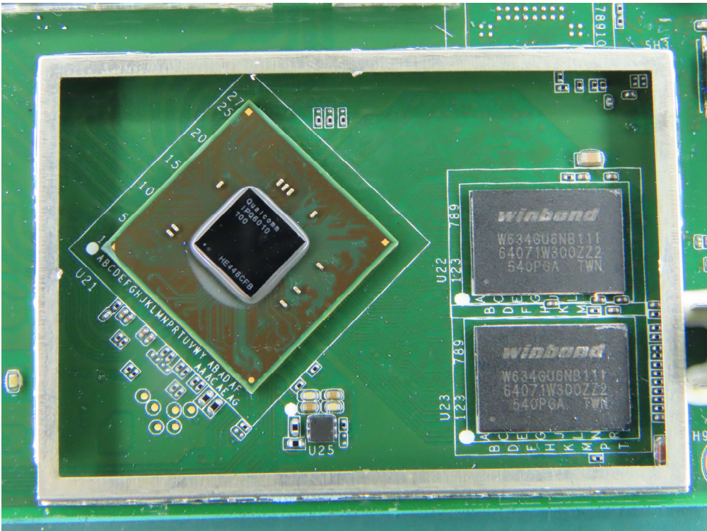
(40) EUT Photo
