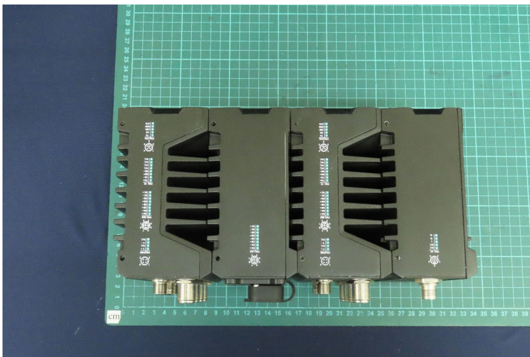
(8) EUT Photo
