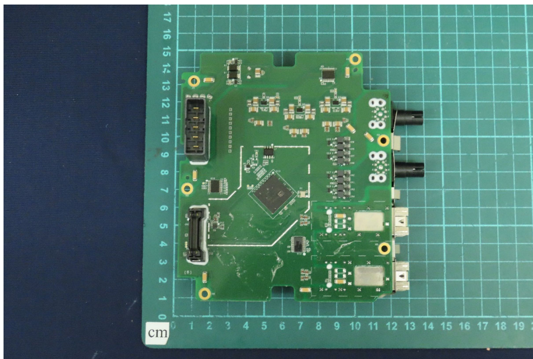
(84) EUT Photo
