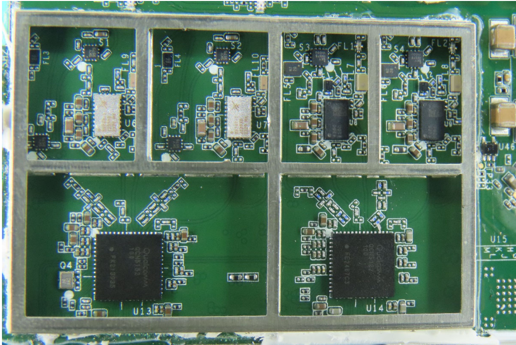
(72) EUT Photo
