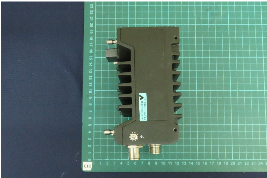
(59) EUT Photo
