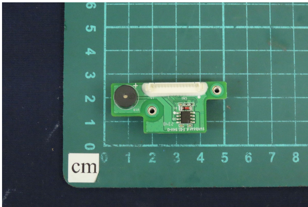
(67) EUT Photo
