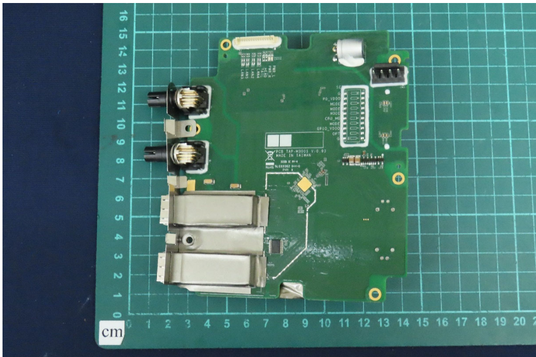
(81) EUT Photo
