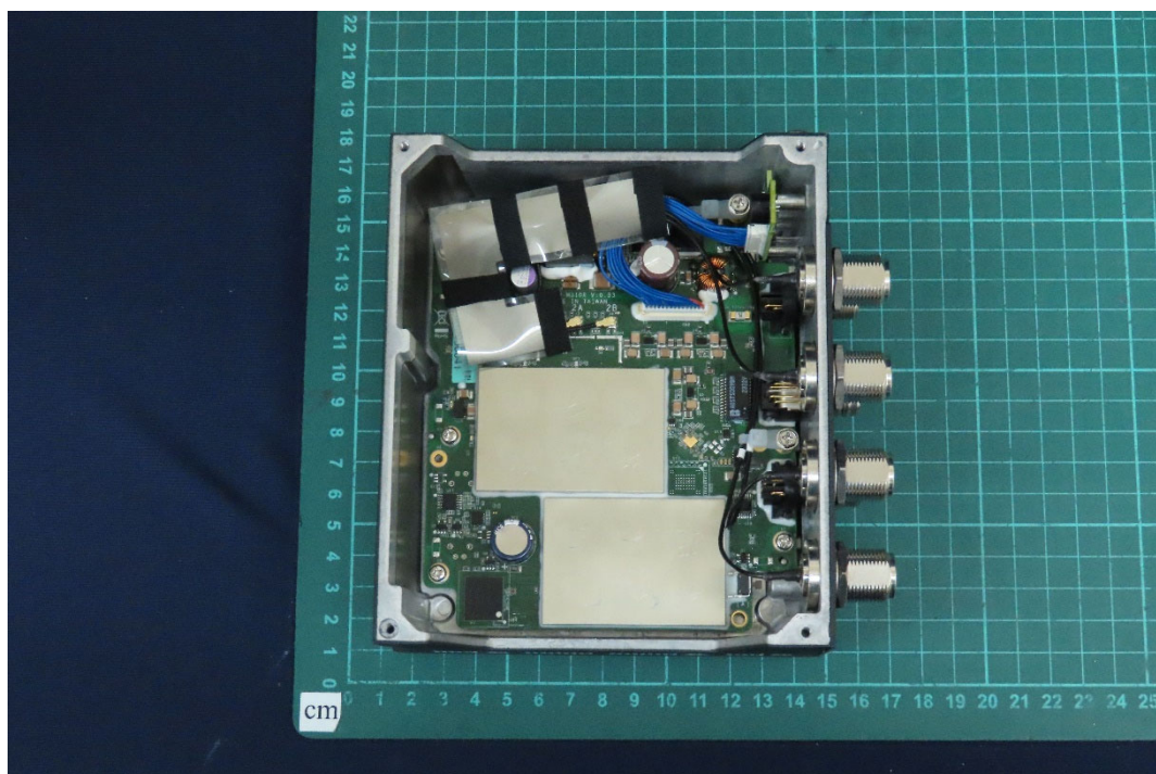
(65) EUT Photo
