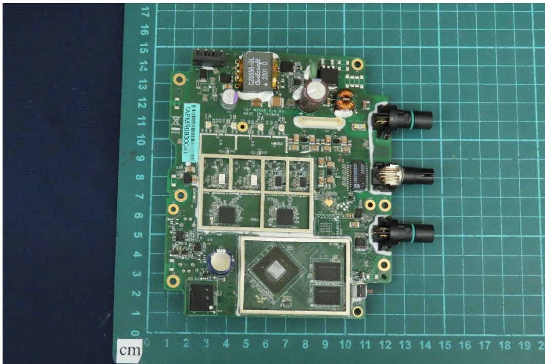
(71) EUT Photo
