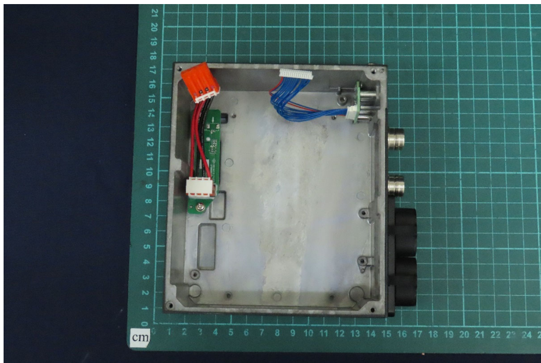
(85) EUT Photo
