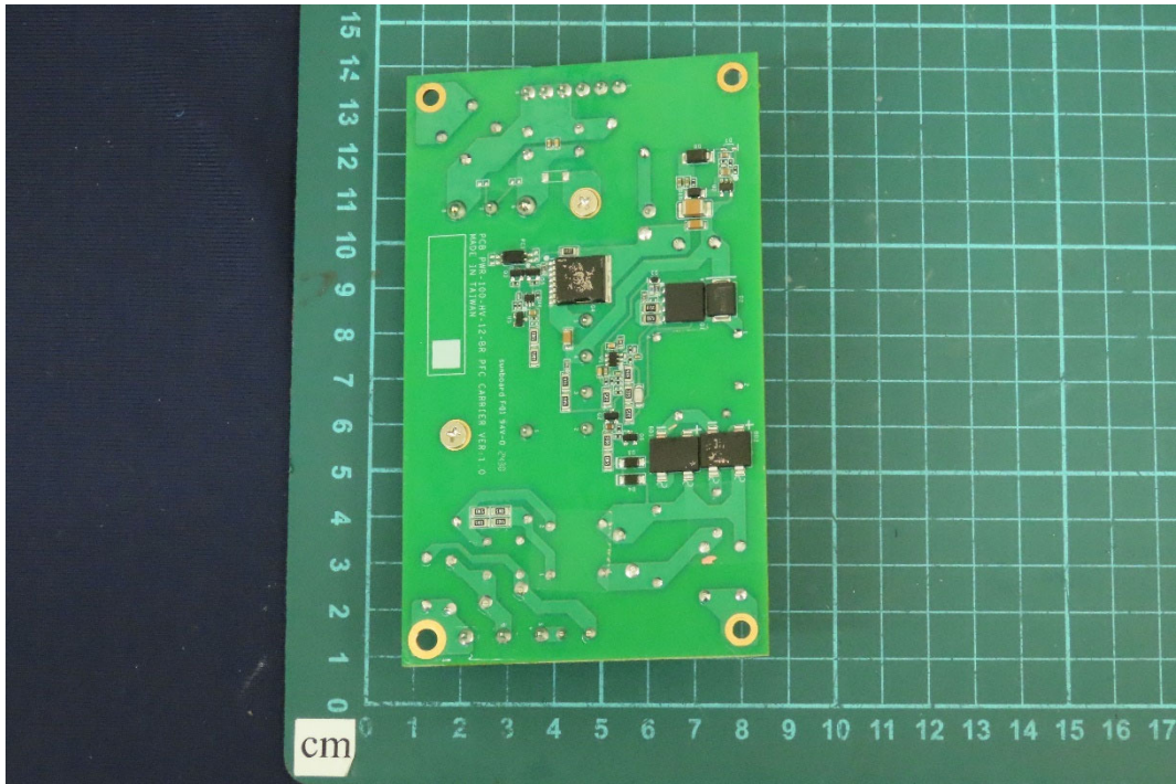
(58) EUT Photo
