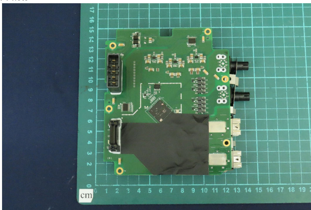
(82) EUT Photo
