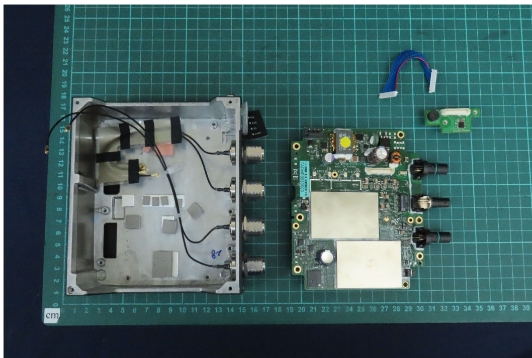
(98) EUT Photo
