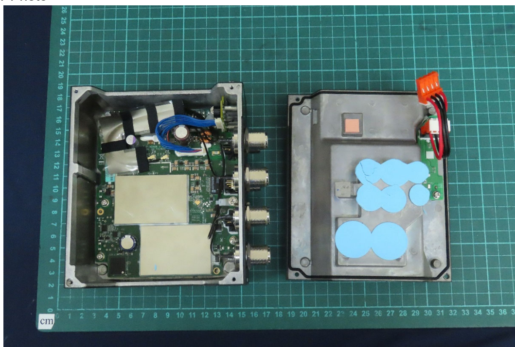
(92) EUT Photo
