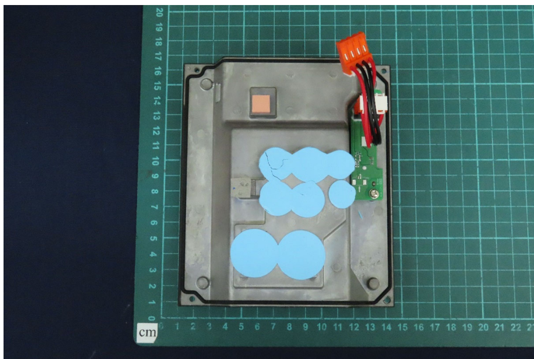
(93) EUT Photo
