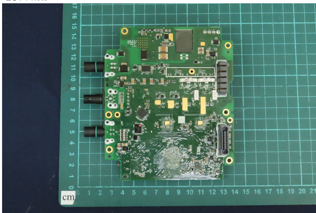
(106) EUT Photo
