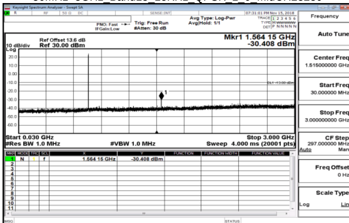
30MHz~3GHz Band13 15KHz QPSK 1 0 MidCH23230
