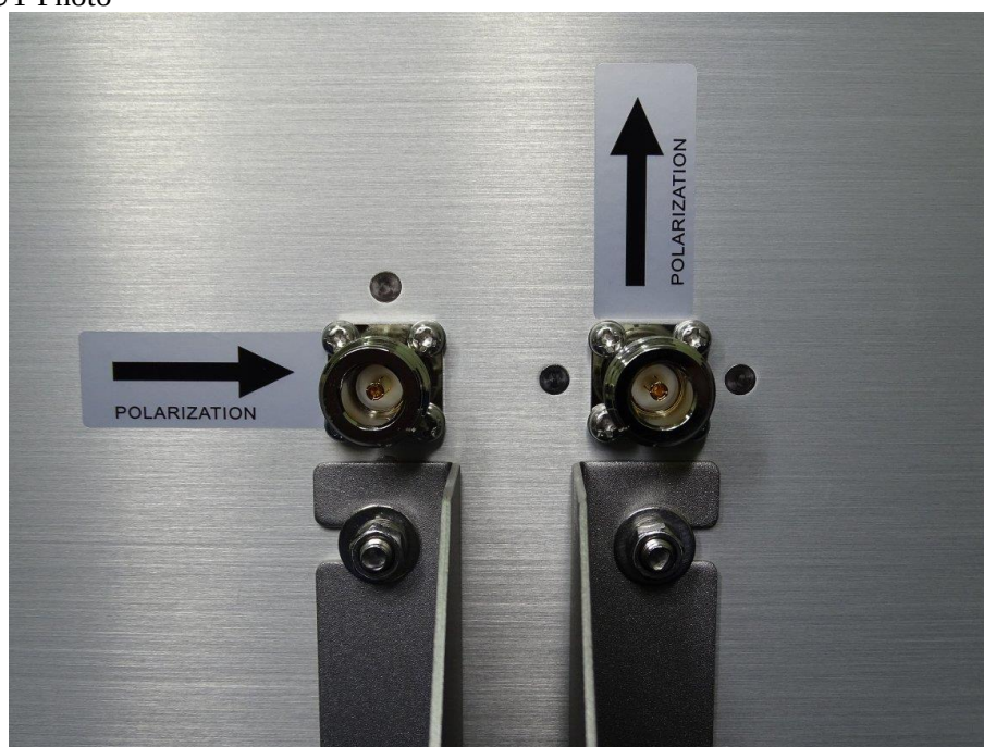
(57) EUT Photo
