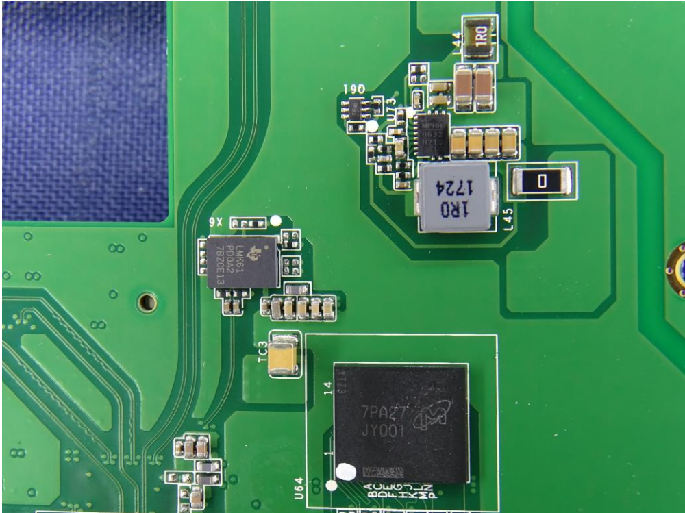
(36) EUT Photo
