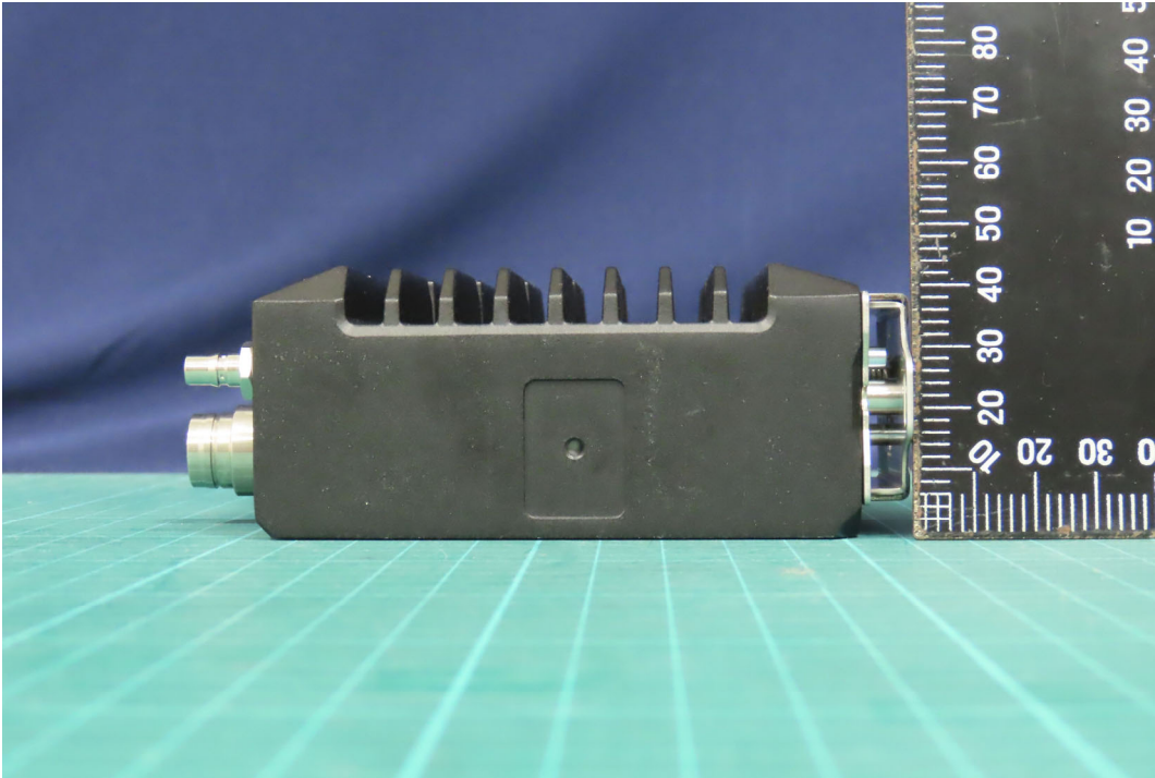
(4) EUT Photo
