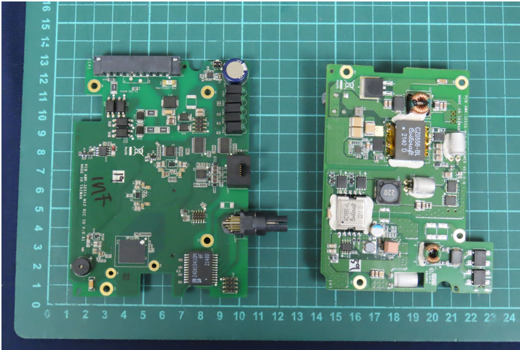
(5) EUT Photo
