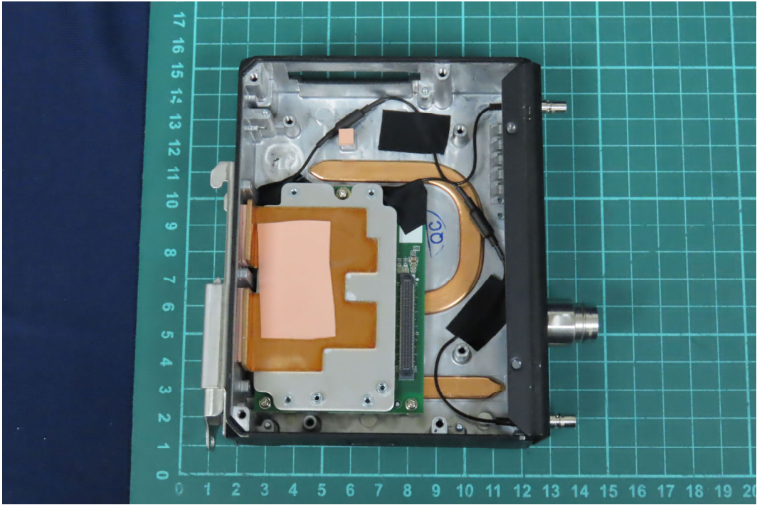
(10) EUT Photo
