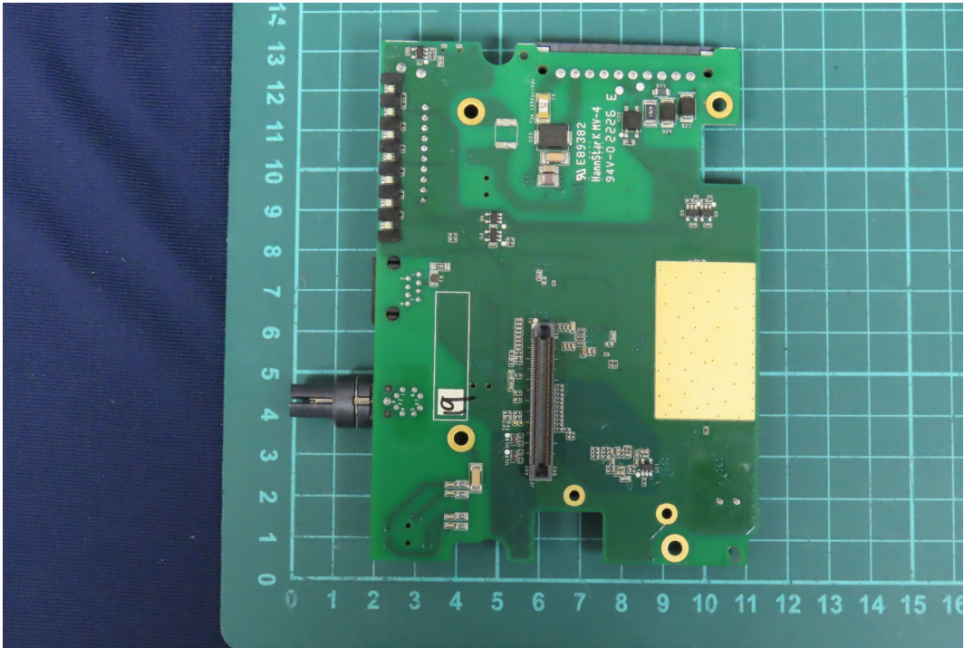
(9) EUT Photo
