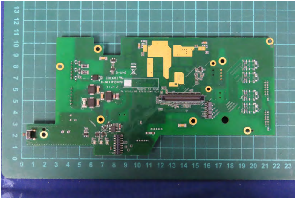
(15) EUT Photo
