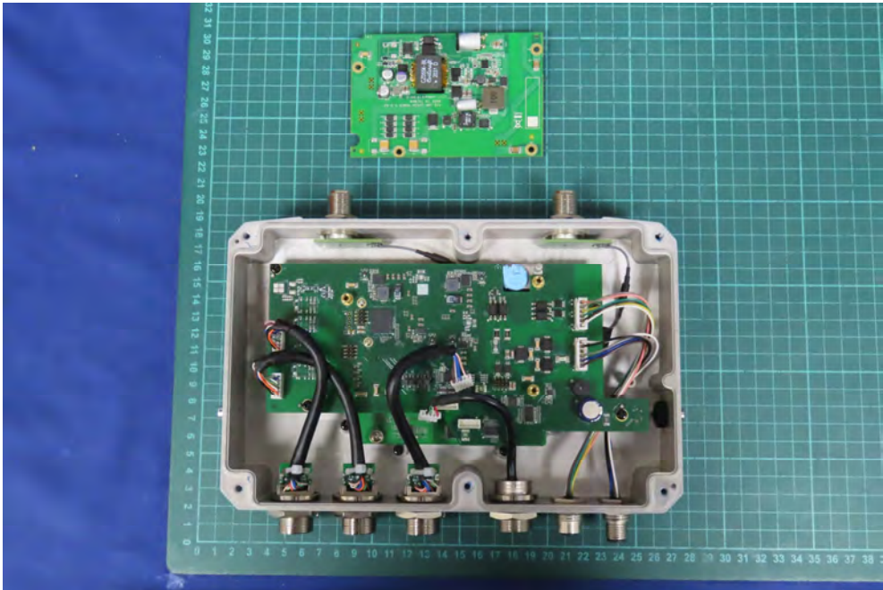
(9) EUT Photo
