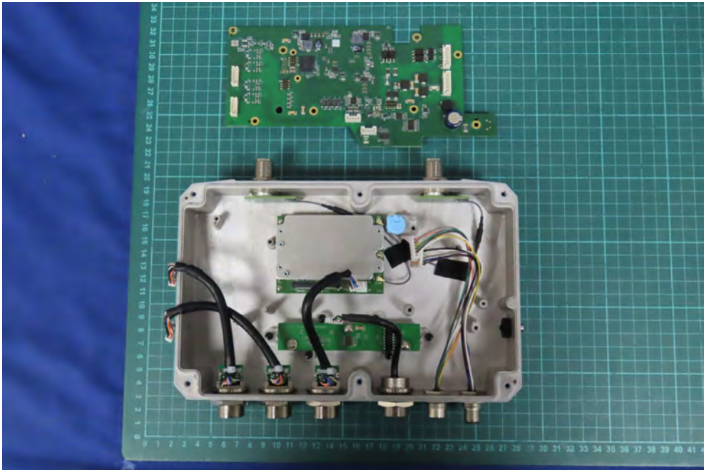
(13) EUT Photo
