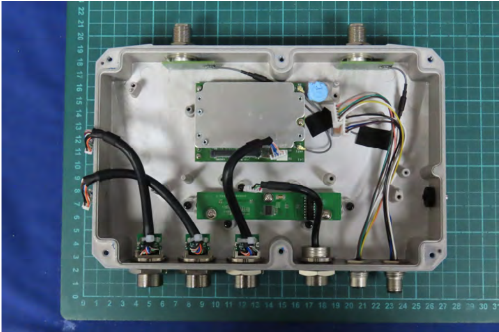
(16) EUT Photo
