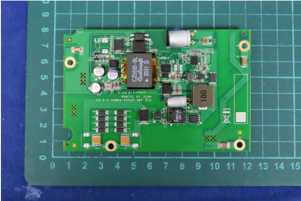
(10) EUT Photo
