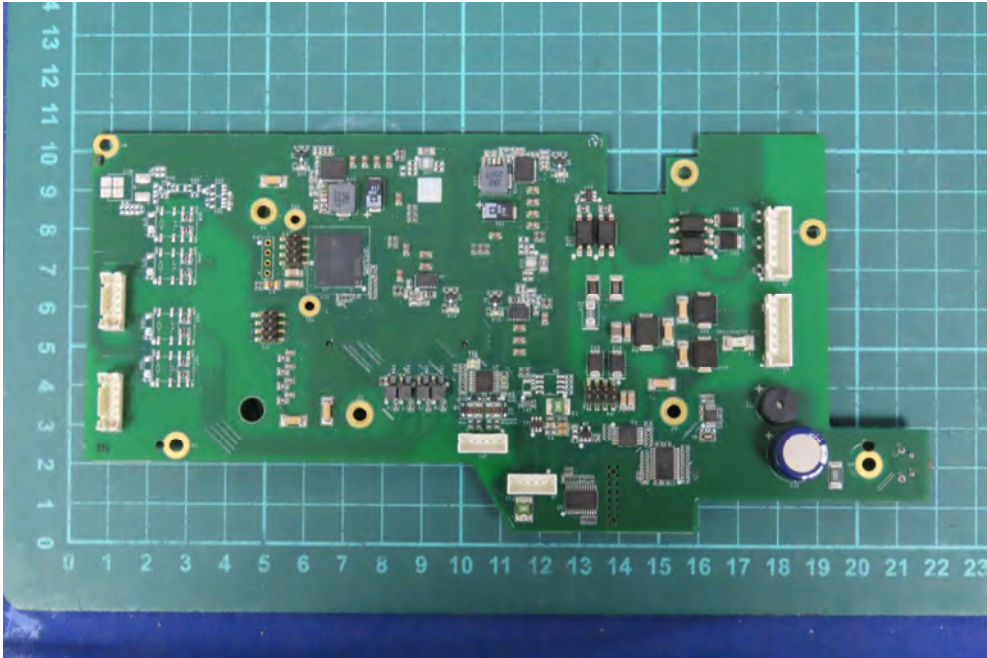
(14) EUT Photo
