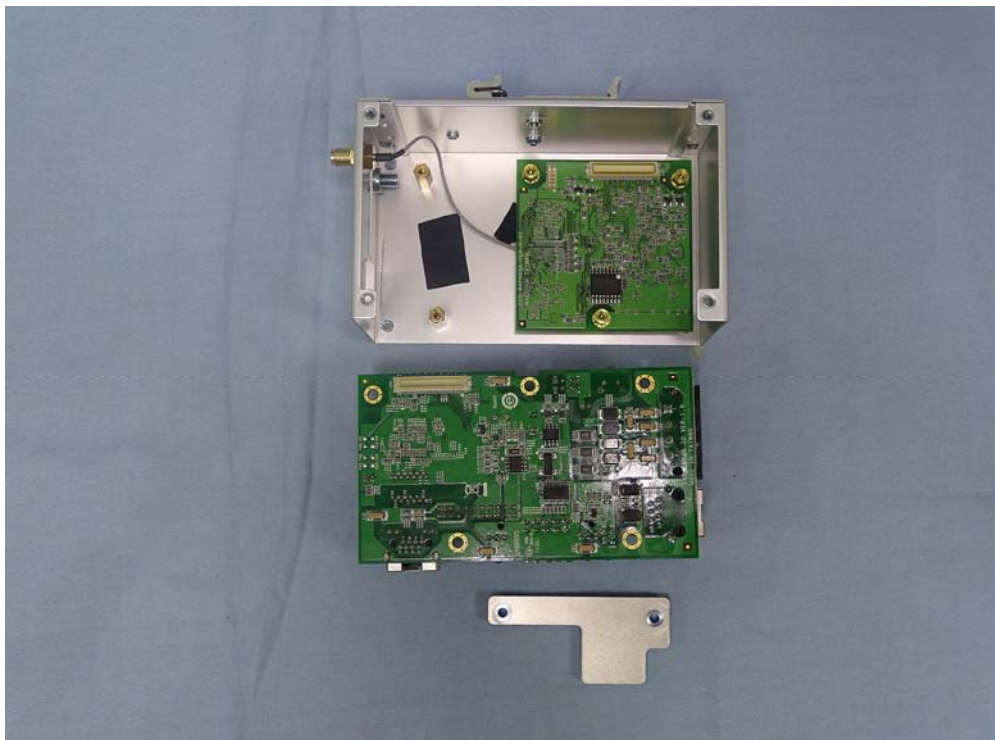
(12) EUT Photo
