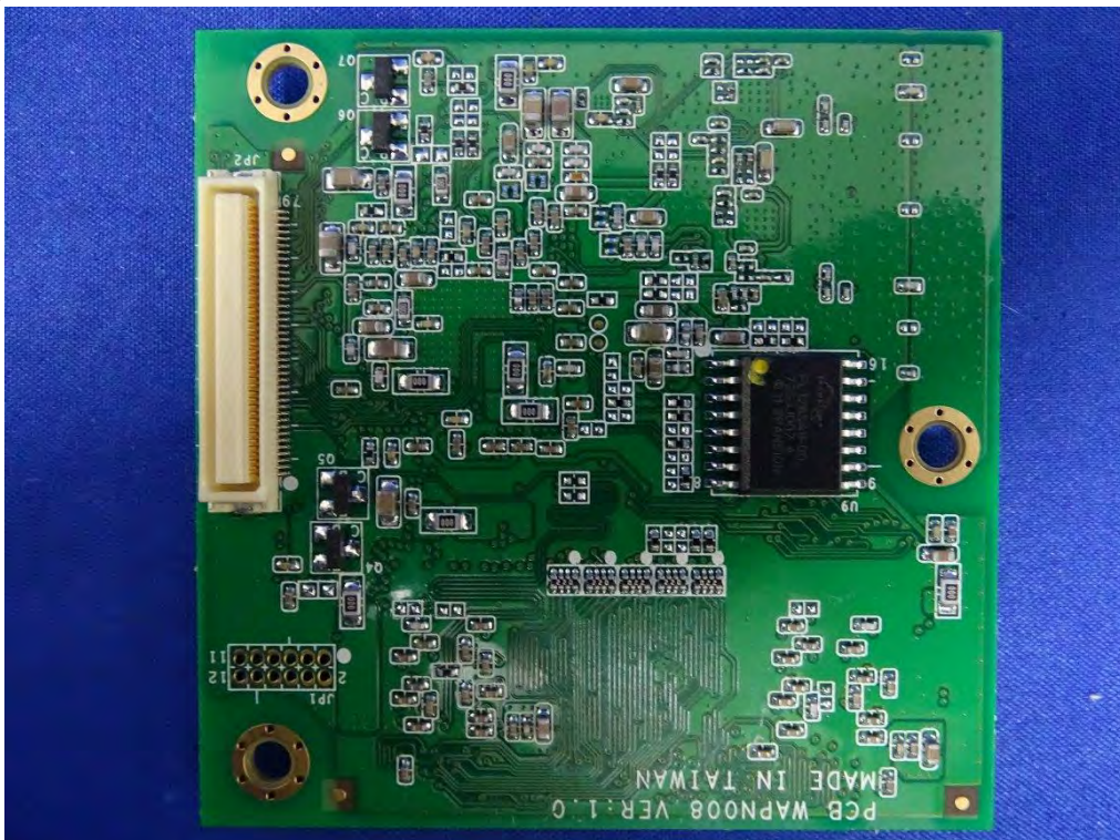
(58) EUT Photo
