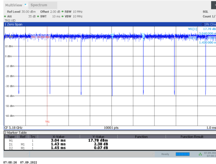
11a-CDD_Wifi1_5180
