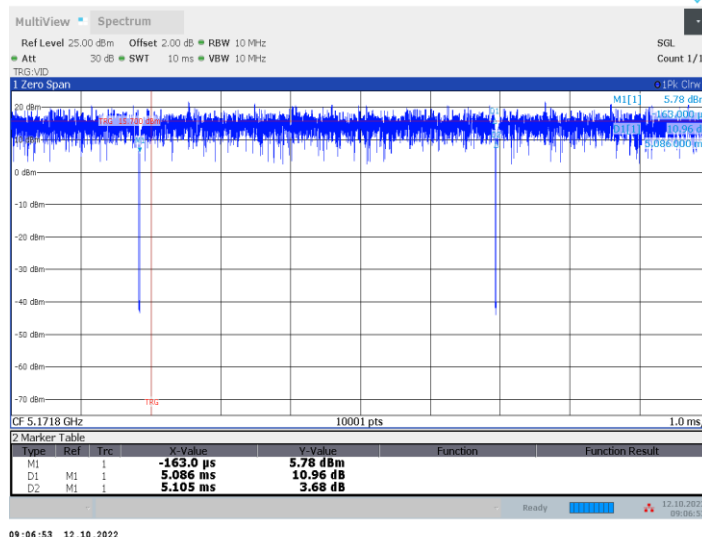
11ax20MIMO_Wifi0_5180_52Tone_RU37
