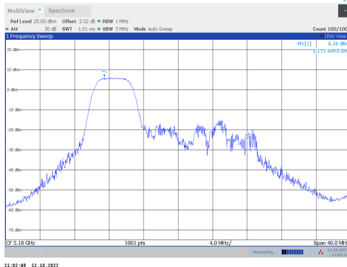
11ax20MIMO_Wifi0_5180_52Tone_RU37
