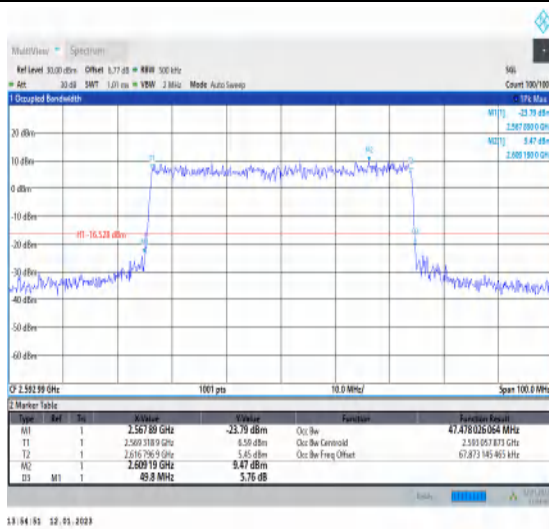
1-N41-PC3-30-50-M-7-CP-16QAM-Outer_Full-133@ 0-Ant1-47.478-49.800-≤50-PASS
