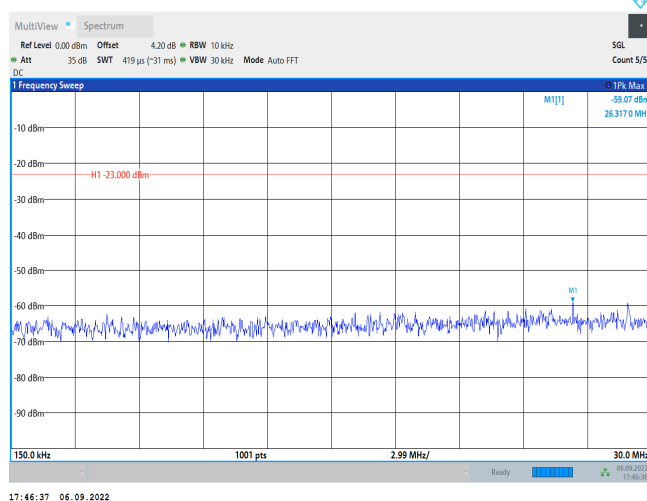
Band4-20MHz-QPSK-20050-1RB#0-Range2:0.15~30MHz
