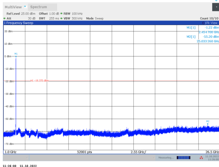
11n40MIMO Wifi1 2452 1000~26500
