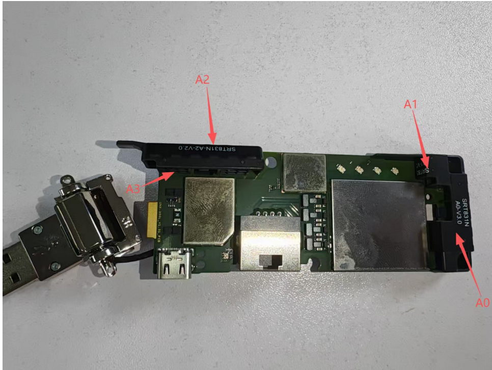
A0: LTE Main Antenna, A1: 5G NR Main Antenna, A2: LTE Div Antenna, A3: 5G NR Div Antenna,
