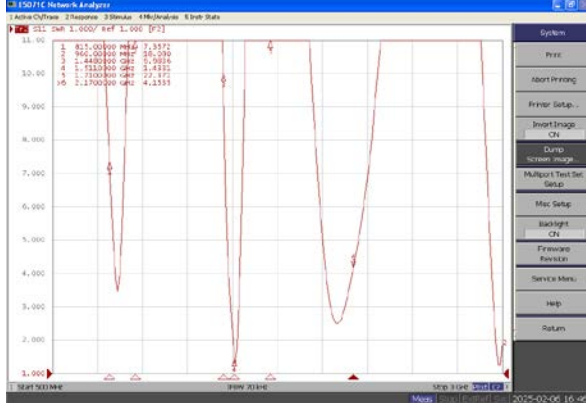
Div Antenna VSWR
