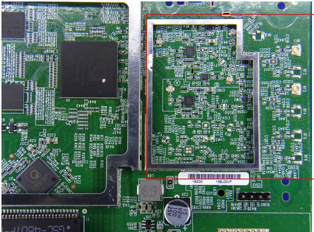
(18) EUT Photo-Module 2.4G
