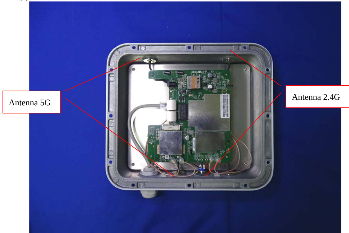
(6) EUT Photo
