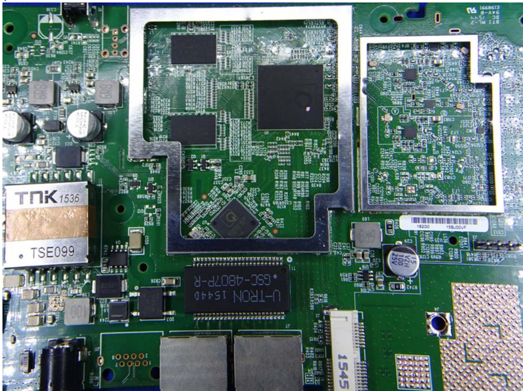
(18) EUT Photo-Module 2.4G
