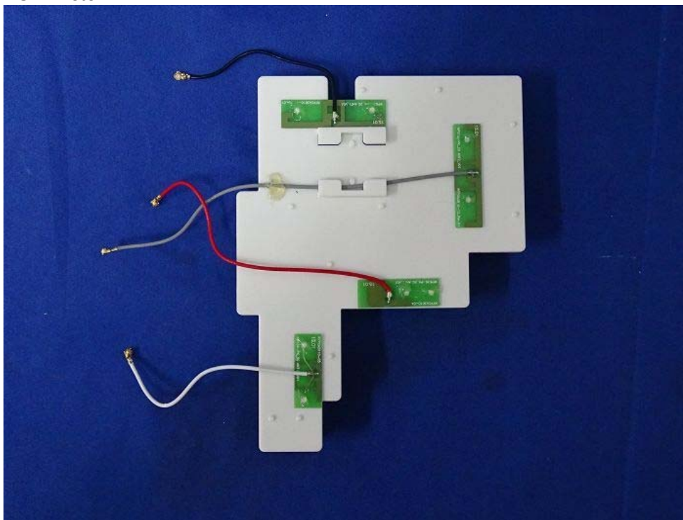
(30) EUT Photo
