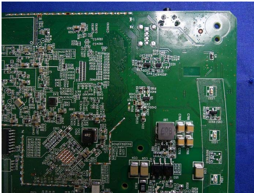
(24) EUT Photo
