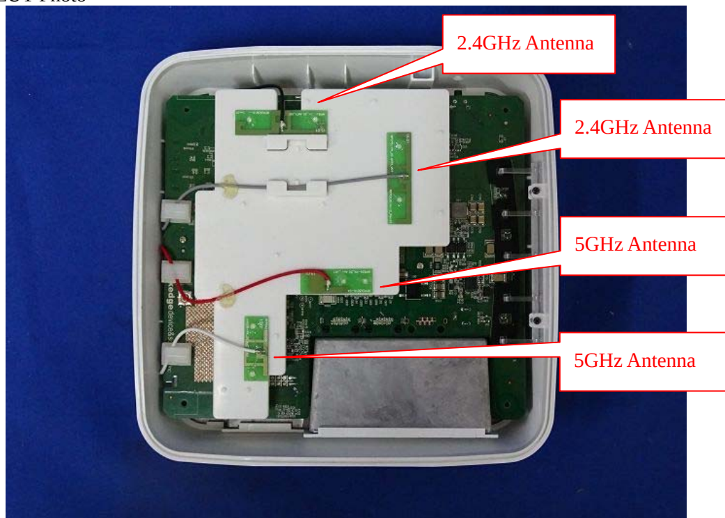
(9) EUT Photo
