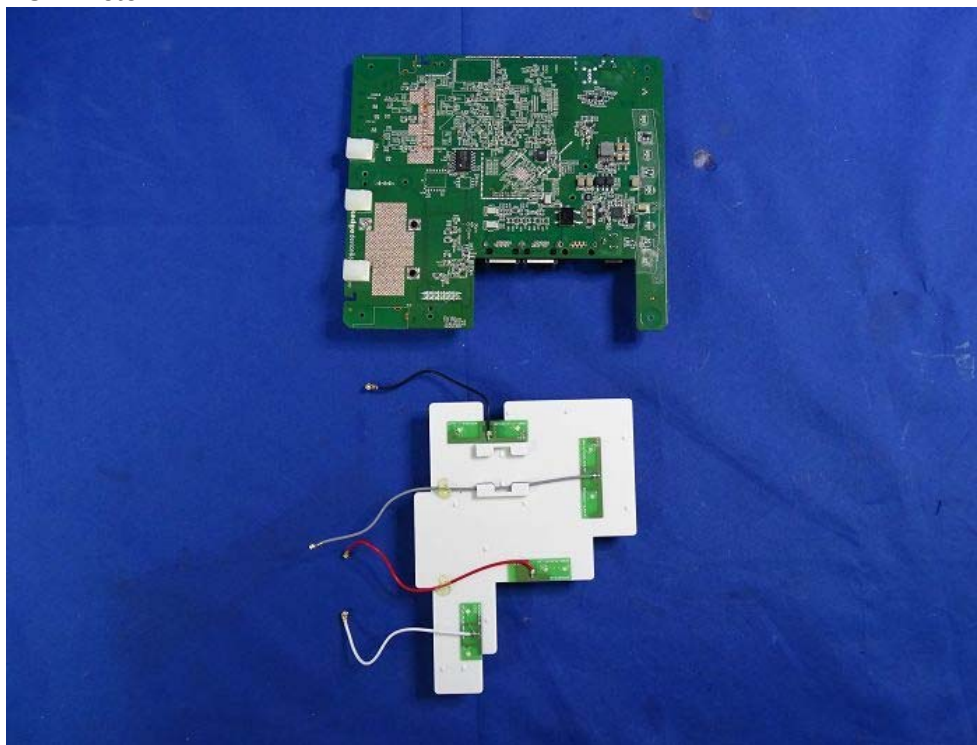
(12) EUT Photo
