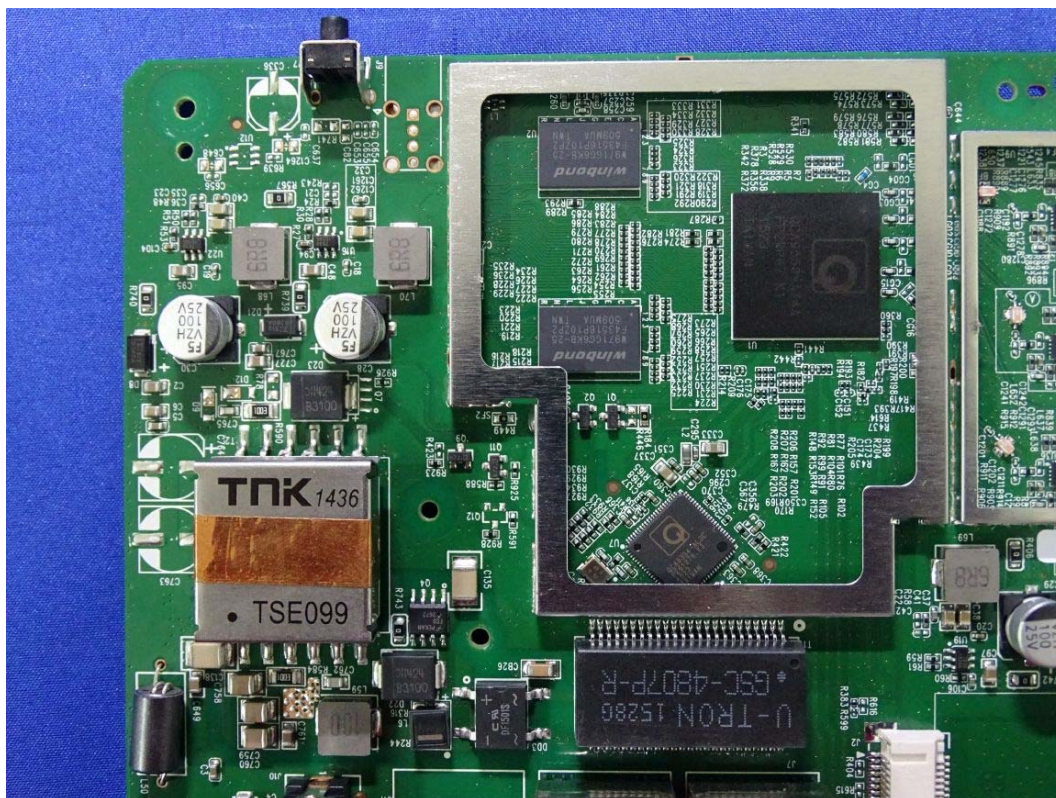
(17) EUT Photo-2.4G Module
