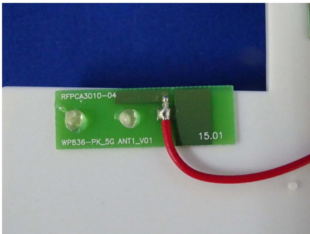
(31) EUT Photo-5G Ant-1
