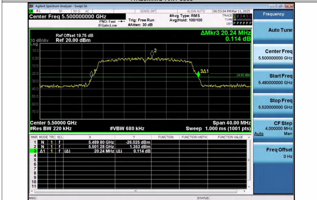
11N20MIMO-Ant2-5500
