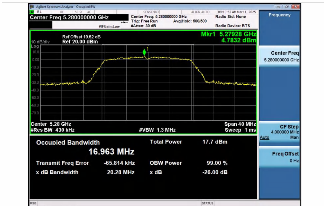
11A-Ant1-5280
