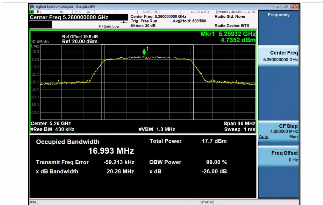
11A-Ant1-5260
