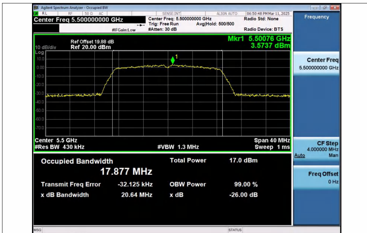
11N20MIMO-Ant1-5500
