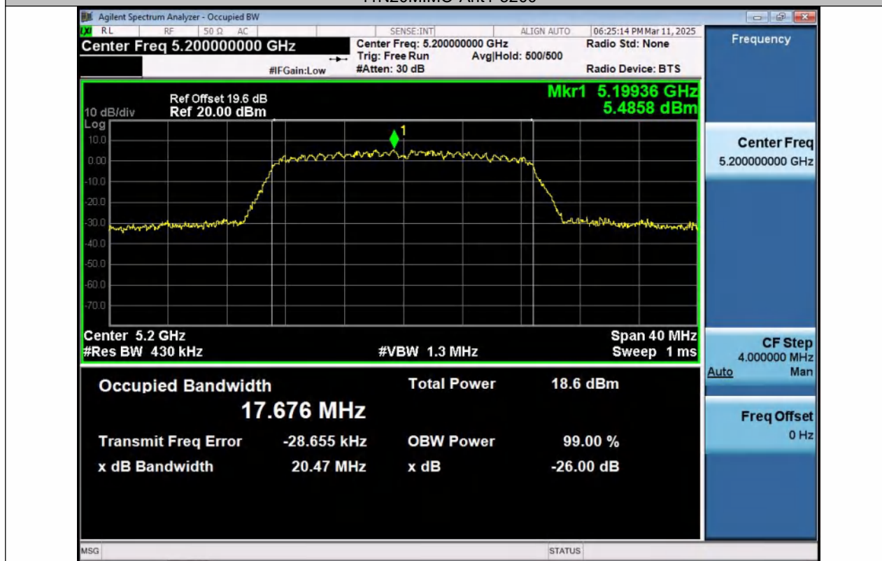
11N20MIMO-Ant2-5200
