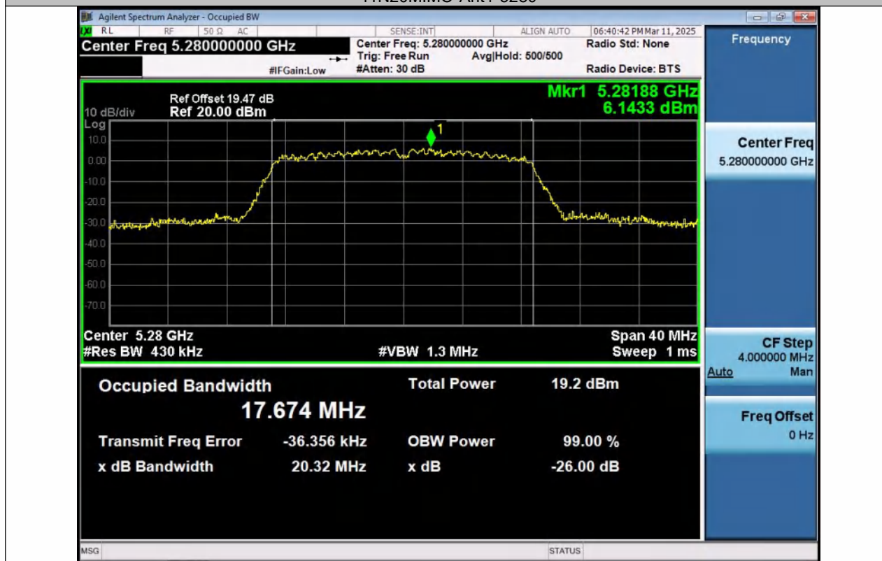
11N20MIMO-Ant2-5280
