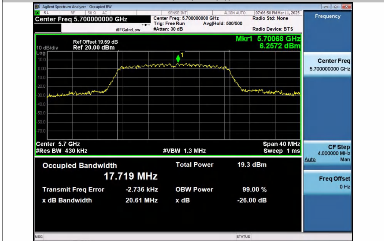
11N20MIMO-Ant2-5700
