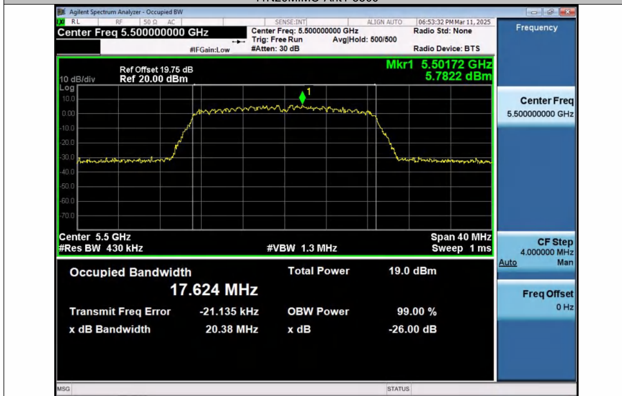
11N20MIMO-Ant2-5500
