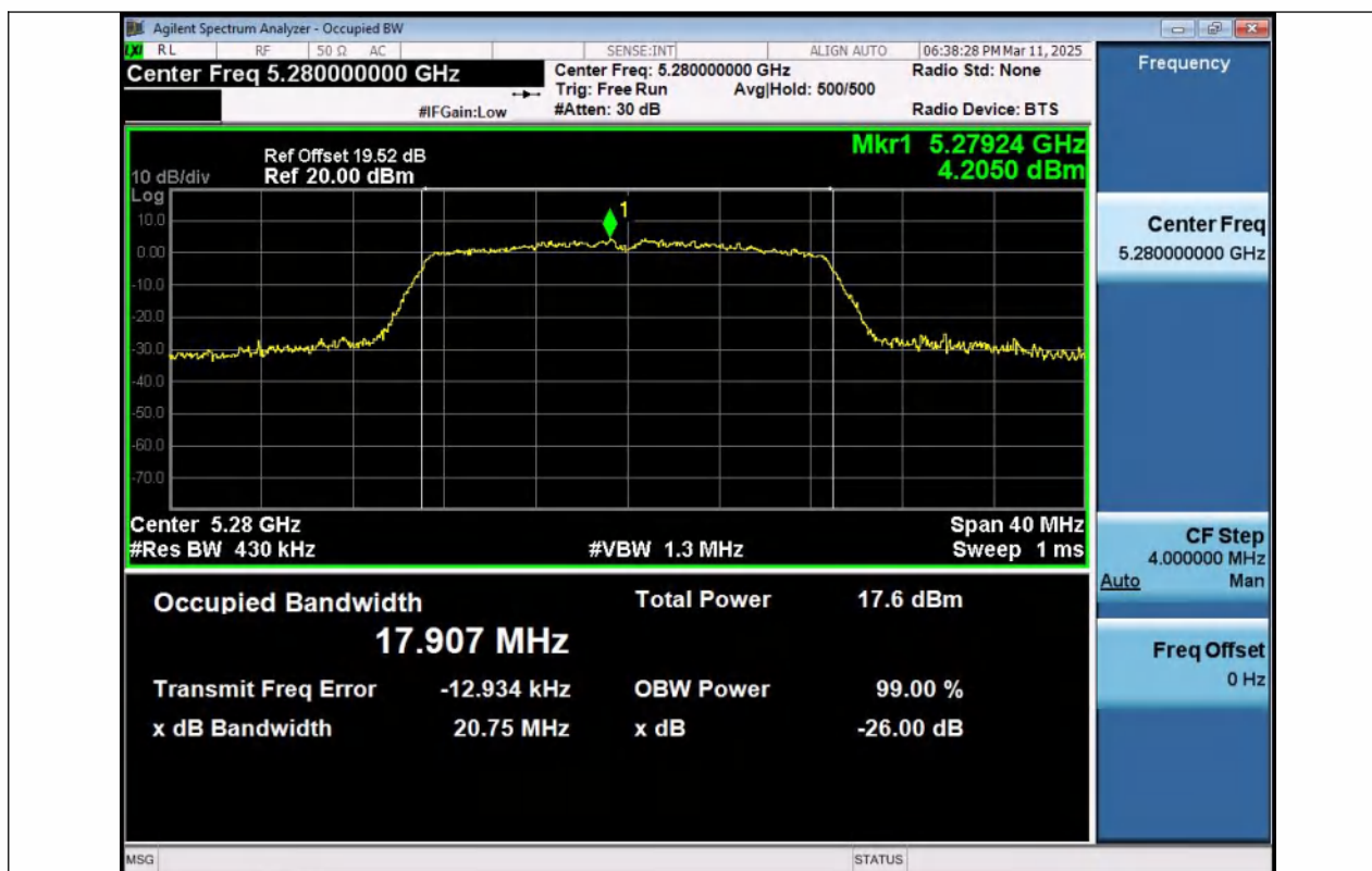
11N20MIMO-Ant1-5280
