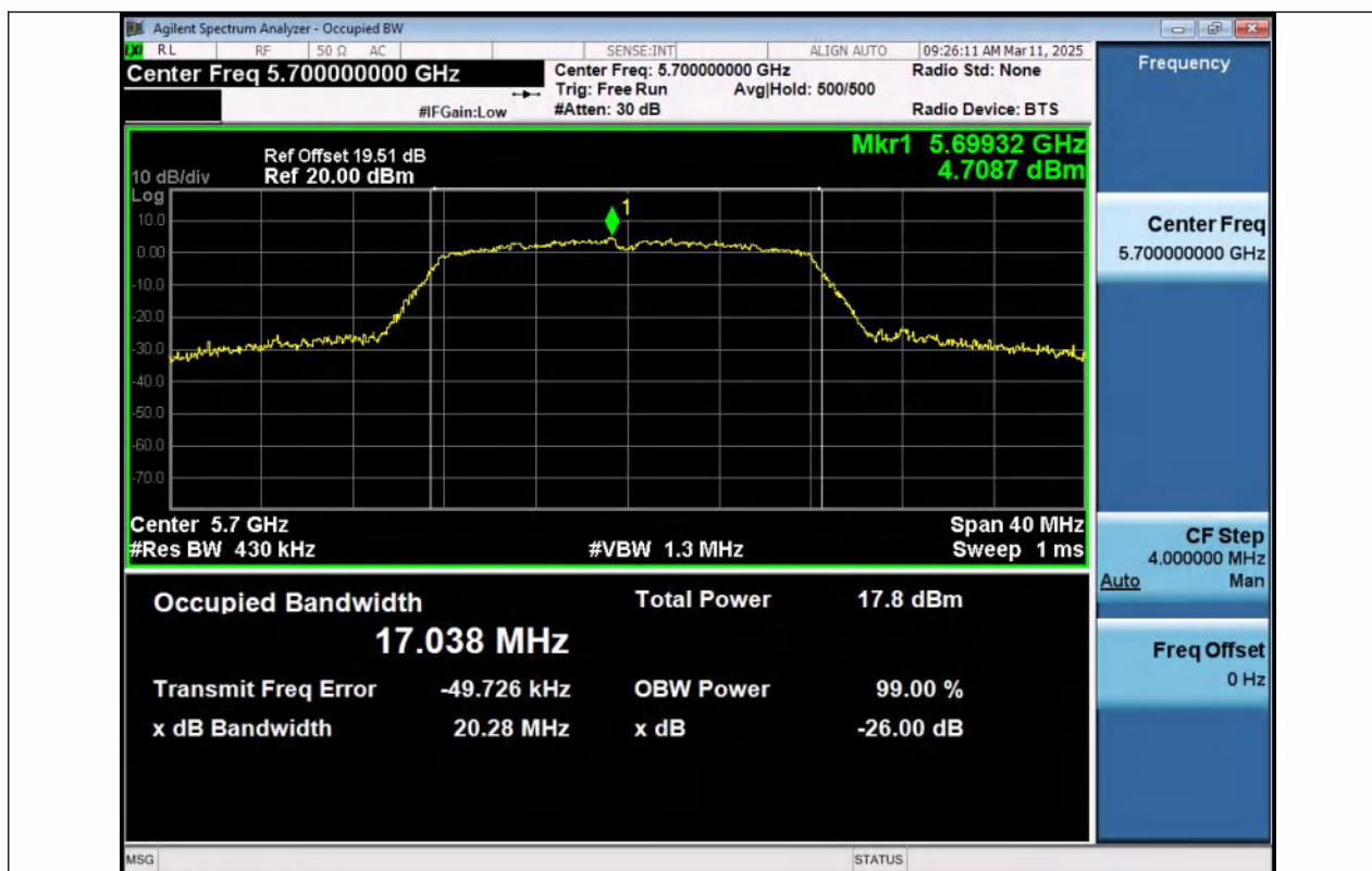
11A-Ant1-5700
