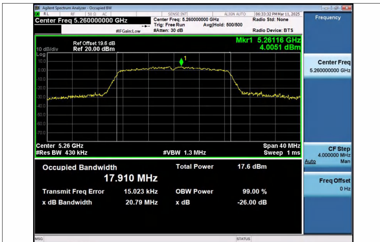
11N20MIMO-Ant1-5260
