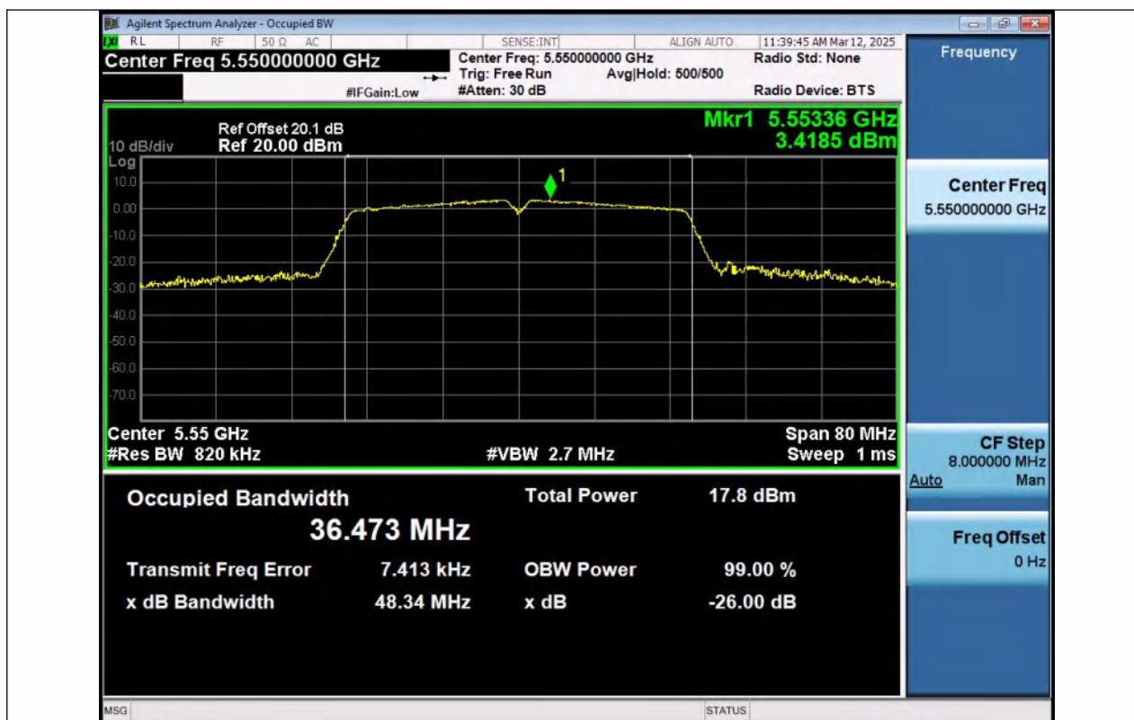
11AC40MIMO-Ant1-5550
