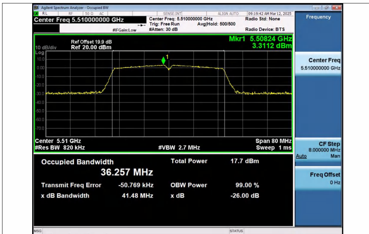
11N40MIMO-Ant1-5510
