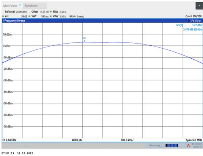
BLE_2M_Ant1_2480
