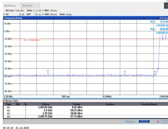
DH5_Ant1_Low_Hop_2402
