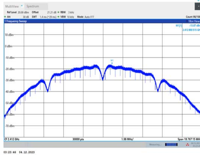
11B_Ant2_2412
