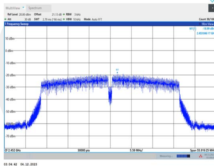
11N40MIMO_Ant2_2452
