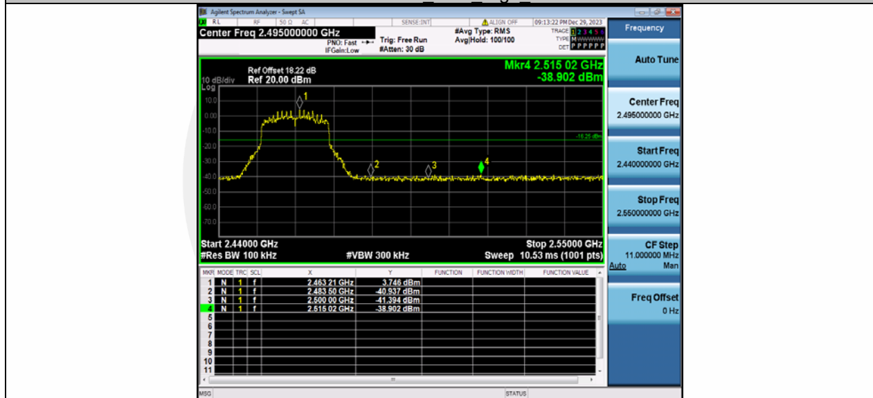
11AX20MIMO_Ant2_High_2462
