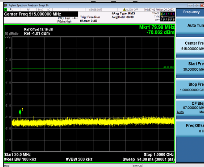
11AX40MIMO Ant2_2452_30~1000
