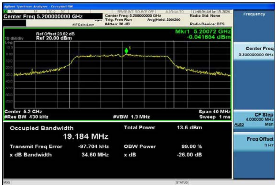
11N20MIMO-Ant1-5200
