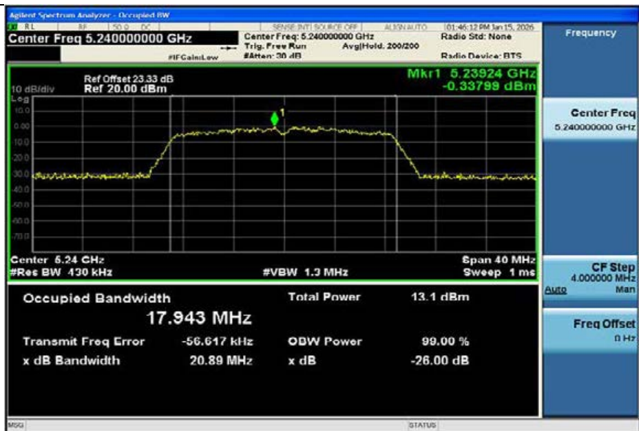
11N20MIMO-Ant1-5240
