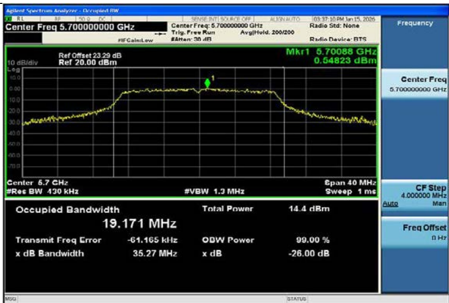
11N20MIMO-Ant1-5700
