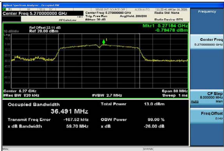
11AC40MIMO-Ant1-5270
