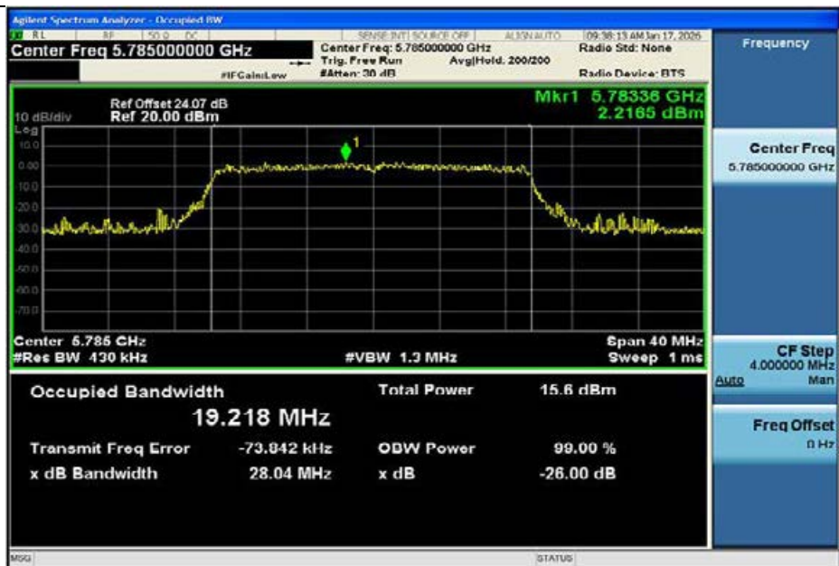
11AX20MIMO-Ant1-5785
