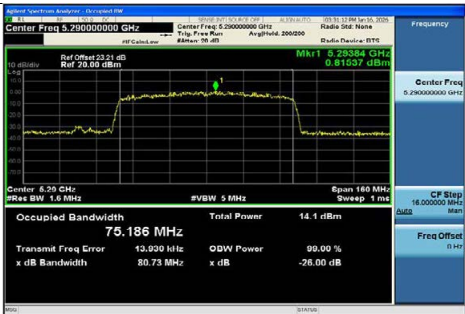
11AC80MIMO-Ant1-5290
