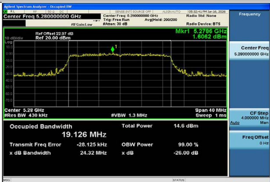
11AX20MIMO-Ant2-5280
