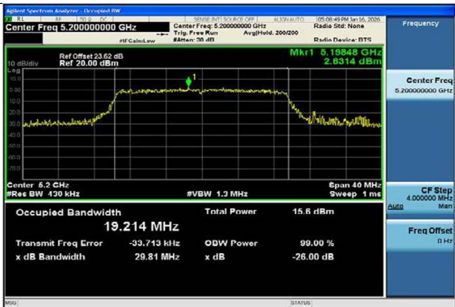
11AX20MIMO-Ant1-5200
