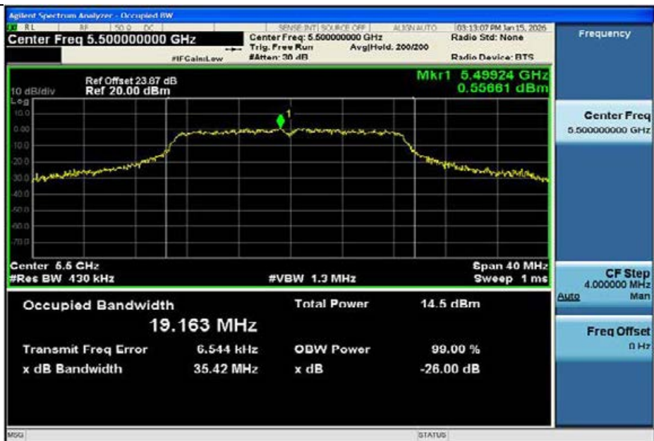
11N20MIMO-Ant1-5500
