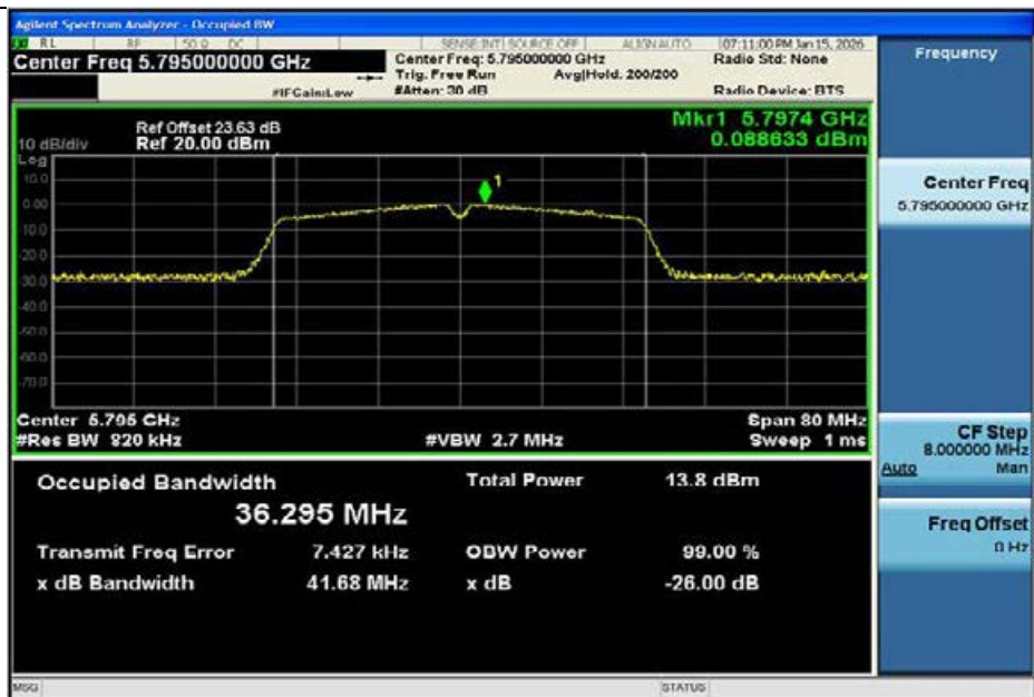
11N40MIMO-Ant1-5795
