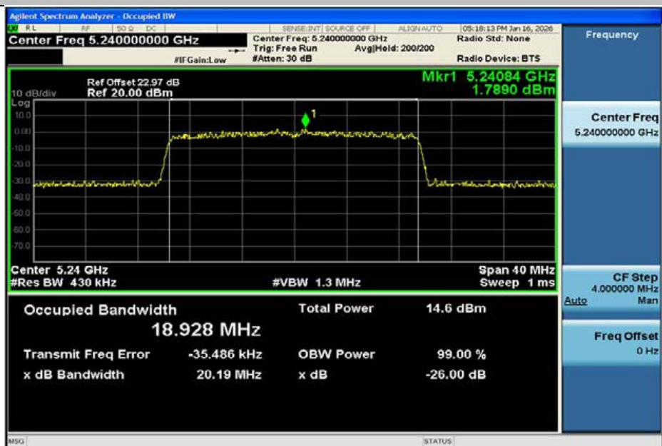
11AX20MIMO-Ant2-5240
