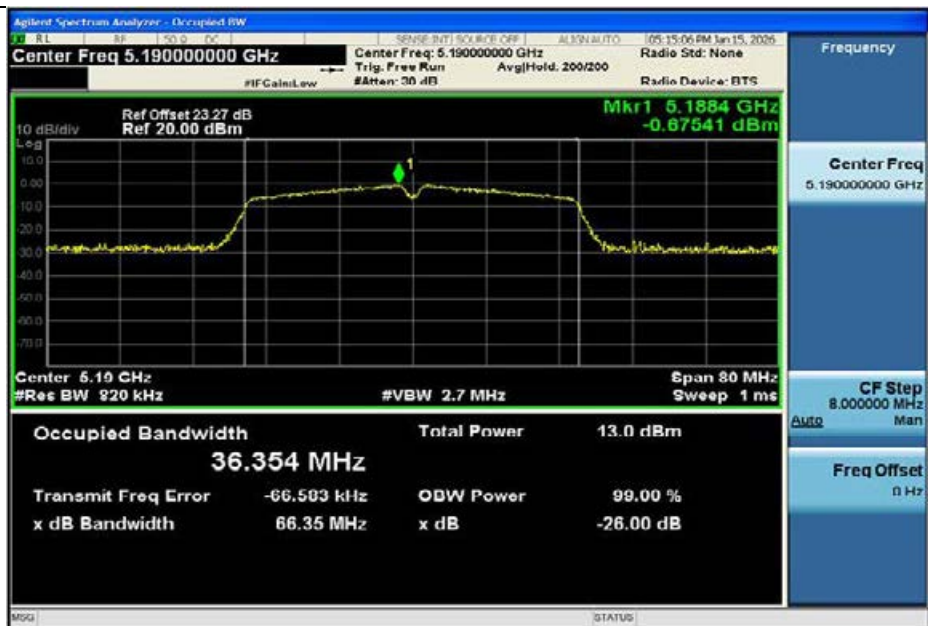
11N40MIMO-Ant1-5190
