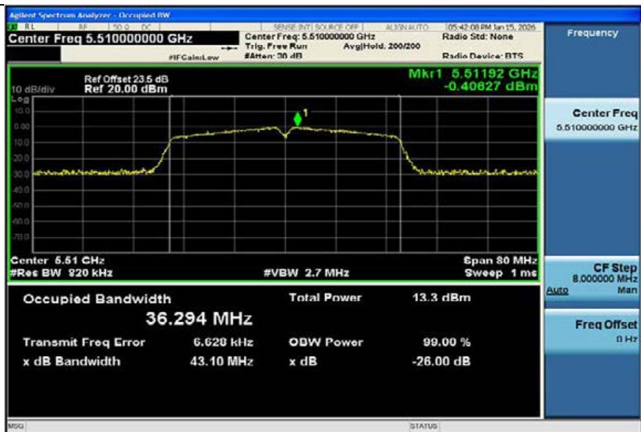
11N40MIMO-Ant1-5510
