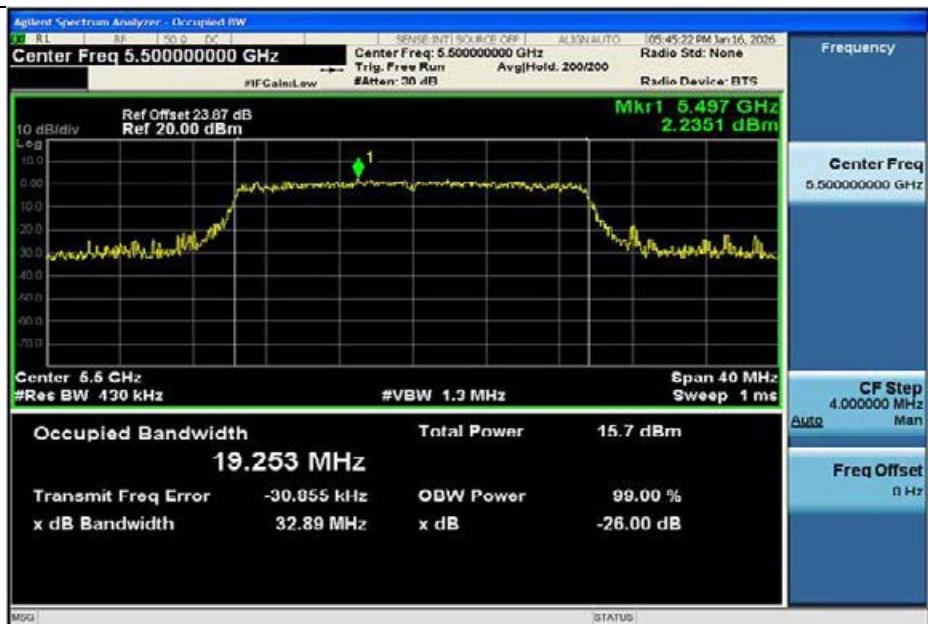
11AX20MIMO-Ant1-5500
