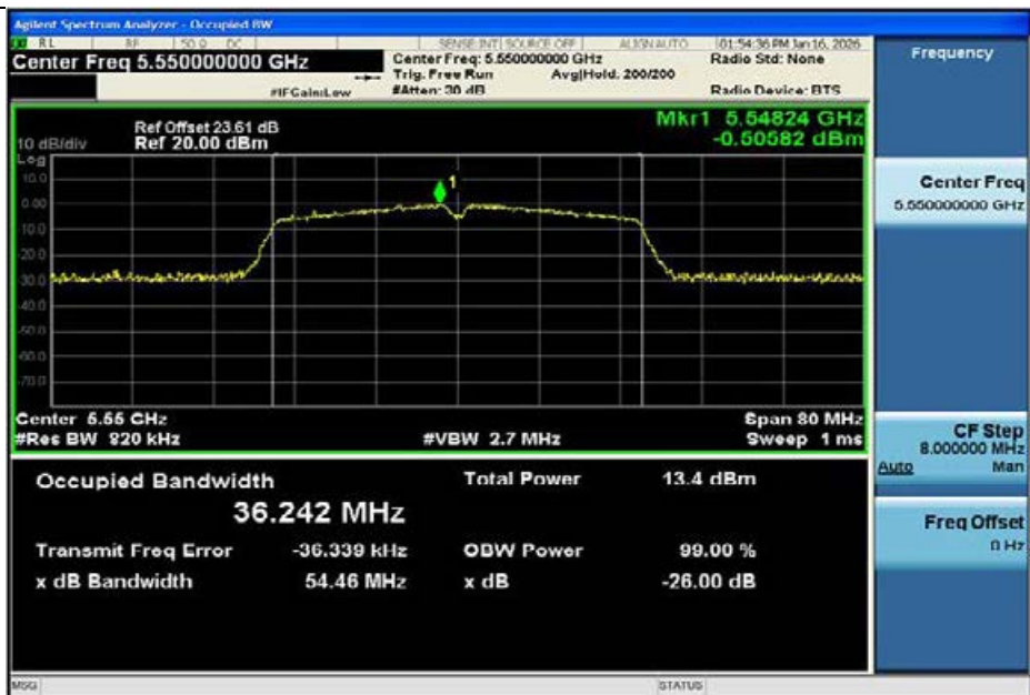
11AC40MIMO-Ant1-5550
