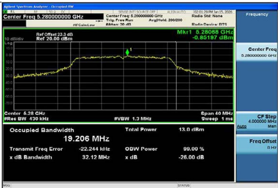
11N20MIMO-Ant1-5280
