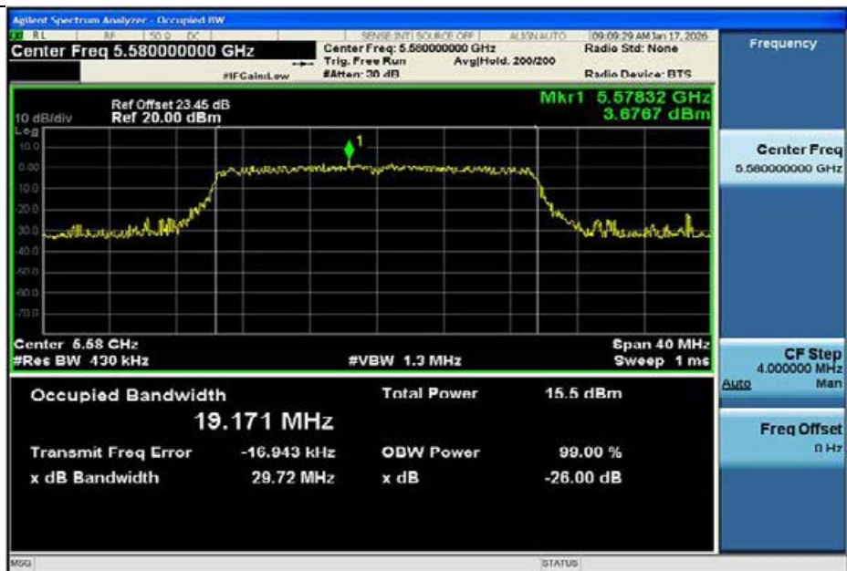
11AX20MIMO-Ant1-5580
