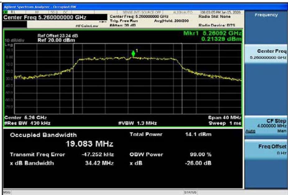
11AC20MIMO-Ant1-5260
