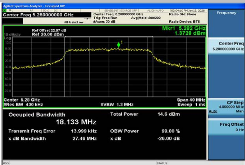
11N20MIMO-Ant2-5280
