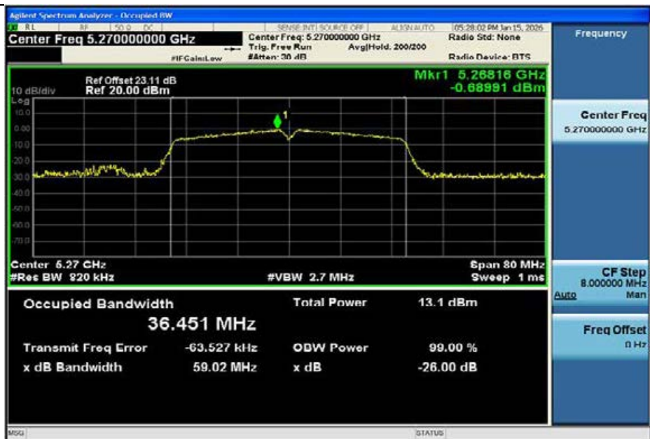
11N40MIMO-Ant1-5270
