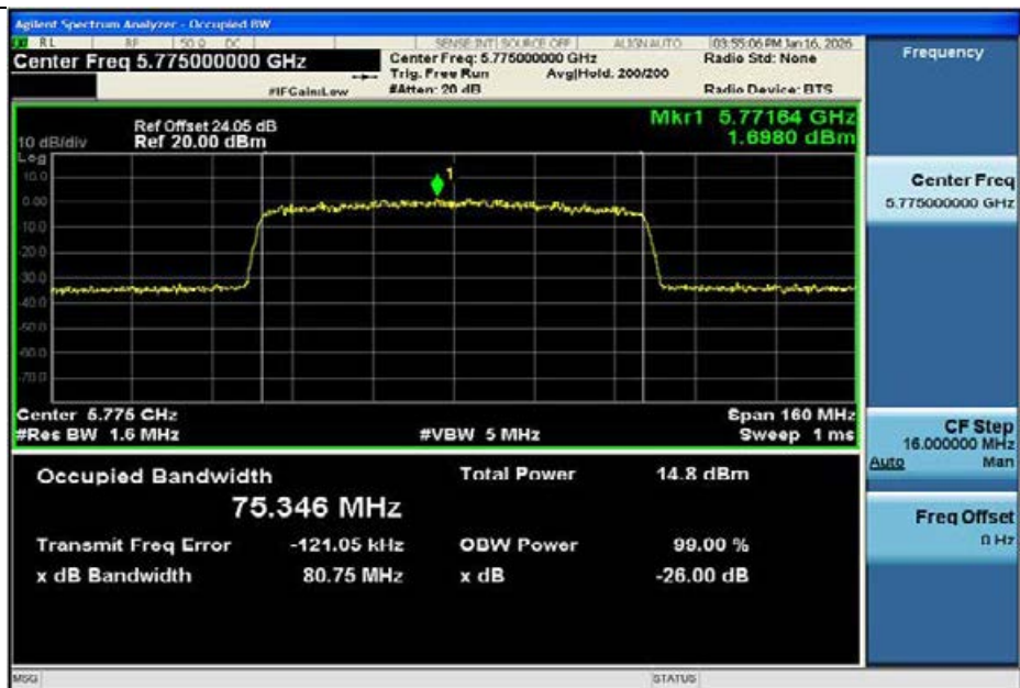
11AC80MIMO-Ant1-5775
