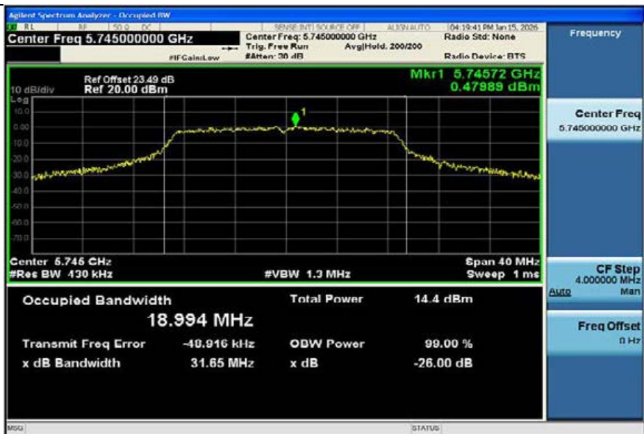
11N20MIMO-Ant1-5745
