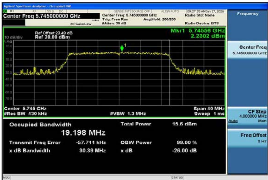
11AX20MIMO-Ant1-5745
