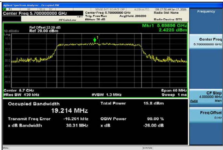
11AX20MIMO-Ant1-5700
