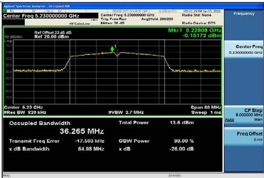
11N40MIMO-Ant1-5230
