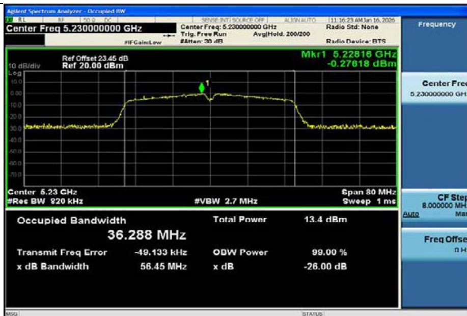
11AC40MIMO-Ant1-5230
