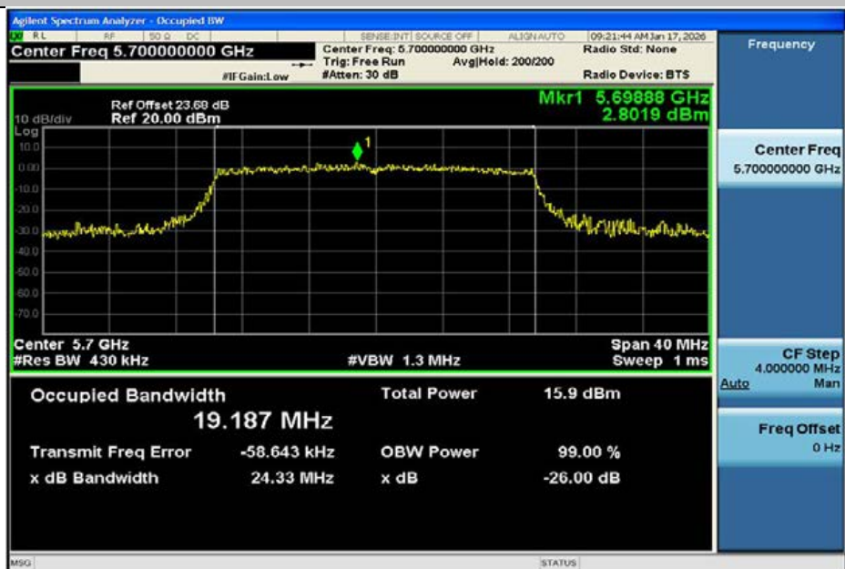
11AX20MIMO-Ant2-5700
