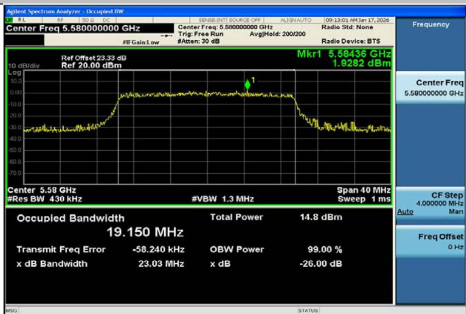
11AX20MIMO-Ant2-5580
