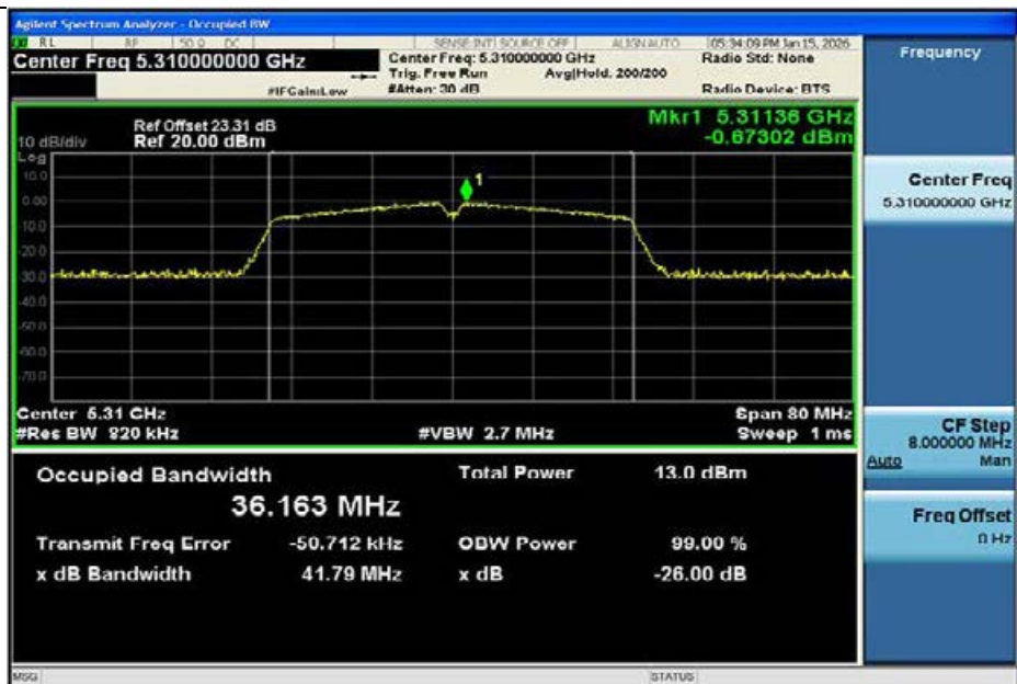
11N40MIMO-Ant1-5310
