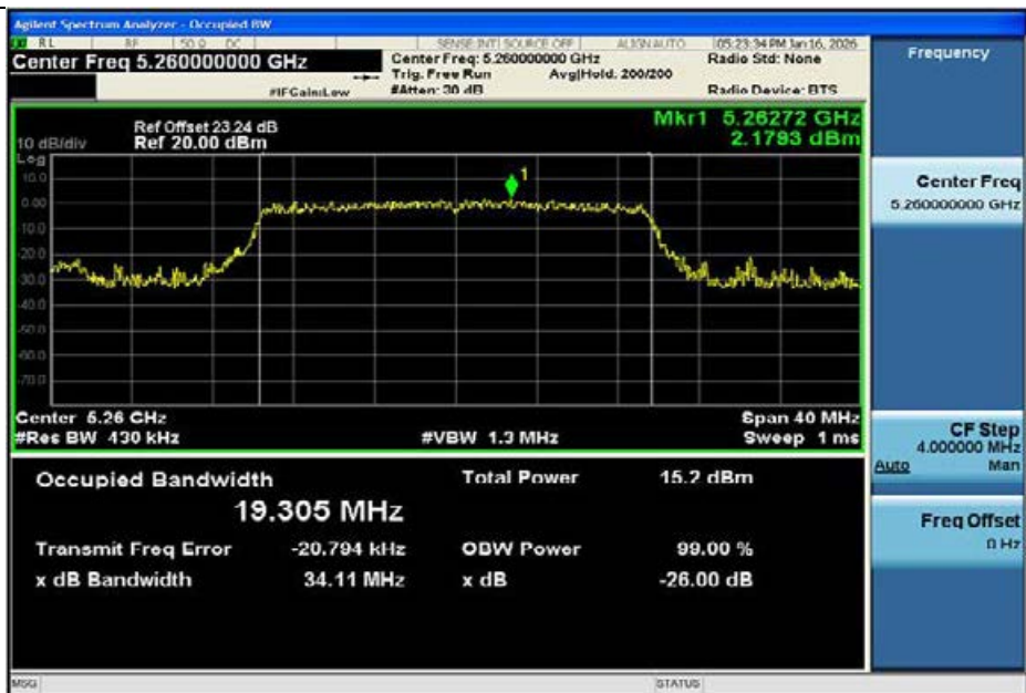
11AX20MIMO-Ant1-5260
