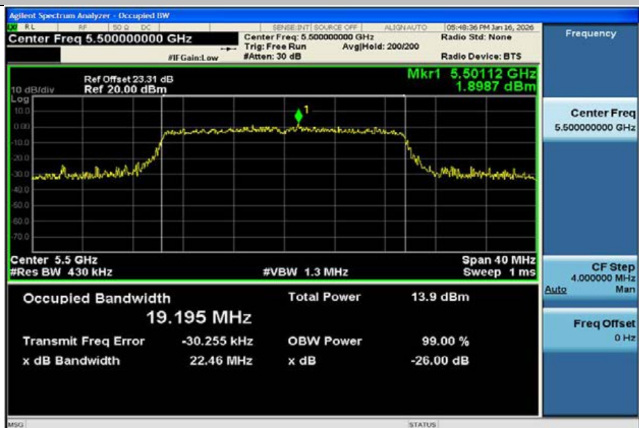
11AX20MIMO-Ant2-5500
