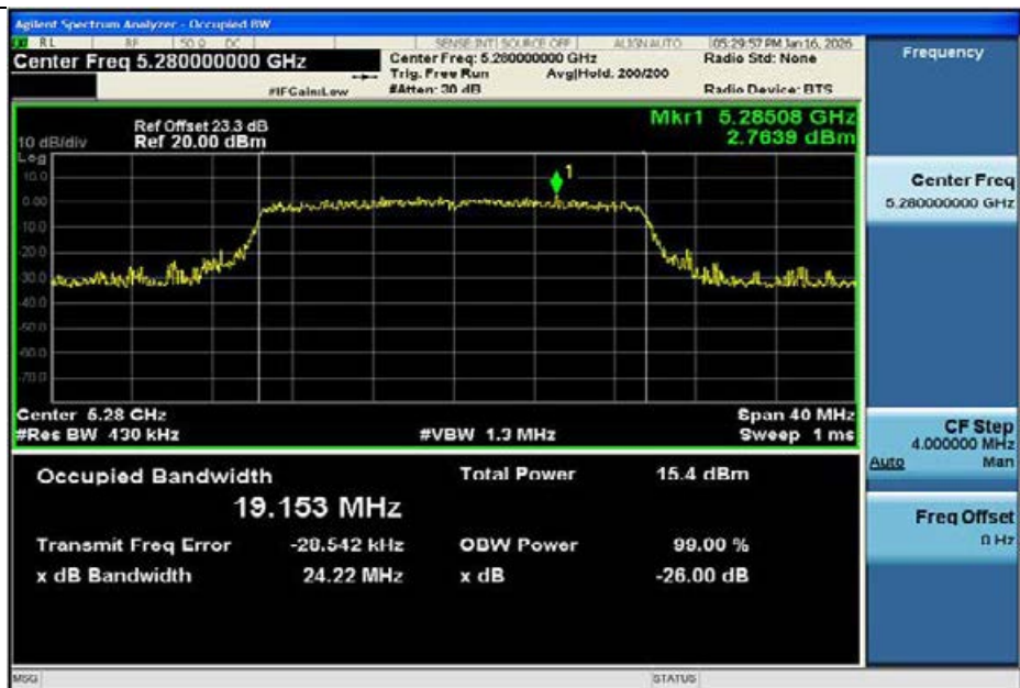
11AX20MIMO-Ant1-5280
