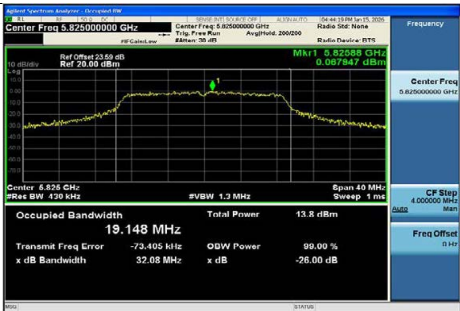
11N20MIMO-Ant1-5825
