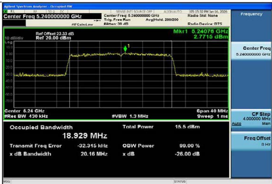
11AX20MIMO-Ant1-5240
