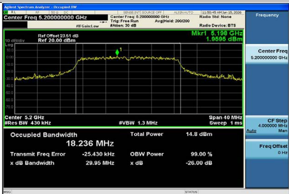
11N20MIMO-Ant2-5200
