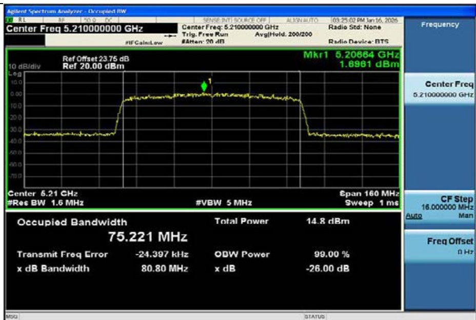
11AC80MIMO-Ant1-5210
