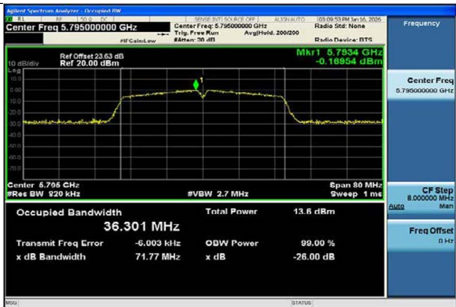
11AC40MIMO-Ant1-5795
