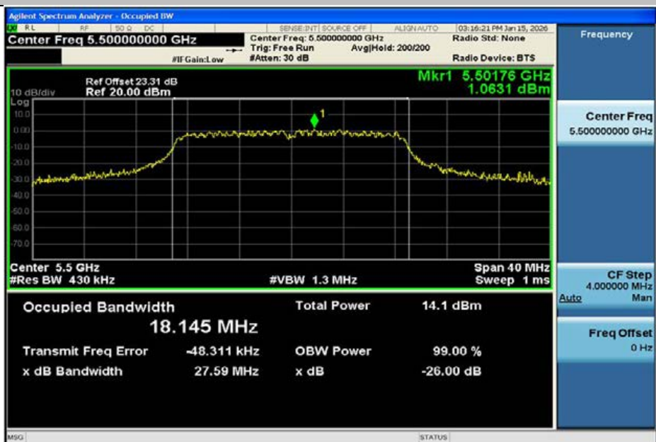
11N20MIMO-Ant2-5500
