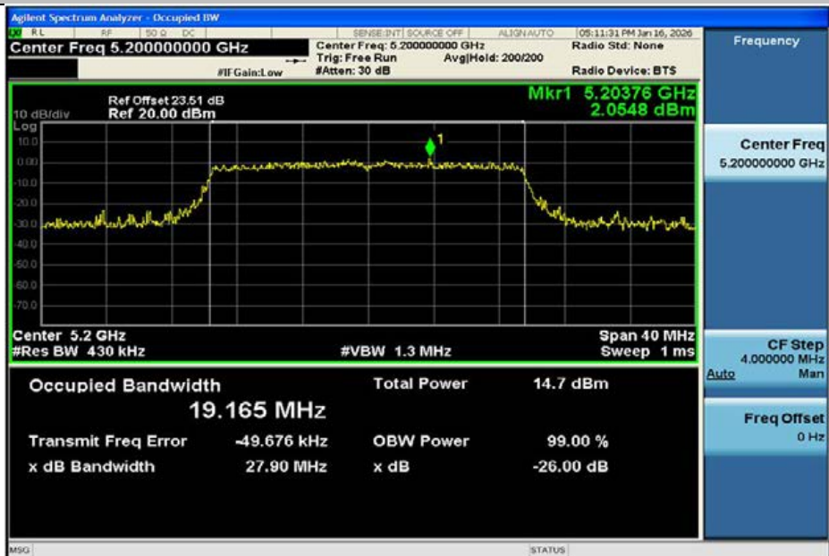
11AX20MIMO-Ant2-5200
