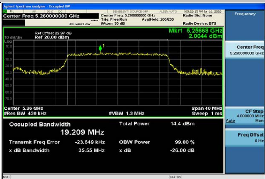
11AX20MIMO-Ant2-5260
