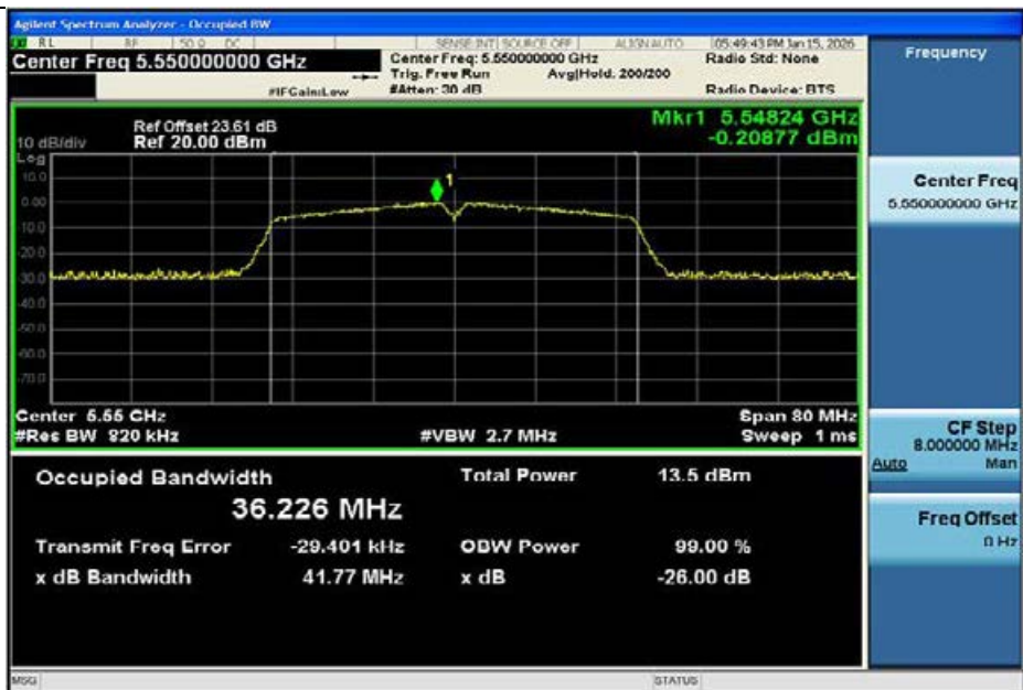
11N40MIMO-Ant1-5550
