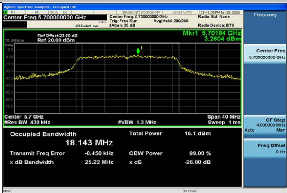
11N20MIMO-Ant2-5700
