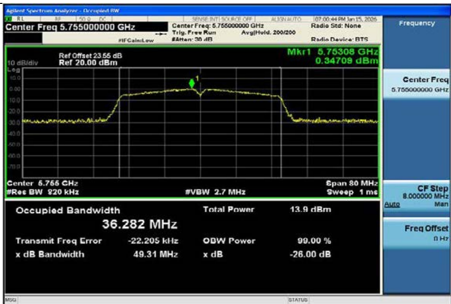
11N40MIMO-Ant1-5755
