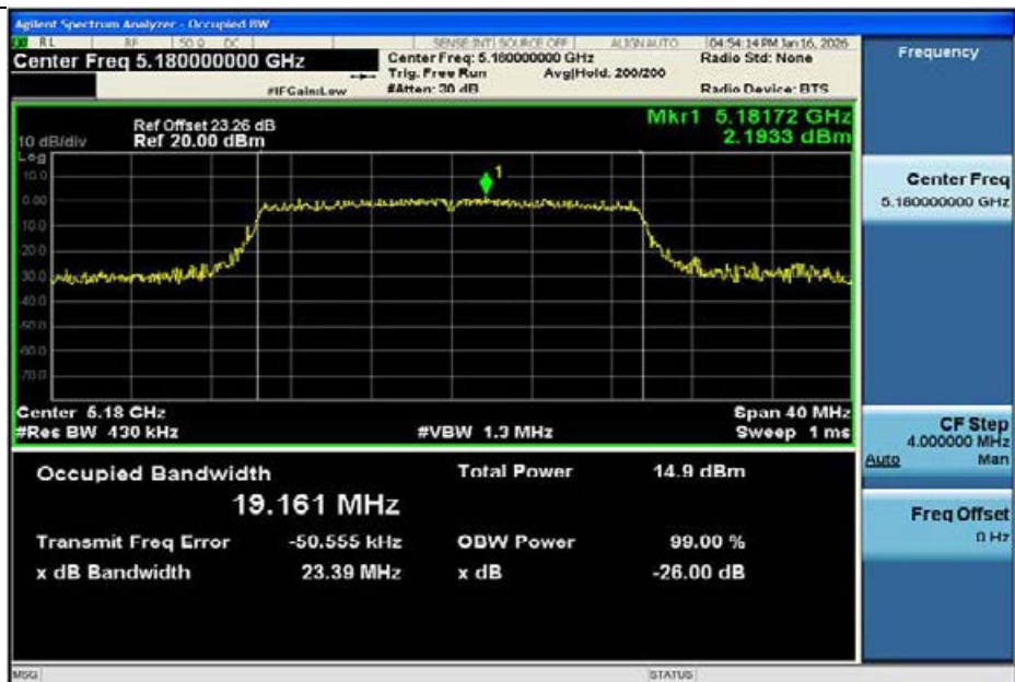
11AX20MIMO-Ant1-5180
