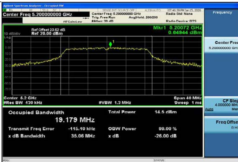
11AC20MIMO-Ant1-5200
