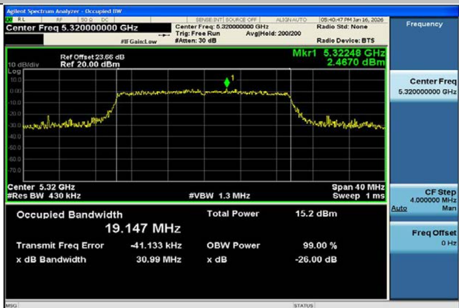
11AX20MIMO-Ant2-5320
