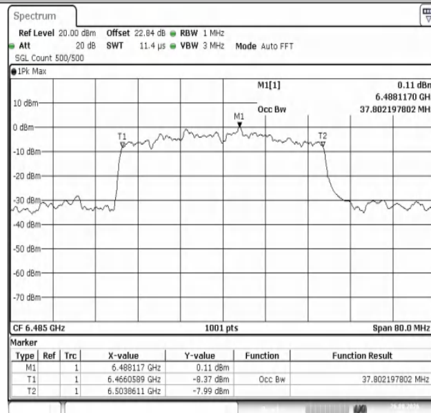
11AX40MIMO-Ant1-6485-PASS
