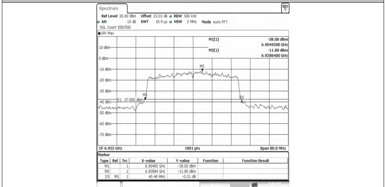
11AX40MIMO-Ant1-6925
