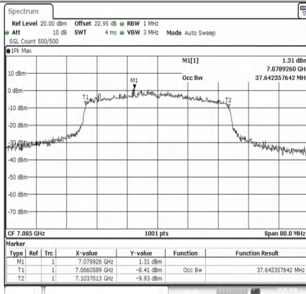
11AX40MIMO-Ant1-7085-PASS
