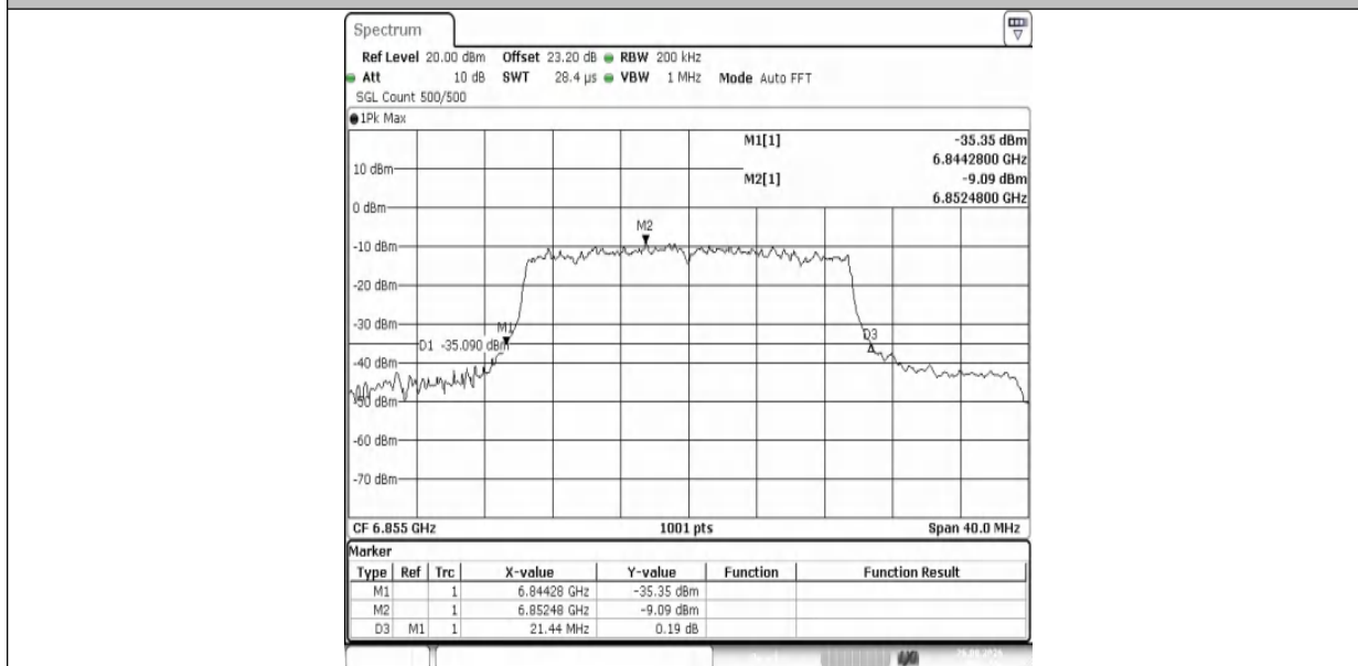
11AX20MIMO-Ant1-6855
