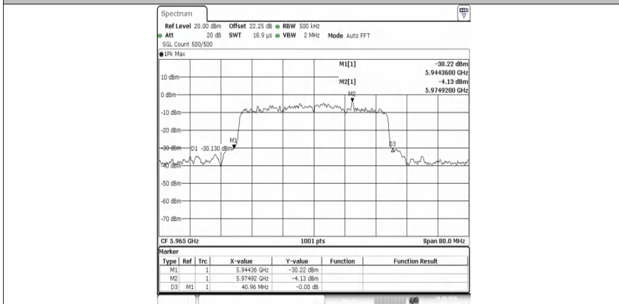
11AX40MIMO-Ant1-5965
