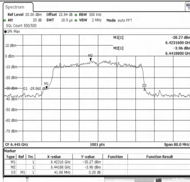
11AX40MIMO-Ant1-6445
