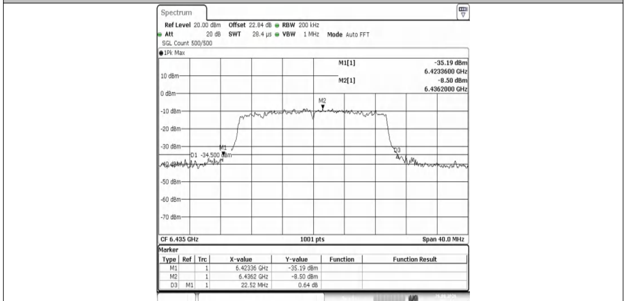
11AX20MIMO-Ant1-6435
