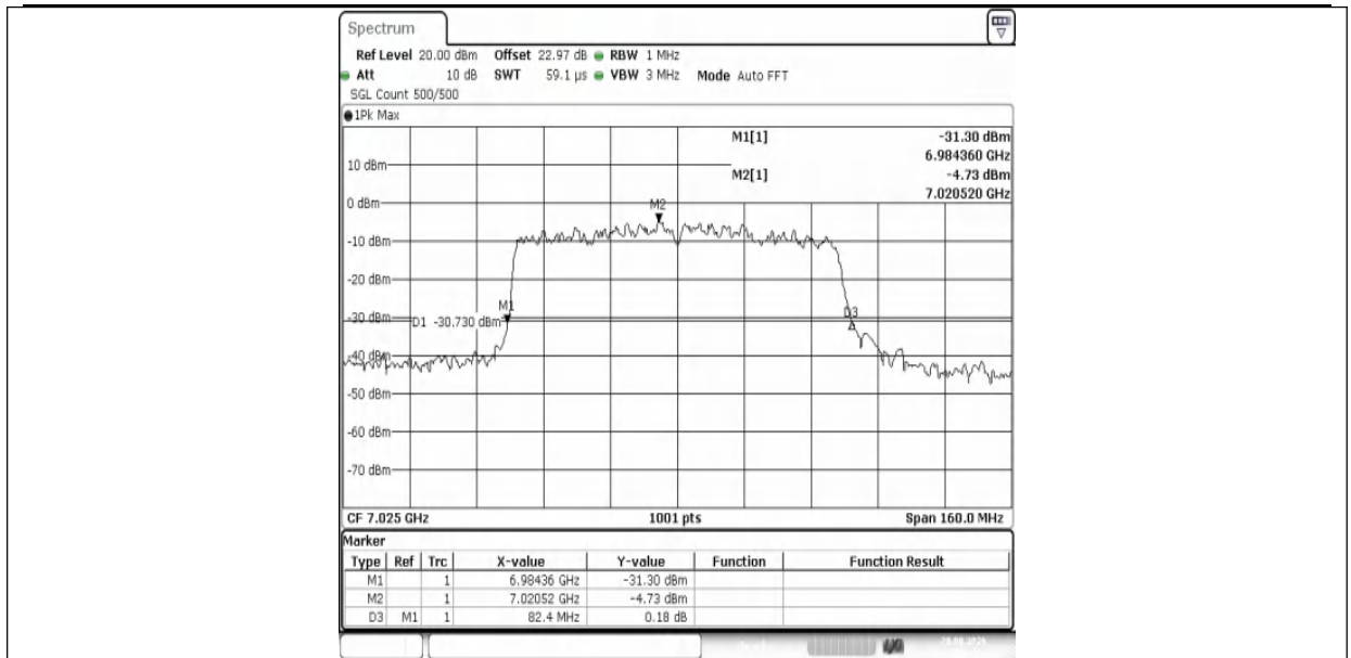
11AX80MIMO-Ant1-7025
