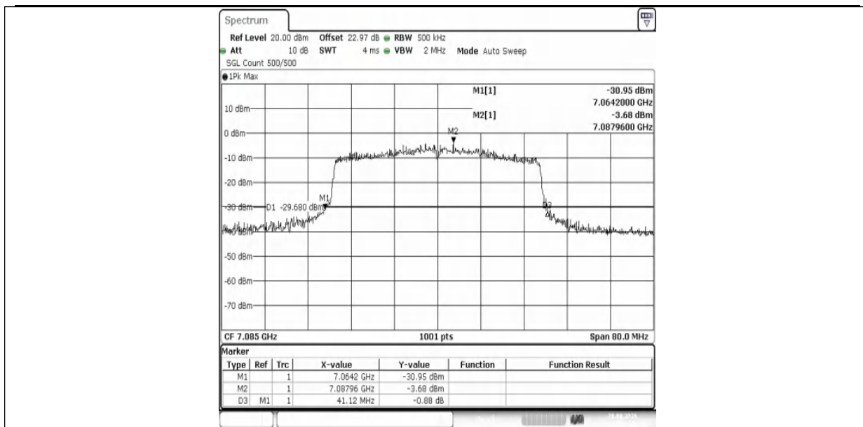
11AX40MIMO-Ant1-7085
