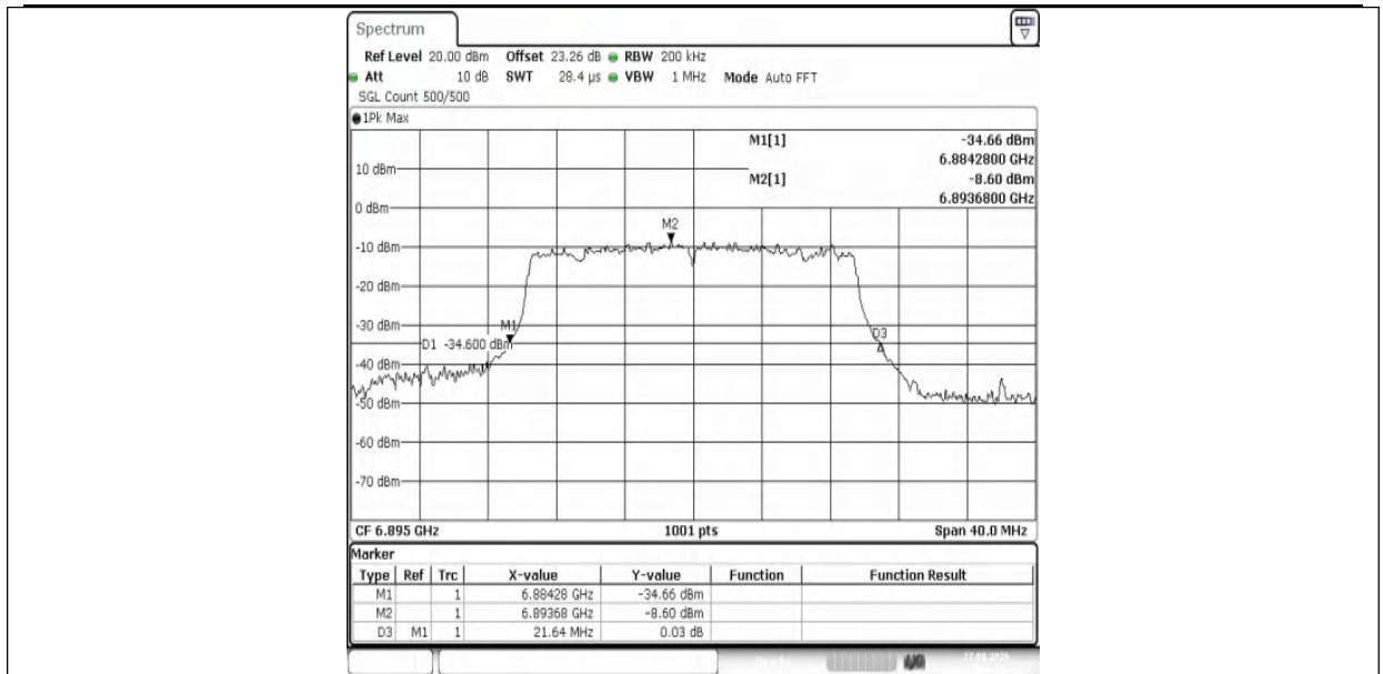
11AX20MIMO-Ant1-6895
