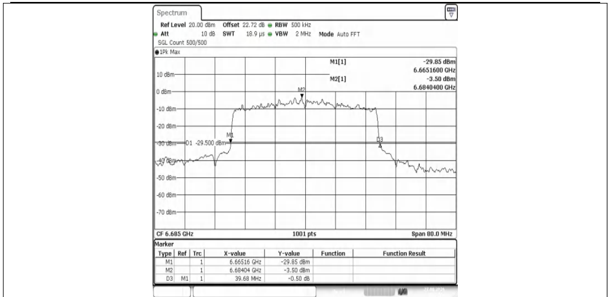
11AX40MIMO-Ant1-6685
