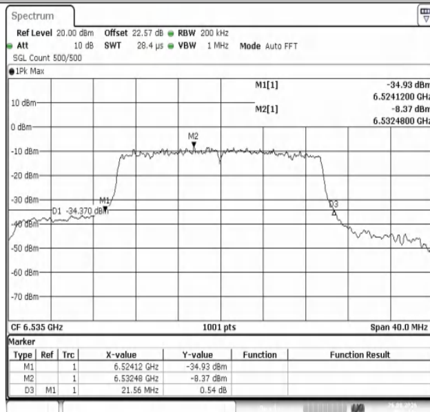
11AX20MIMO-Ant1-6535
