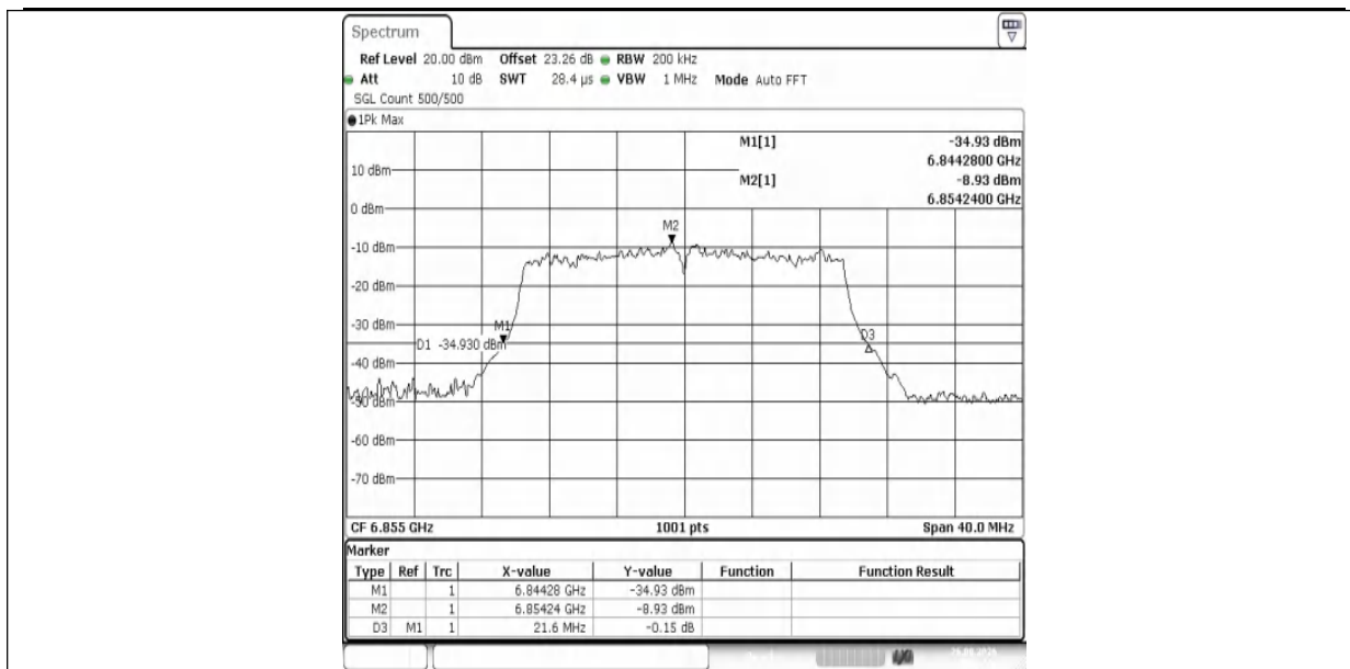
11AX20MIMO-Ant1-6855
