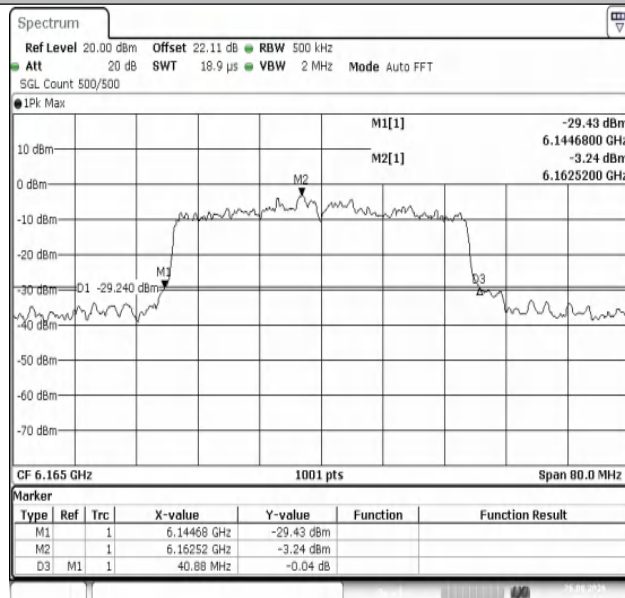
11AX40MIMO-Ant1-6165
