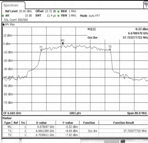
11AX40MIMO-Ant1-6685-PASS
