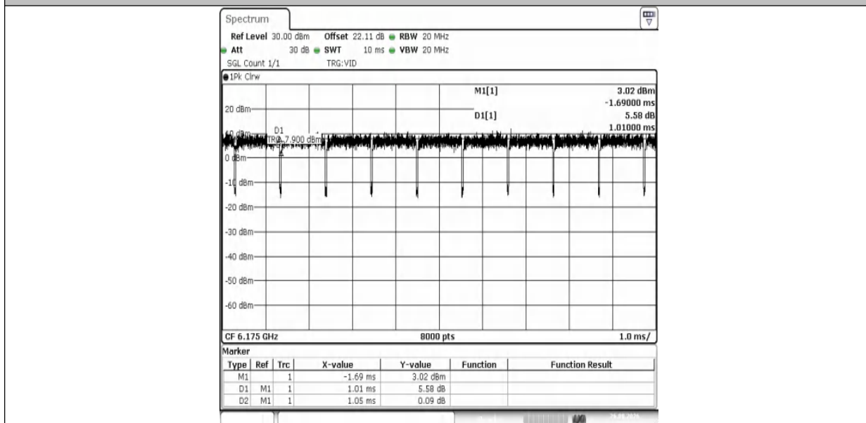
NTNV-11AX20MIMO-Ant1-6175
