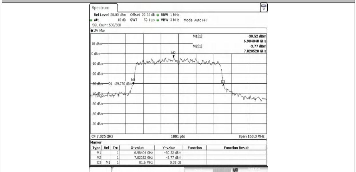
11AX80MIMO-Ant1-7025
