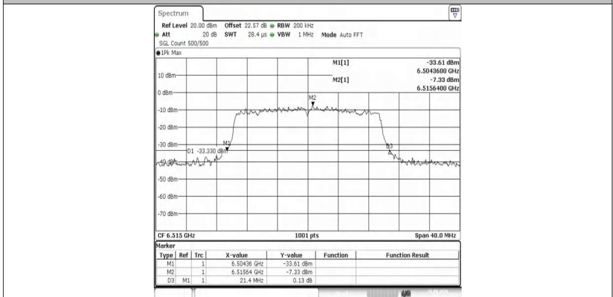
11AX20MIMO-Ant1-6515
