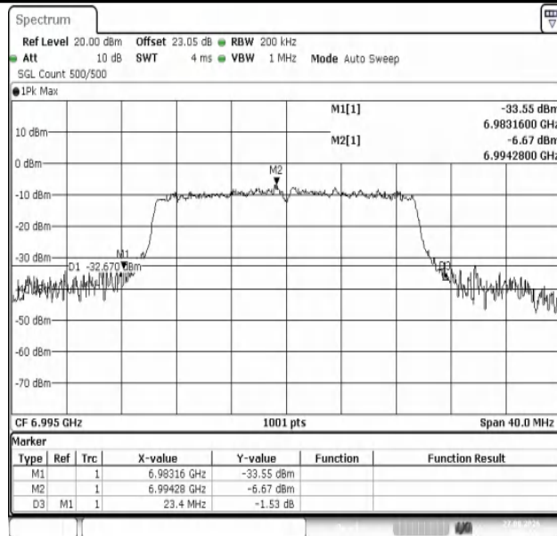
11AX20MIMO-Ant1-6995
