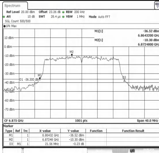
11AX20MIMO-Ant1-6875
