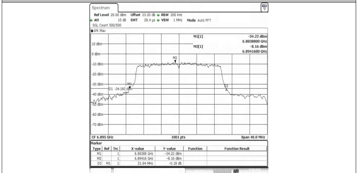
11AX20MIMO-Ant1-6895
