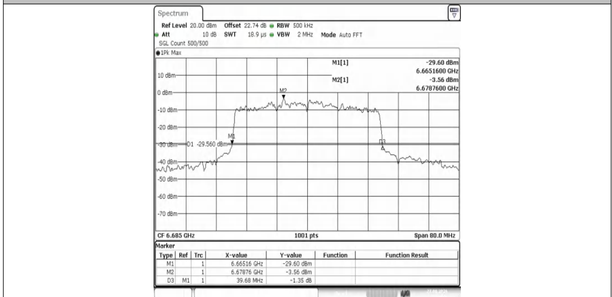
11AX40MIMO-Ant1-6685
