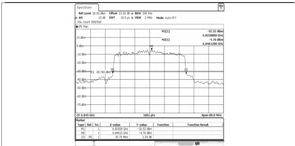
11AX40MIMO-Ant1-6845
