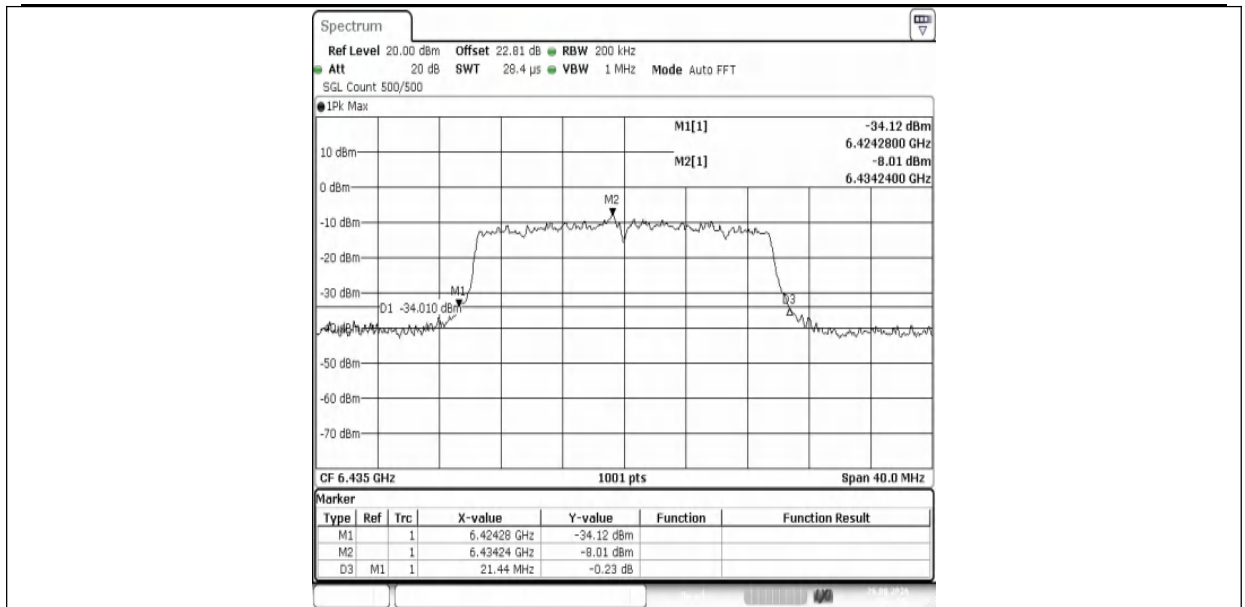
11AX20MIMO-Ant1-6435
