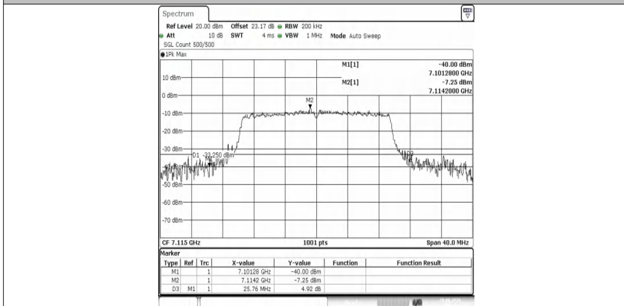
11AX20MIMO-Ant1-7115
