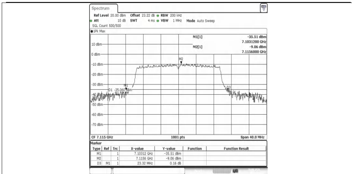
11AX20MIMO-Ant1-7115
