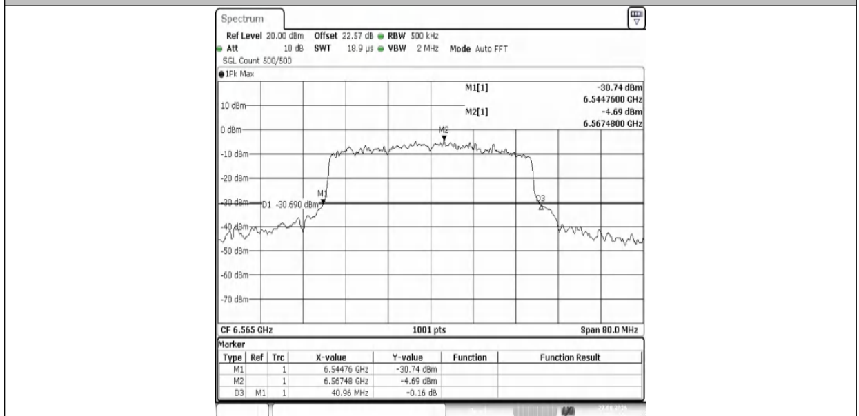
11AX40MIMO-Ant1-6565
