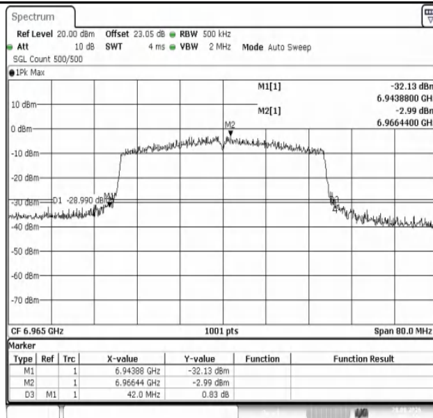
11AX40MIMO-Ant1-6965
