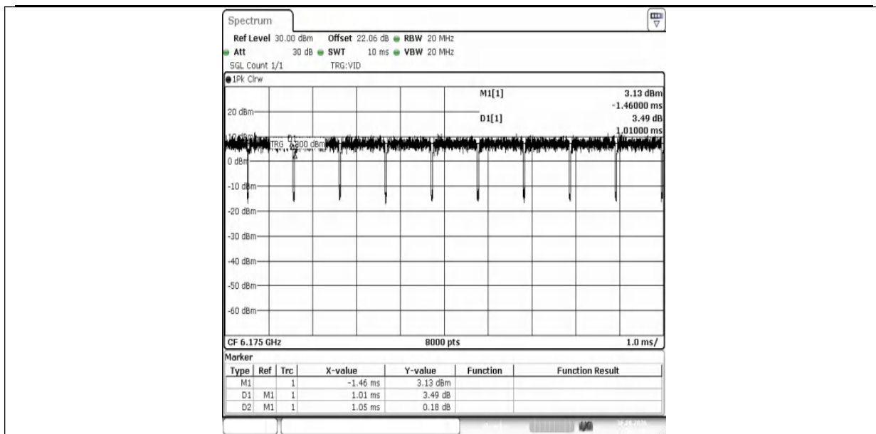
NTNV-11AX20MIMO-Ant1-6175
