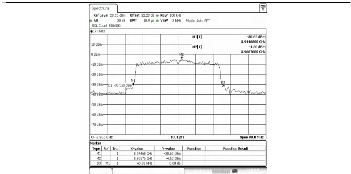
11AX40MIMO-Ant1-5965
