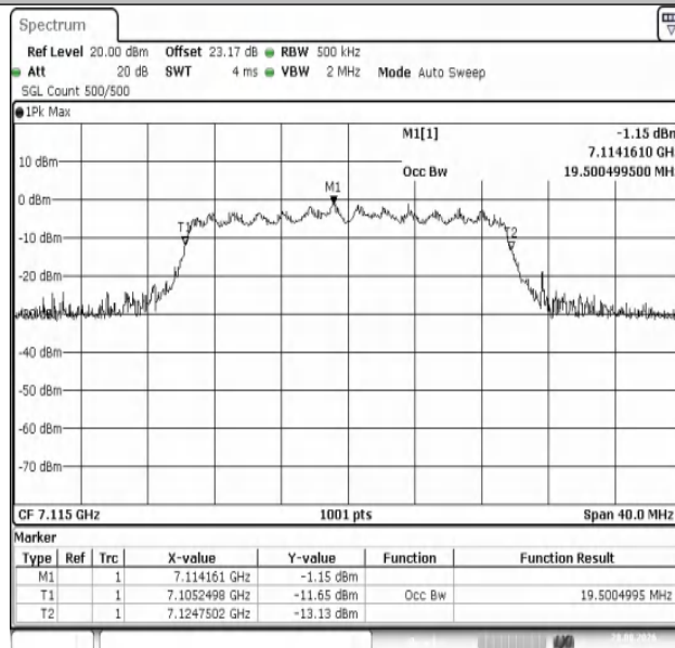
11AX20MIMO-Ant1-7115-PASS
