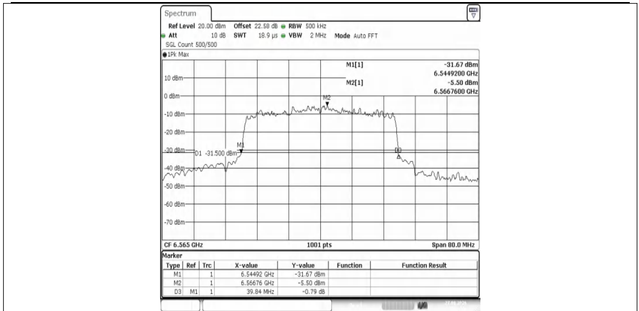
11AX40MIMO-Ant1-6565
