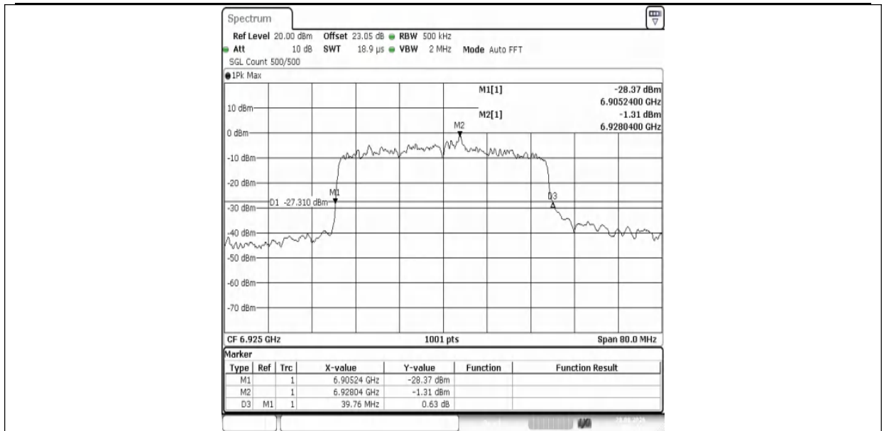
11AX40MIMO-Ant1-6925
