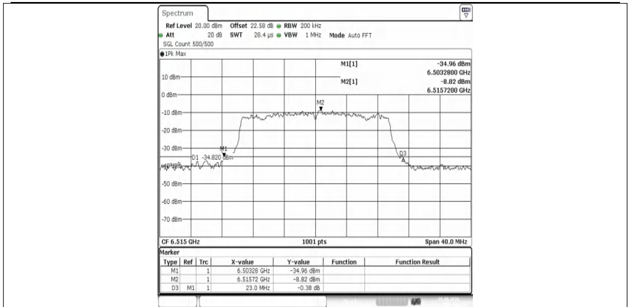
11AX20MIMO-Ant1-6515
