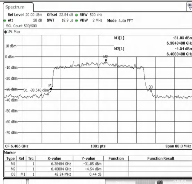
11AX40MIMO-Ant1-6405
