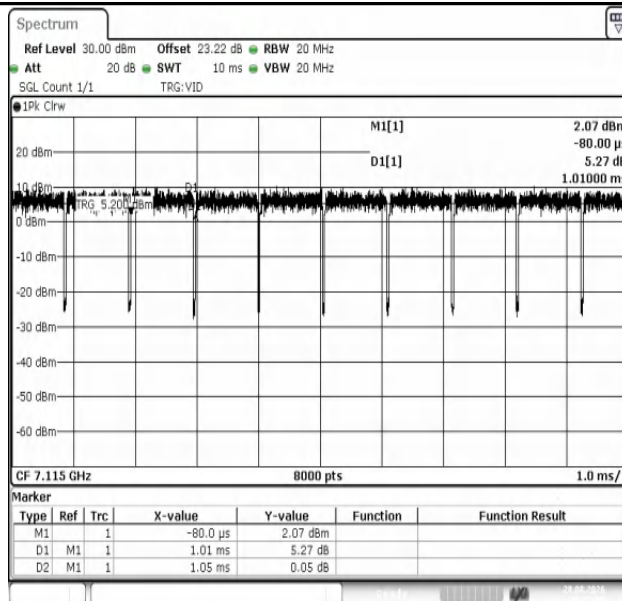
NTNV-11AX20MIMO-Ant1-7115
