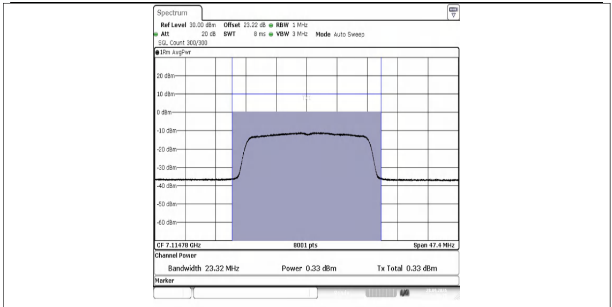
11AX20MIMO-Ant1-7115-PASS
