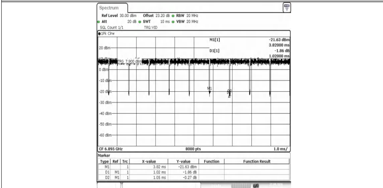
NTNV-11AX20MIMO-Ant1-6895
