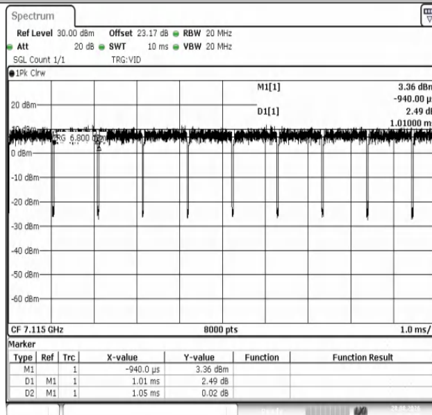
NTNV-11AX20MIMO-Ant2-7115
