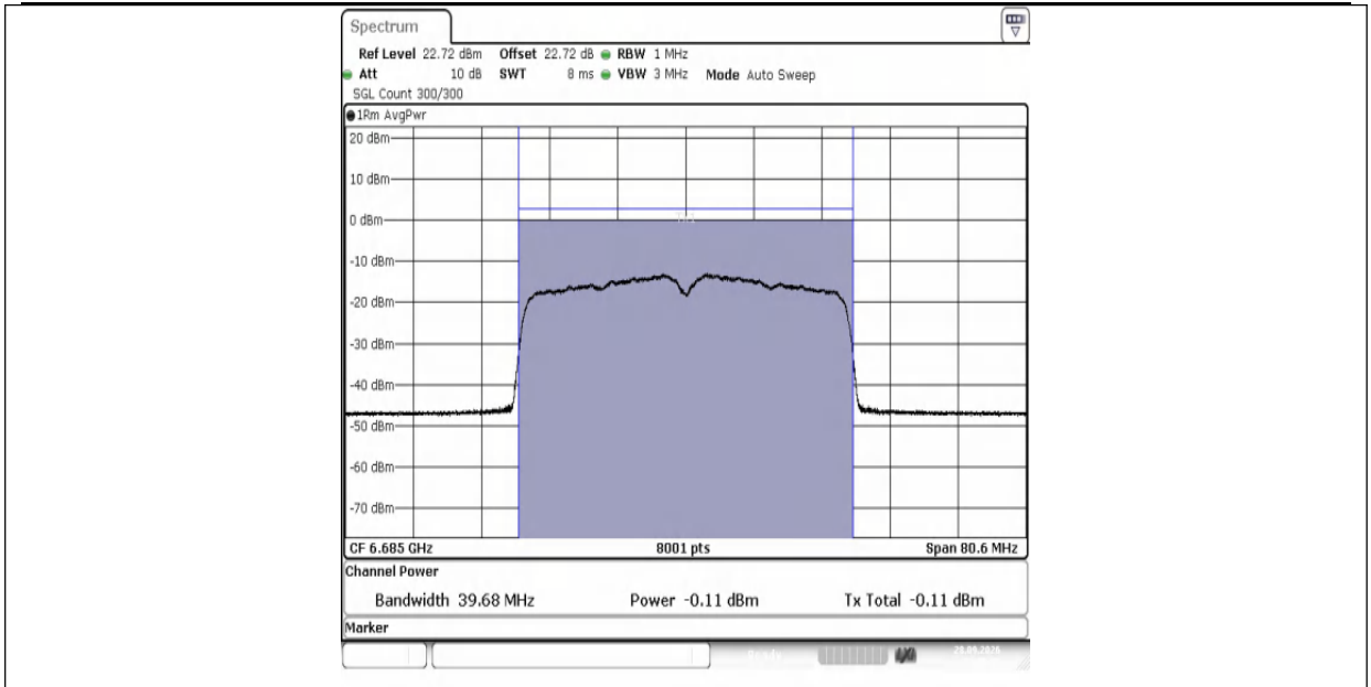
11AX40MIMO-Ant1-6685-PASS
