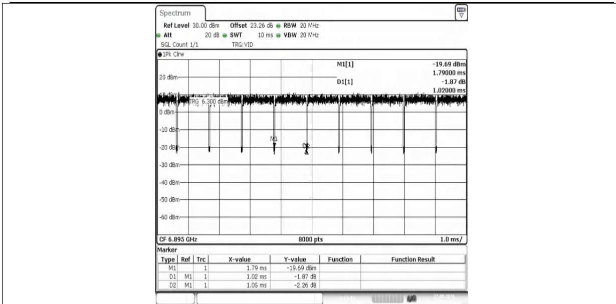
NTNV-11AX20MIMO-Ant1-6895
