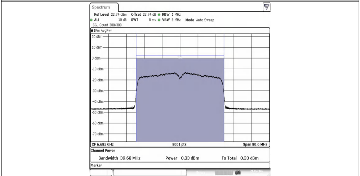
11AX40MIMO-Ant1-6685-PASS
