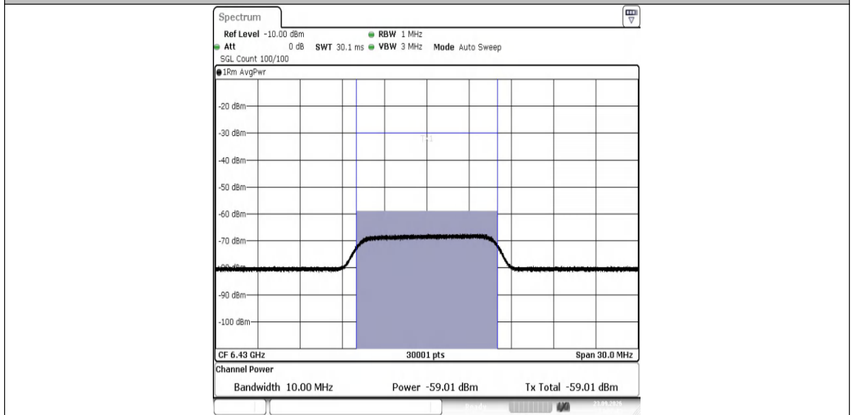
11AX80SISO-Ant1-6465-6430-PASS
