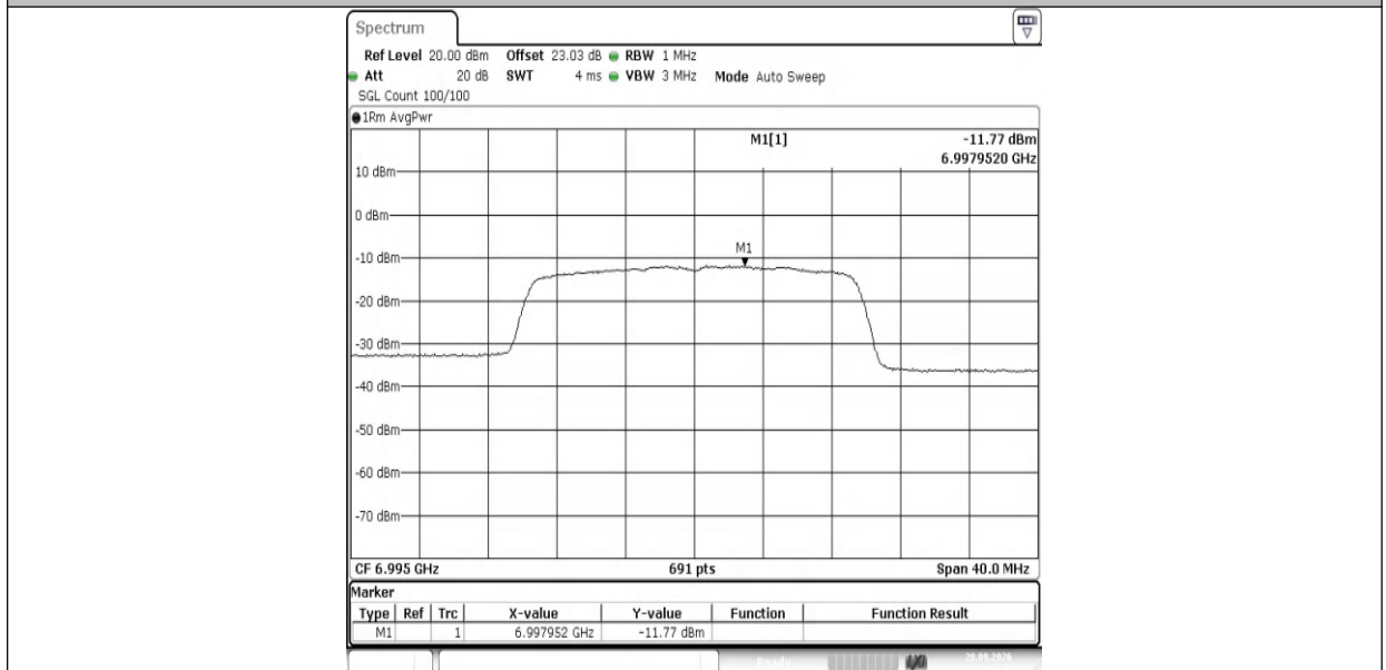
11AX20MIMO-Ant1-6995-PASS
