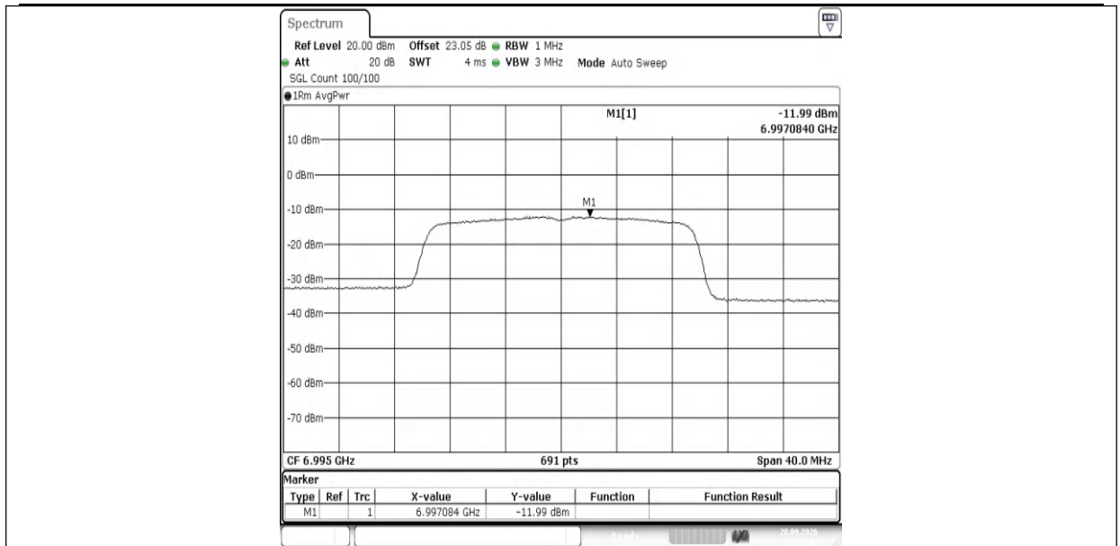
11AX20MIMO-Ant1-6995-PASS
