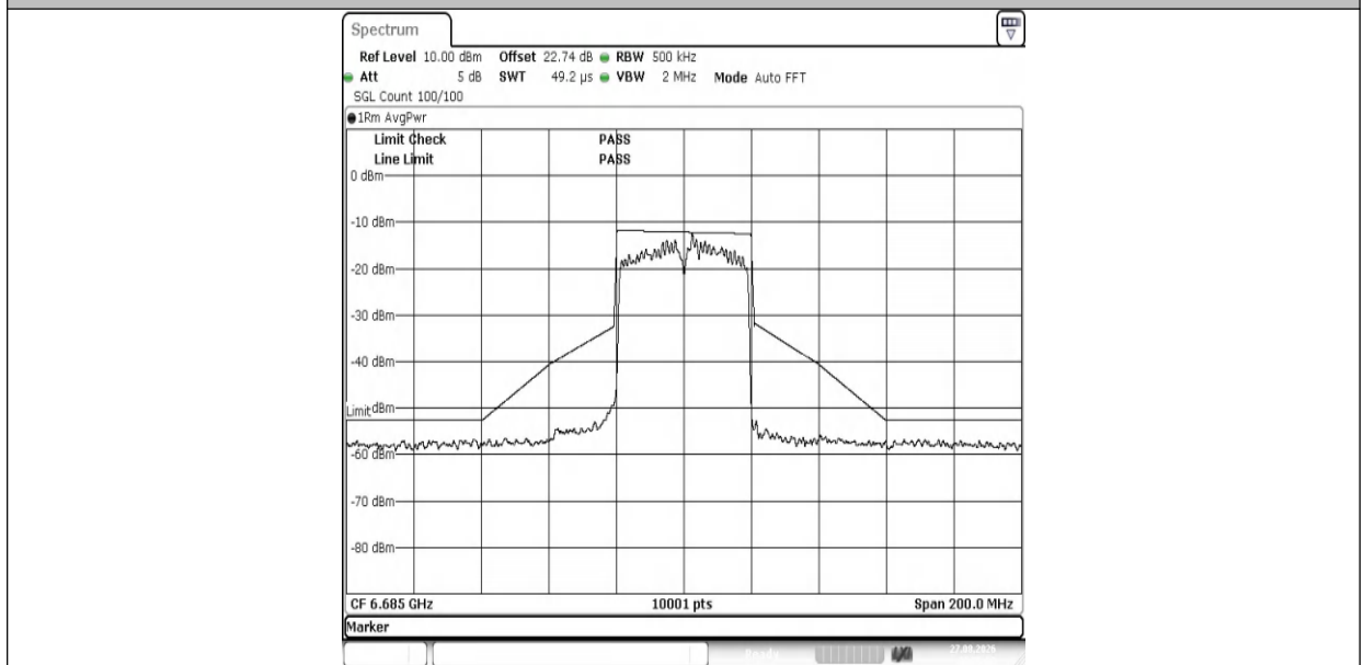
NTNV-11AX40MIMO-Ant1-6685-PASS
