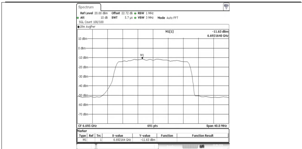
11AX20MIMO-Ant1-6695-PASS
