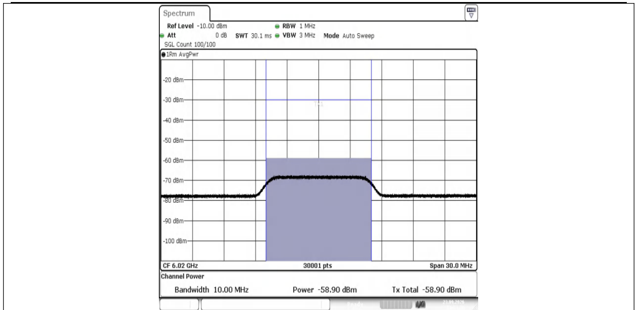
11AX80SISO-Ant1-5985-6020-PASS
