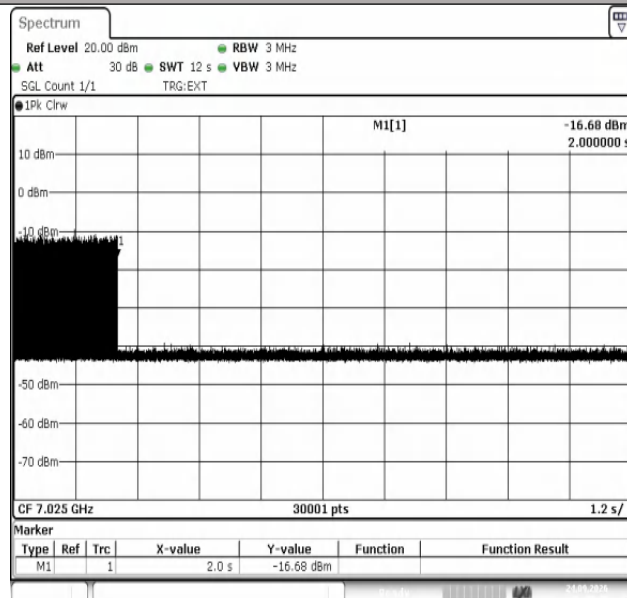
11AX80SISO-Ant1-7025-7025-3-PASS
