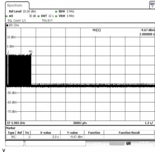
11AX80SISO-Ant1-5985-5985-1-PASS
