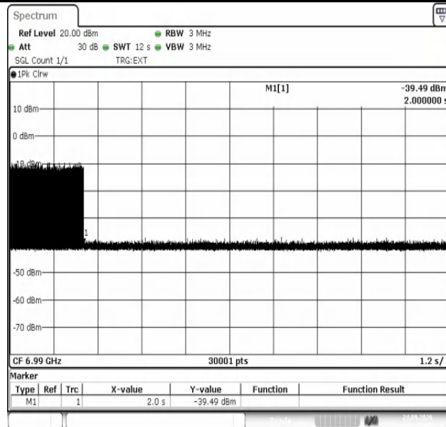
11AX80SISO-Ant1-7025-6990-7-PASS
