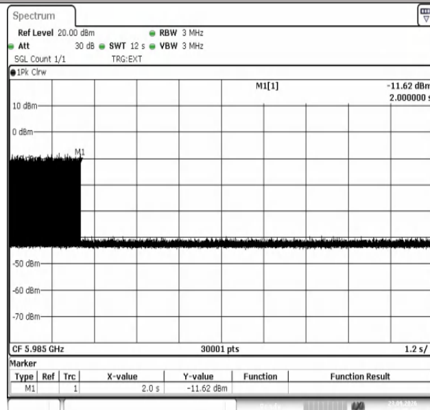
11AX80SISO-Ant1-5985-5985-7-PASS
