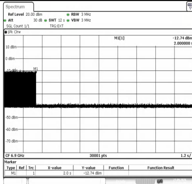
11AX80SISO-Ant1-6865-6900-7-PASS
