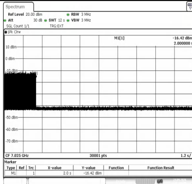
11AX80SISO-Ant1-7025-7025-5-PASS
