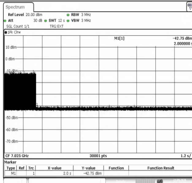
11AX80SISO-Ant1-7025-7025-1-PASS
