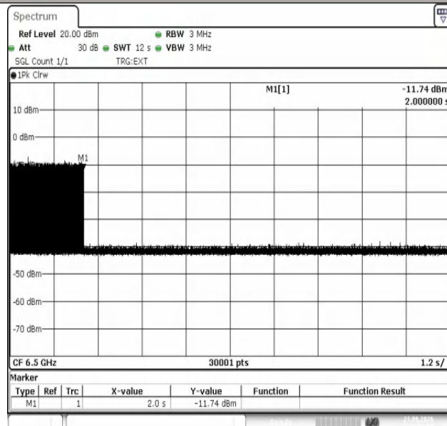
11AX80SISO-Ant1-6465-6500-3-PASS
