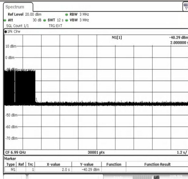
11AX80SISO-Ant1-7025-6990-5-PASS
