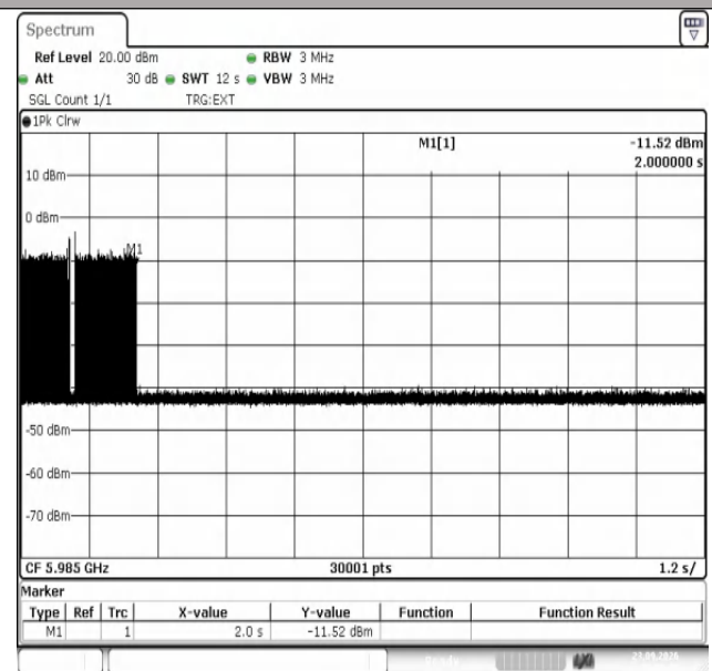
11AX80SISO-Ant1-5985-5985-2-PASS
