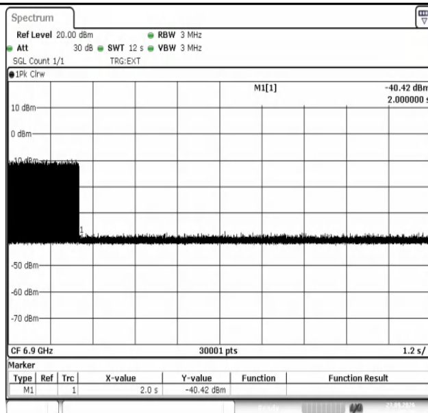
11AX80SISO-Ant1-6865-6900-1-PASS
