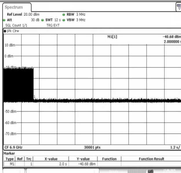
11AX80SISO-Ant1-6865-6900-1-PASS
