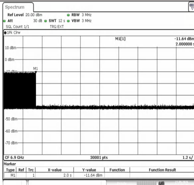
11AX80SISO-Ant1-6865-6900-3-PASS
