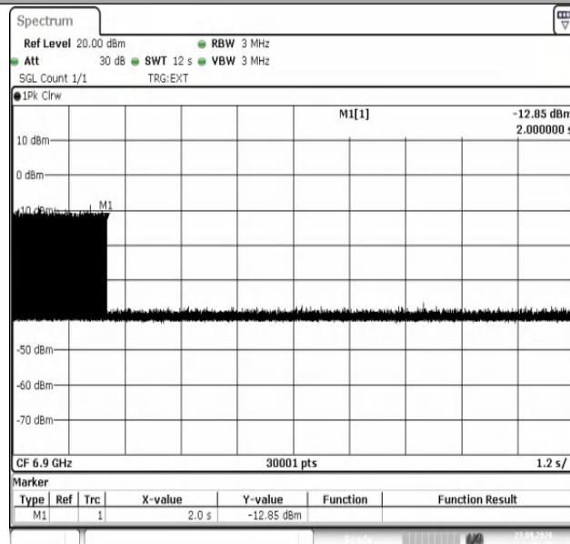
11AX80SISO-Ant1-6865-6900-5-PASS
