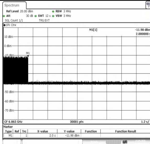
11AX80SISO-Ant1-6865-6865-9-PASS
